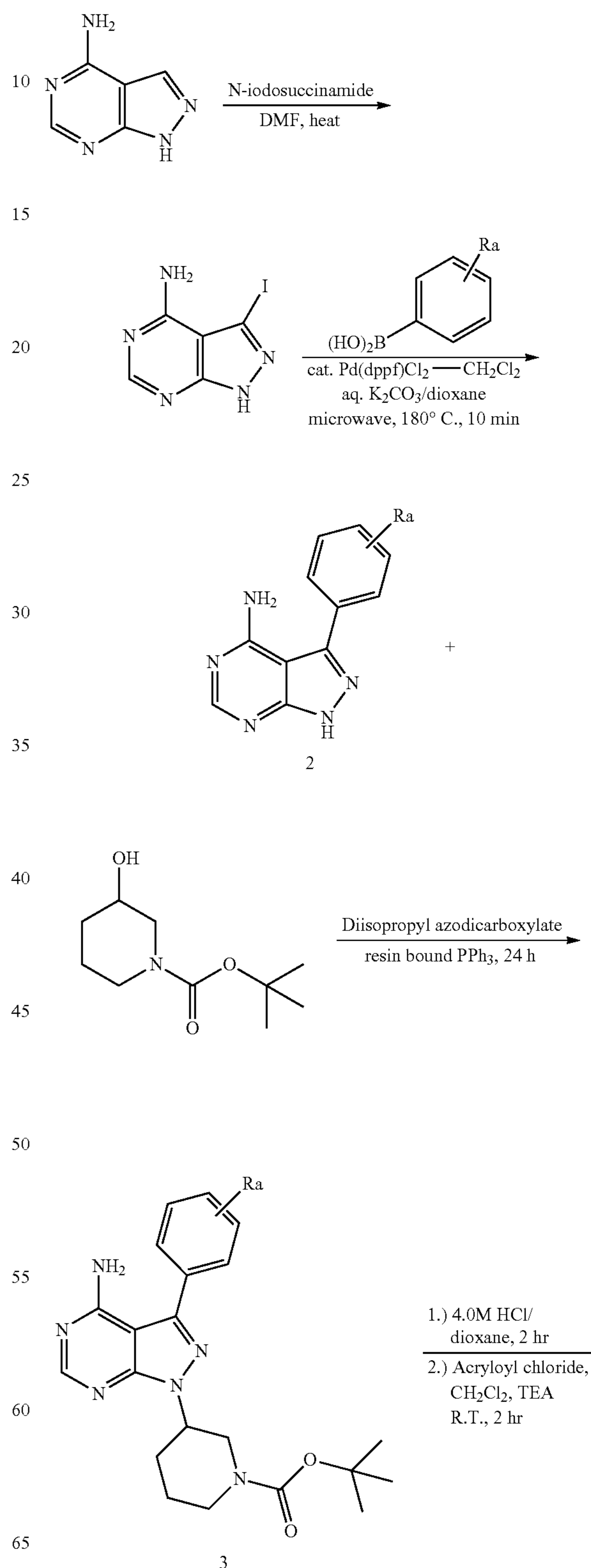
Scheme I.
