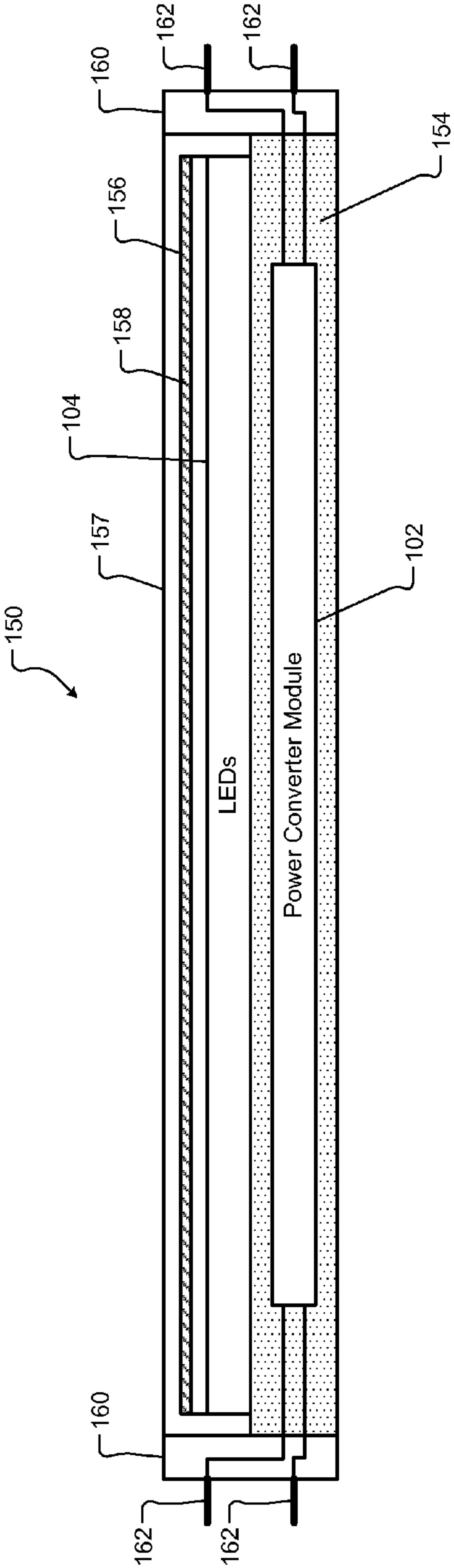
FIG. 5A
