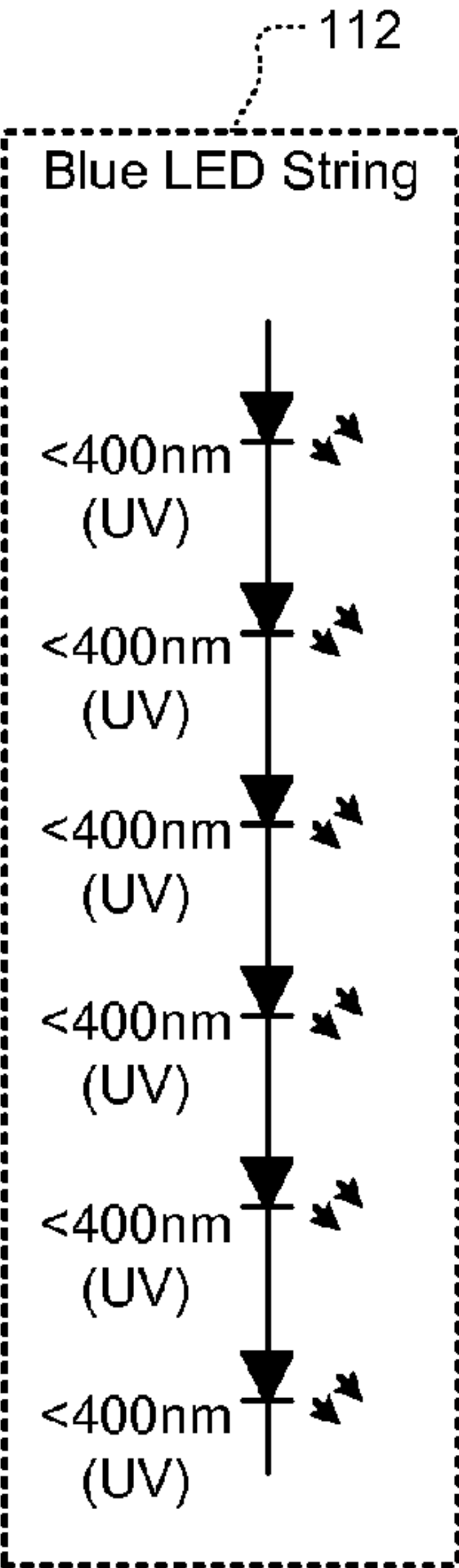
FIG. 12A
