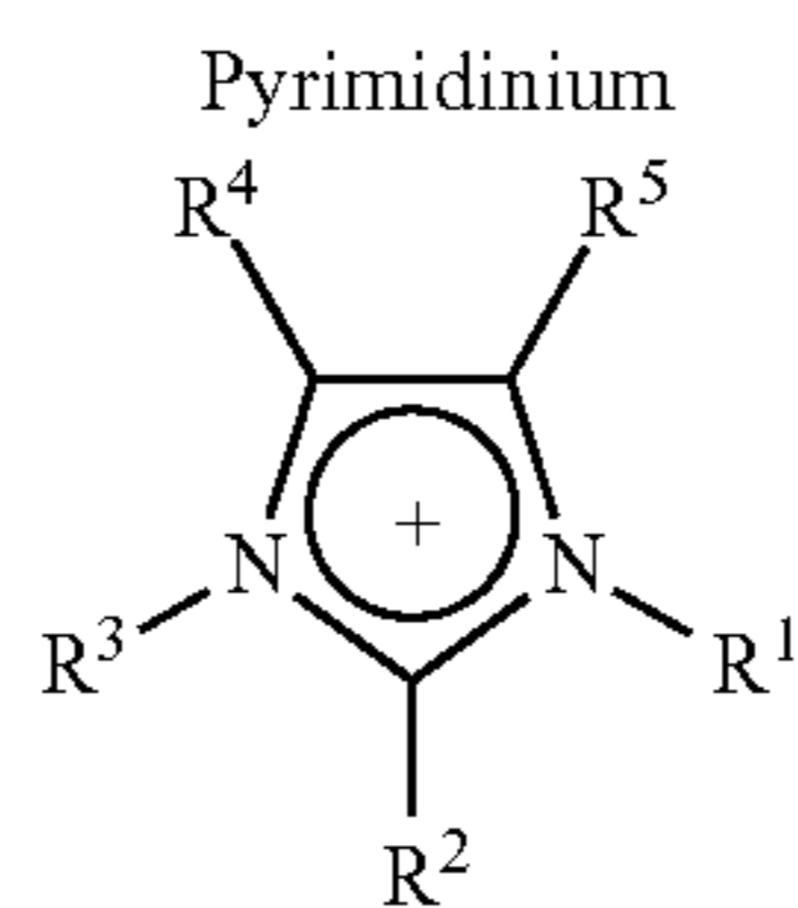
Imidazolium
