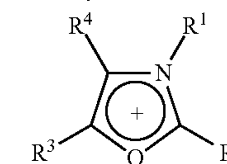
Oxazolium
