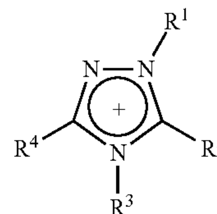
Triazolium
