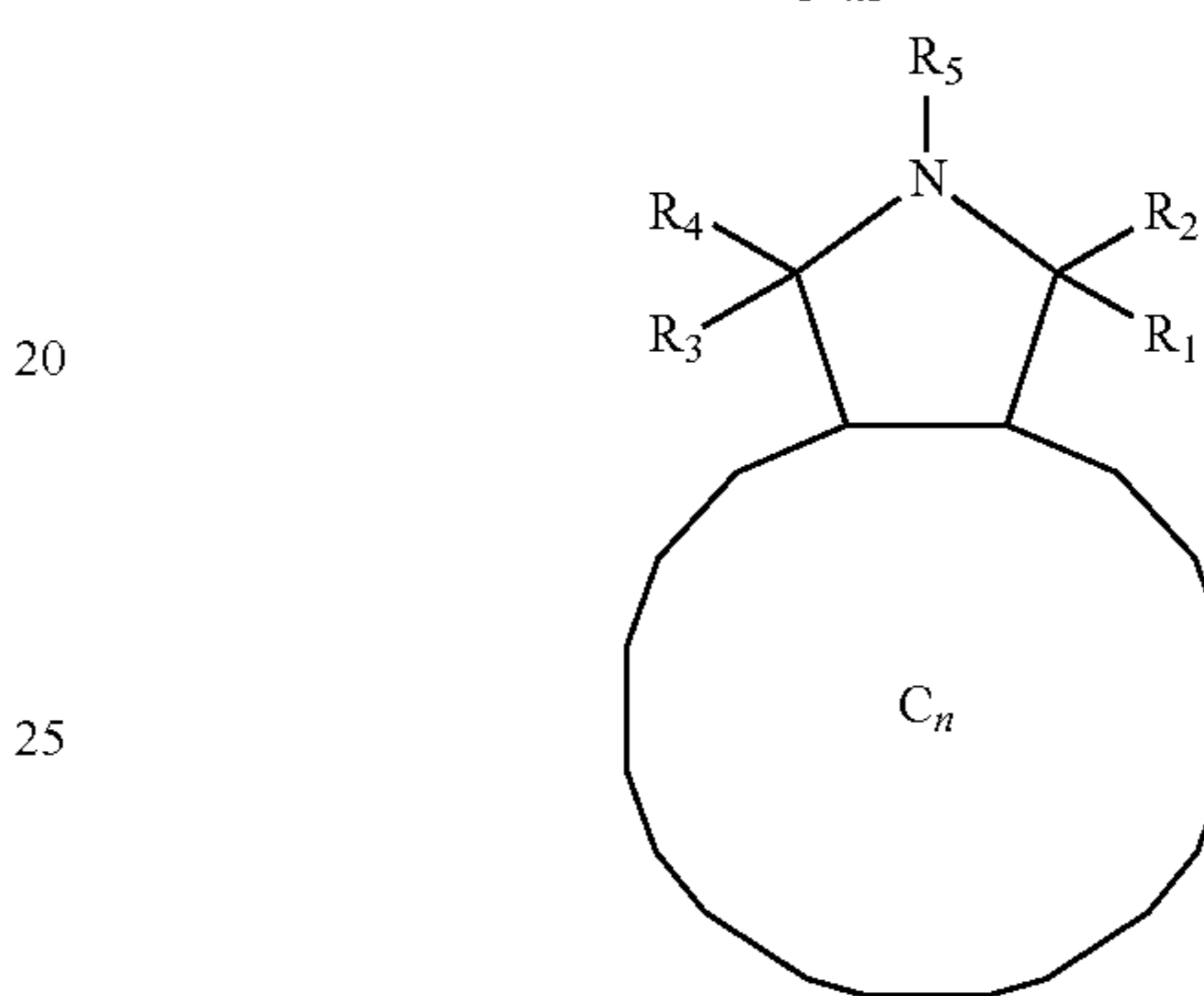
[ C_n ]Prato
