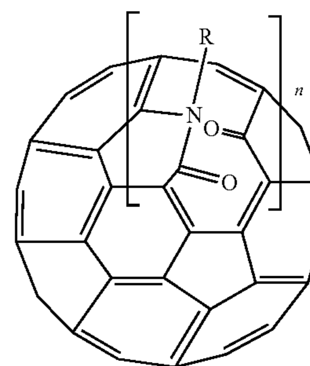
Ketolactam
