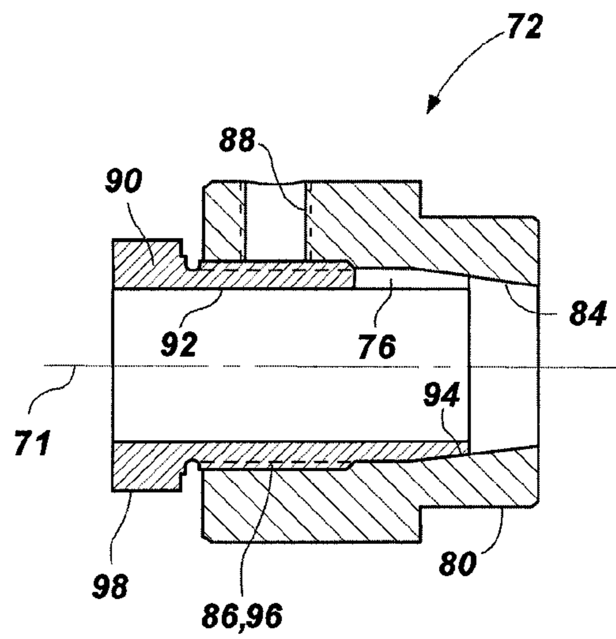
Section A-A
