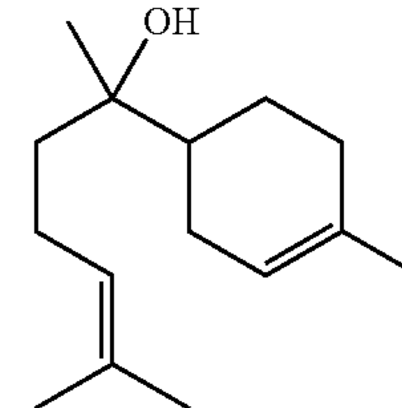
nerolidol (CAS #7212-44-4)
