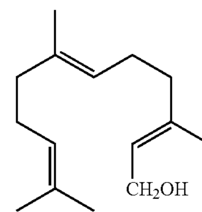
farnesol (CAS #4602-84-0)
