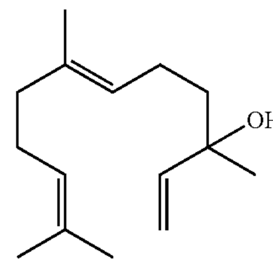
farnesol (CAS #4602-84-0)
