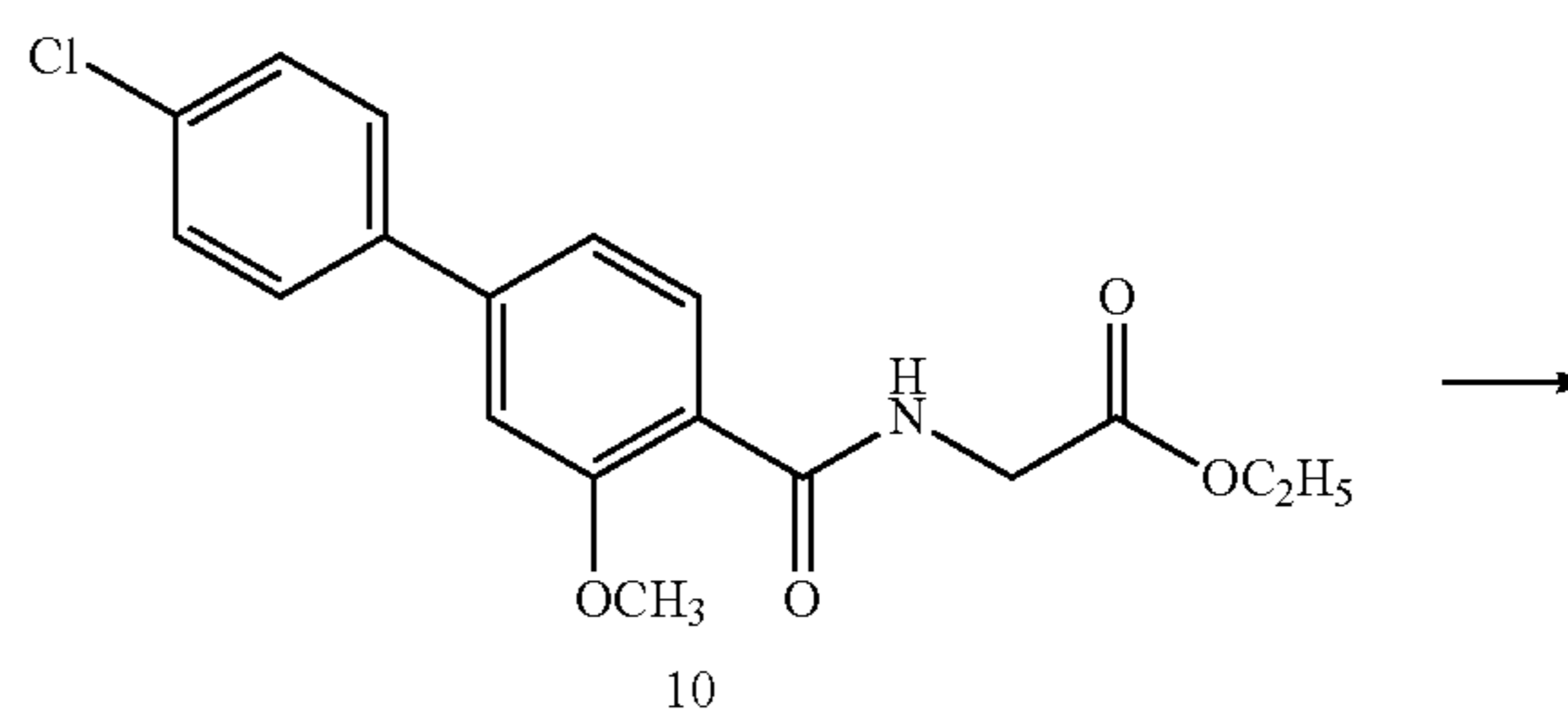
Scheme VI
