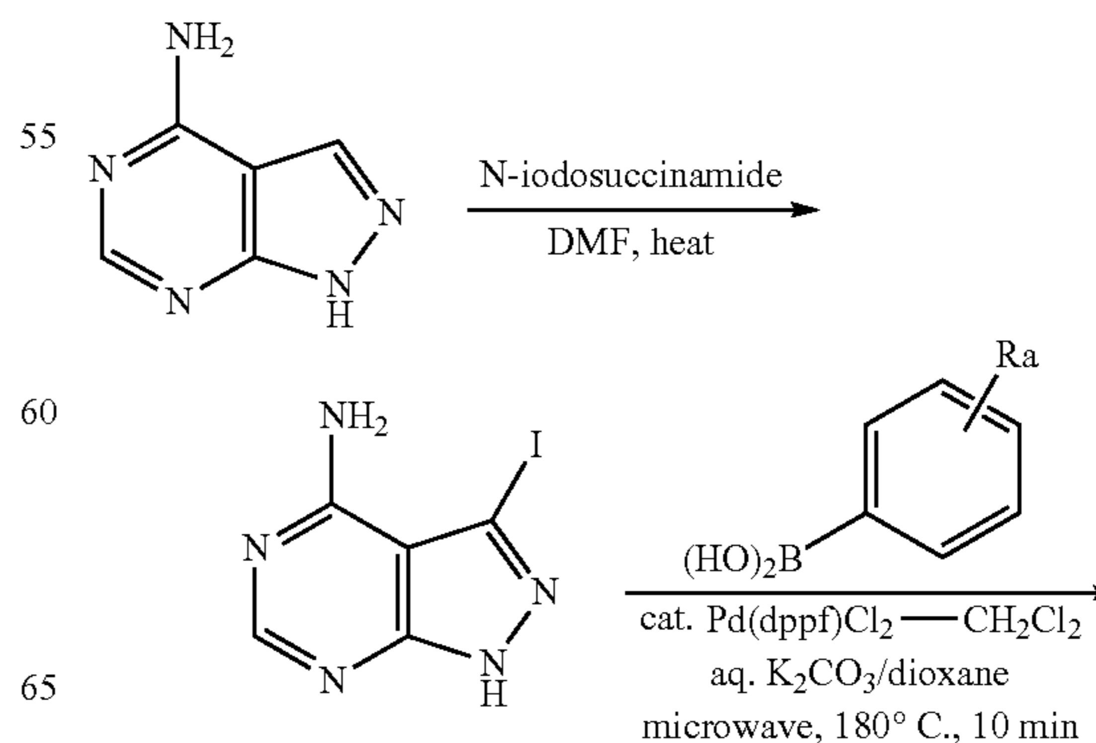
Scheme I.
