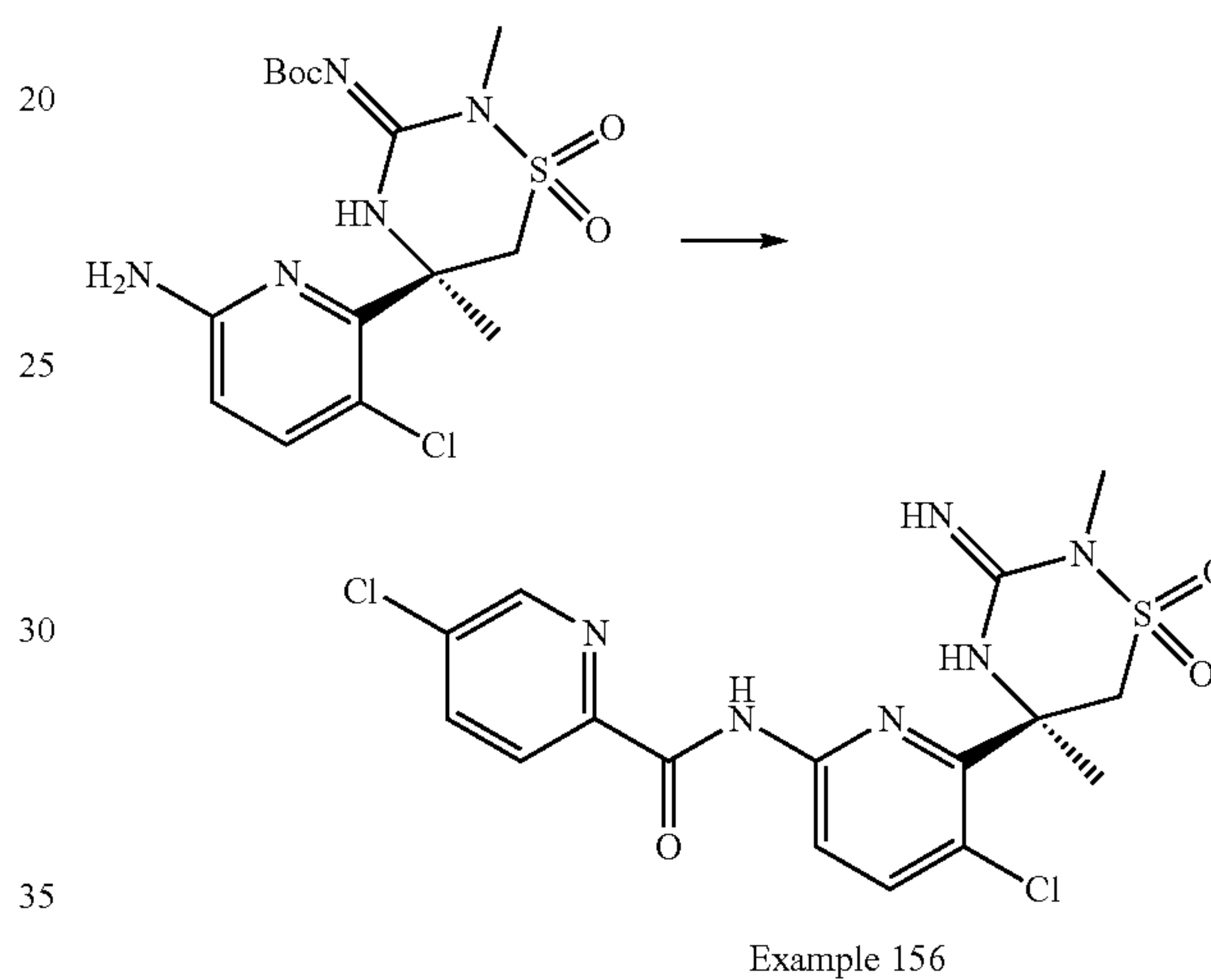
Scheme 37:
