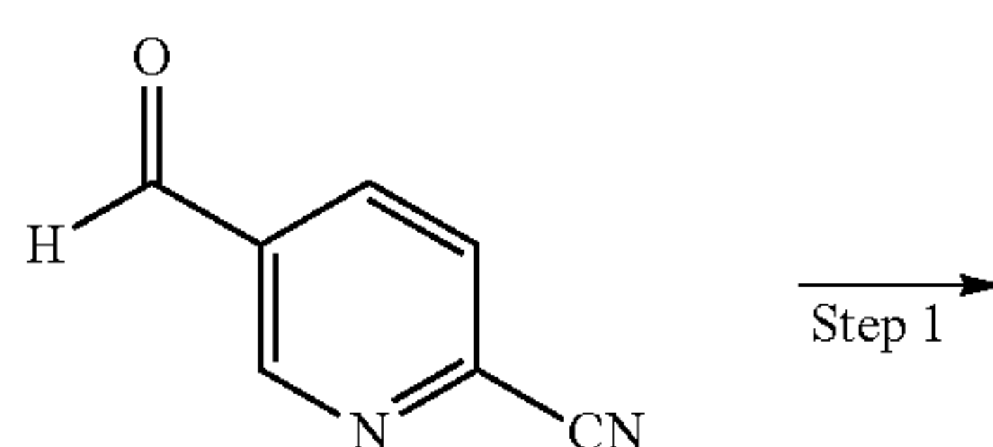
Scheme 11ab:
