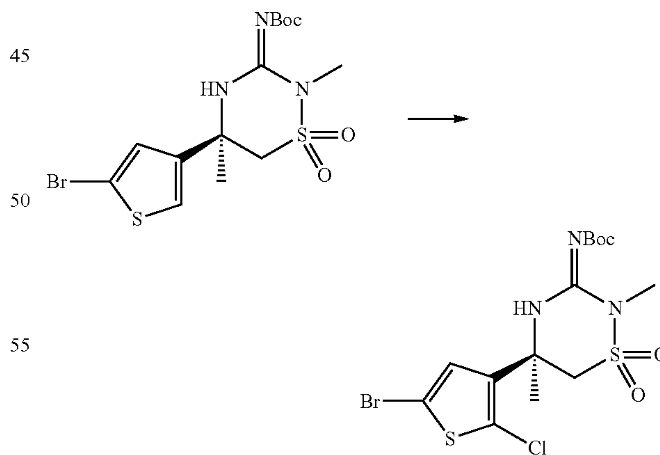
Scheme 9a:
