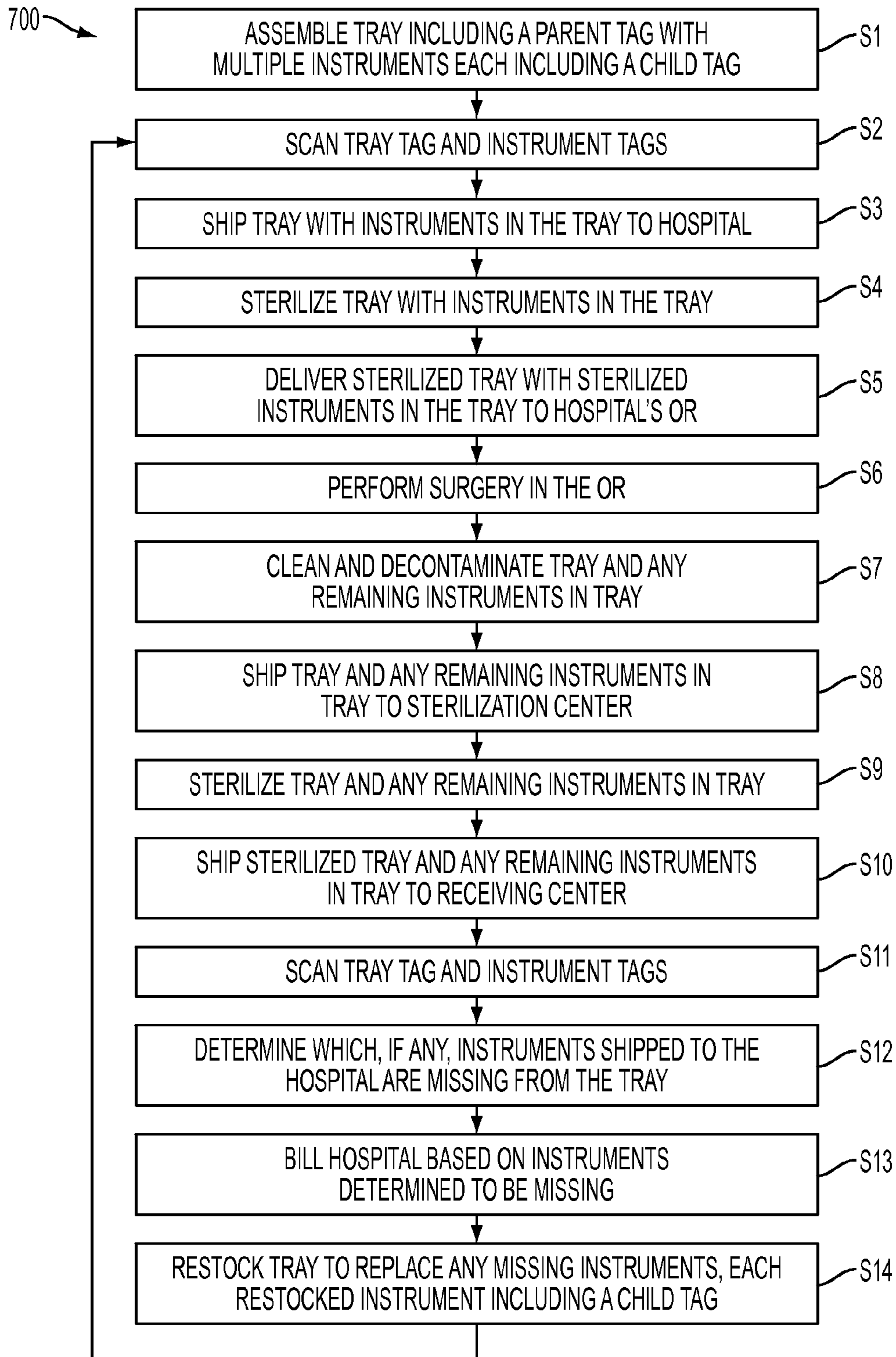
FIG. 17
