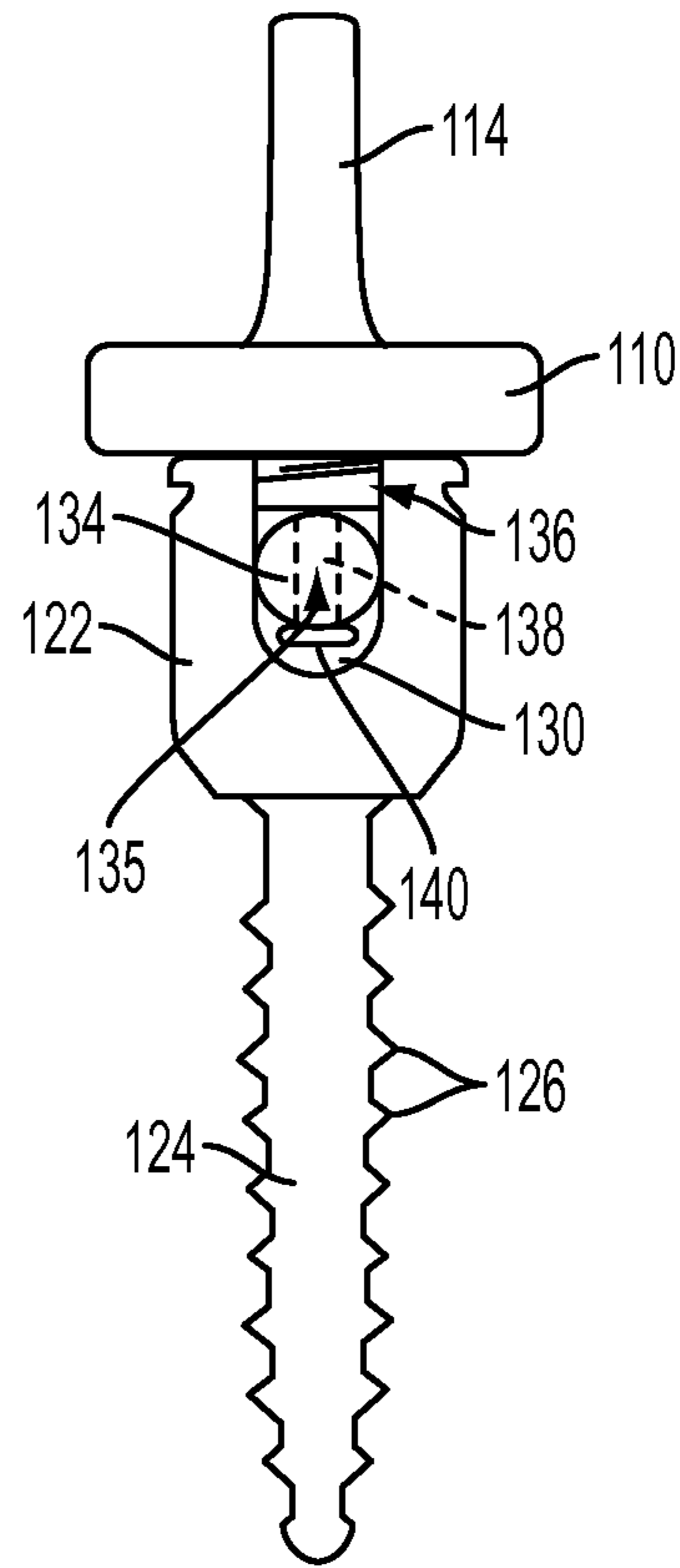
FIG. 6
