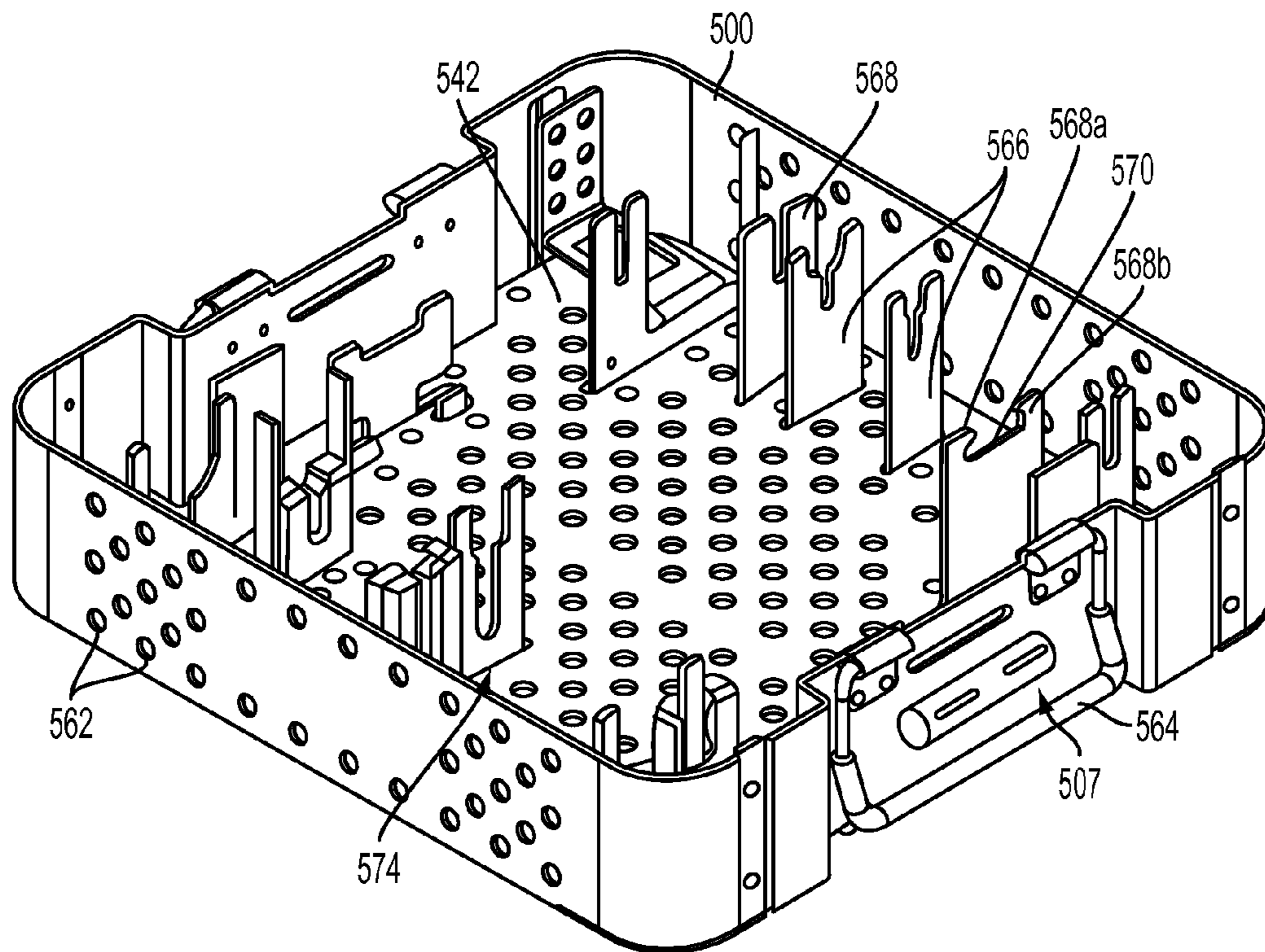
FIG. 15
