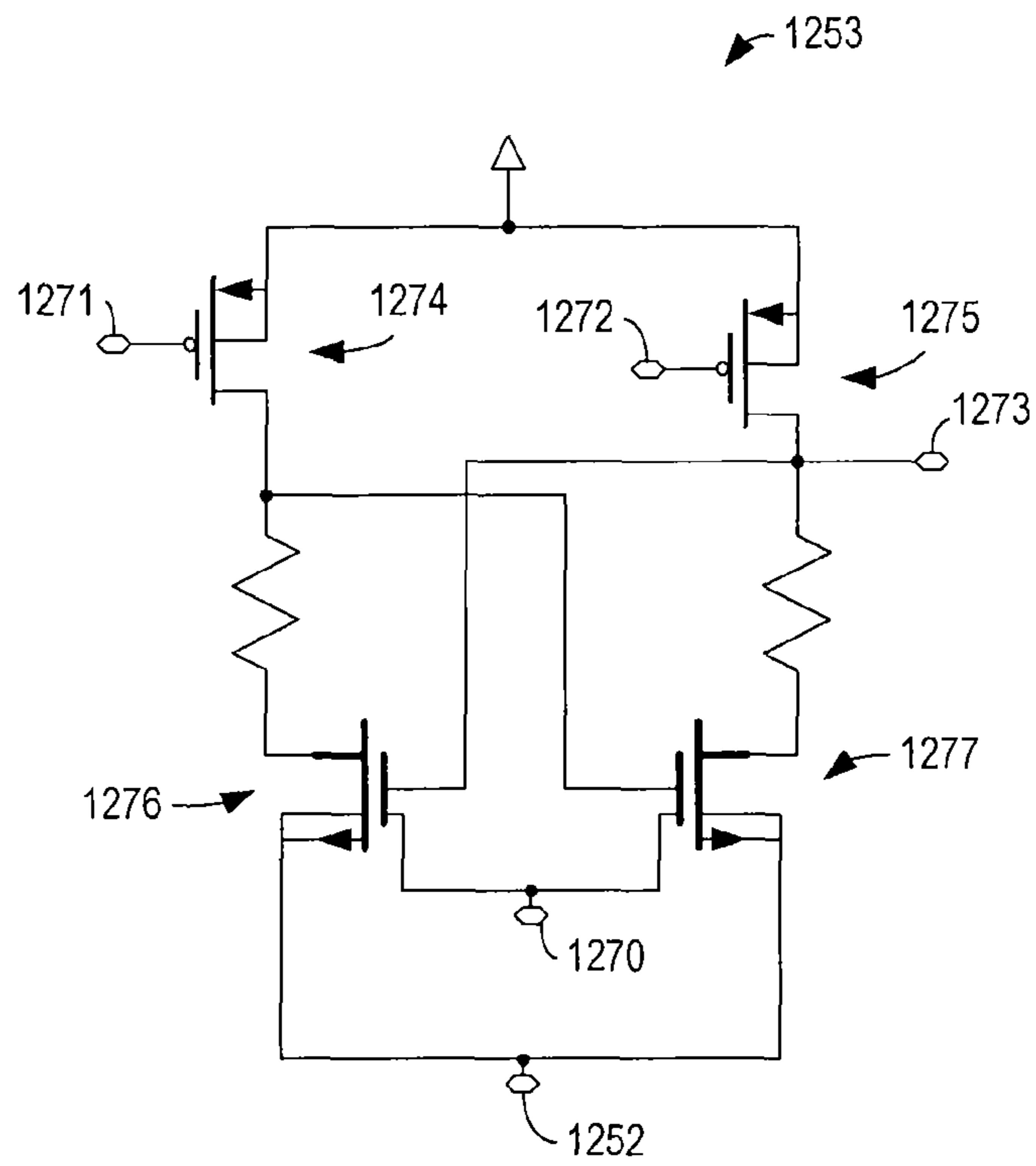
FIG. 12A
