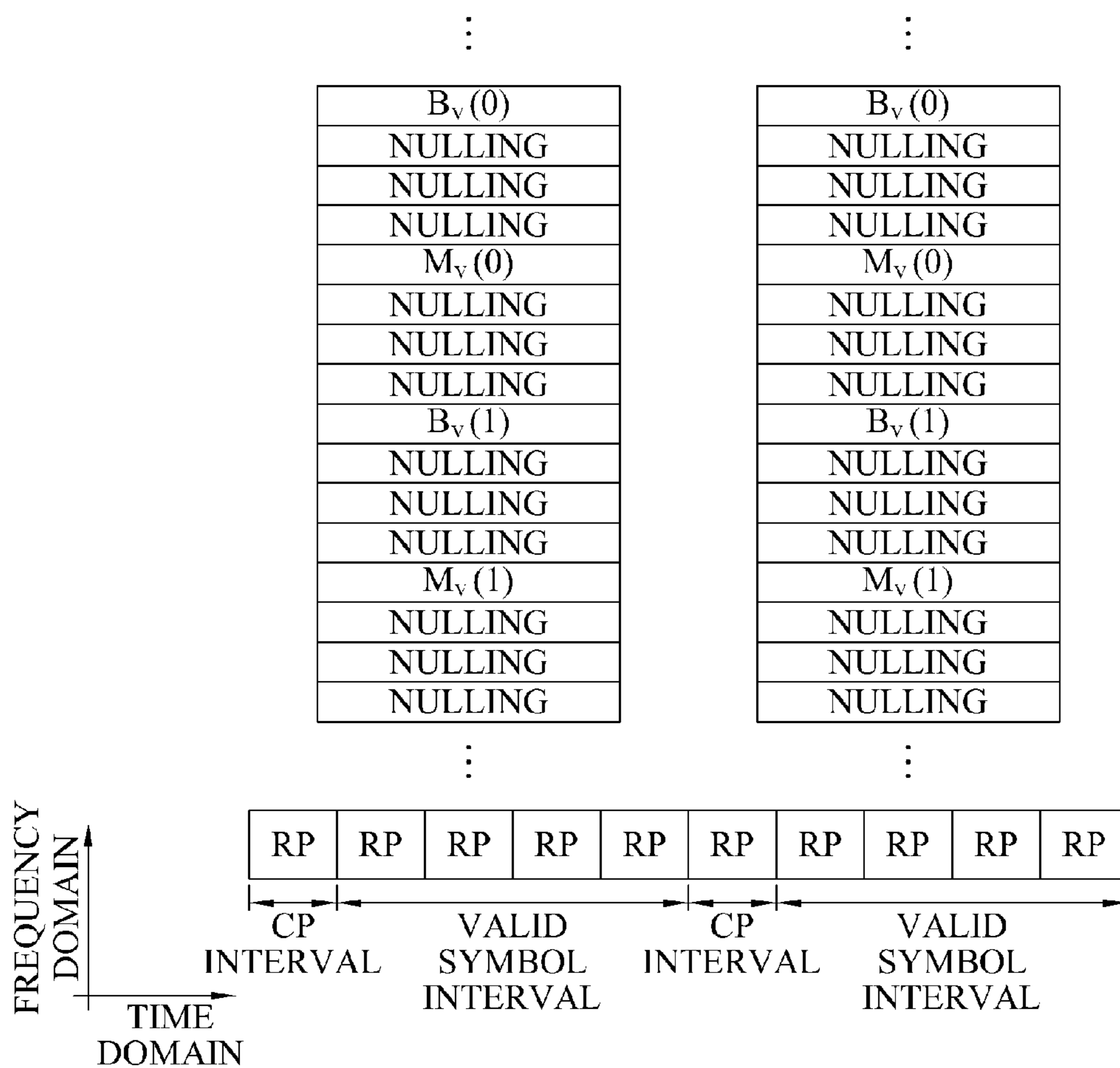
FIG. 17
