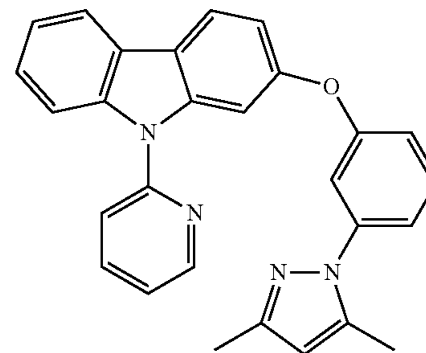
2-[3-(3,5-Dimethylpyrazol-1-yl)-phenoxy]-9-pyridin-2-ylcarbazole
