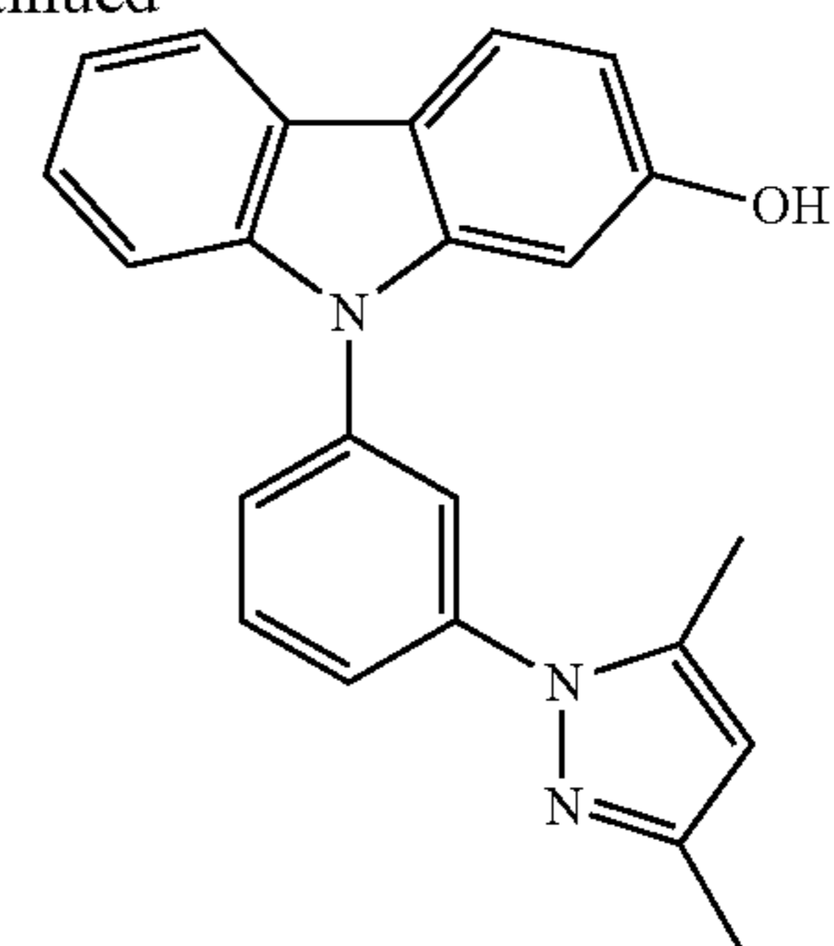
N-(3,5-Dimethylpyrazolyl)phenyl)-2-hydroxycarbazole
