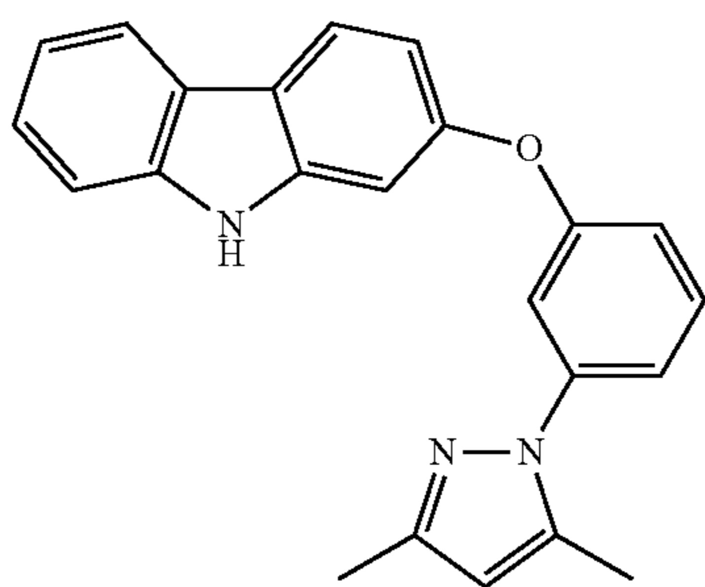
2-[3-(3,5-Dimethylpyrazol-1-yl)-phenoxy]-carbazole
