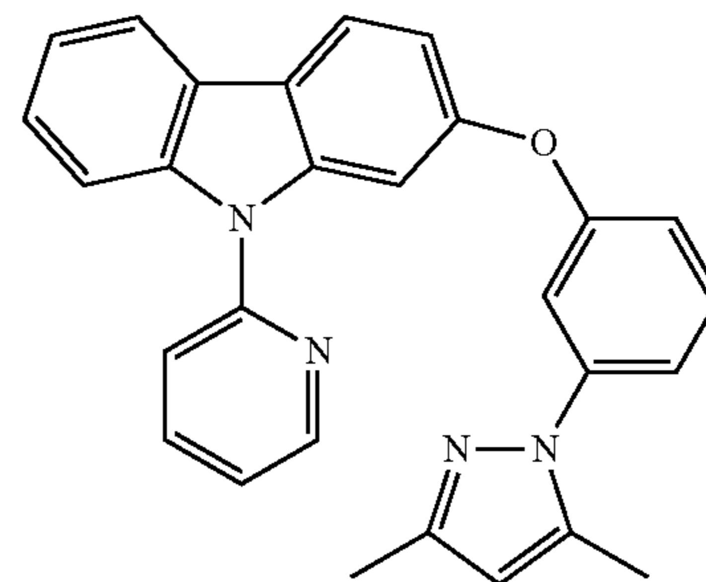
2-[3-(3,5-Dimethylpyrazol-1-yl)-phenoxy]-9-pyridin-2-ylcarbazole
