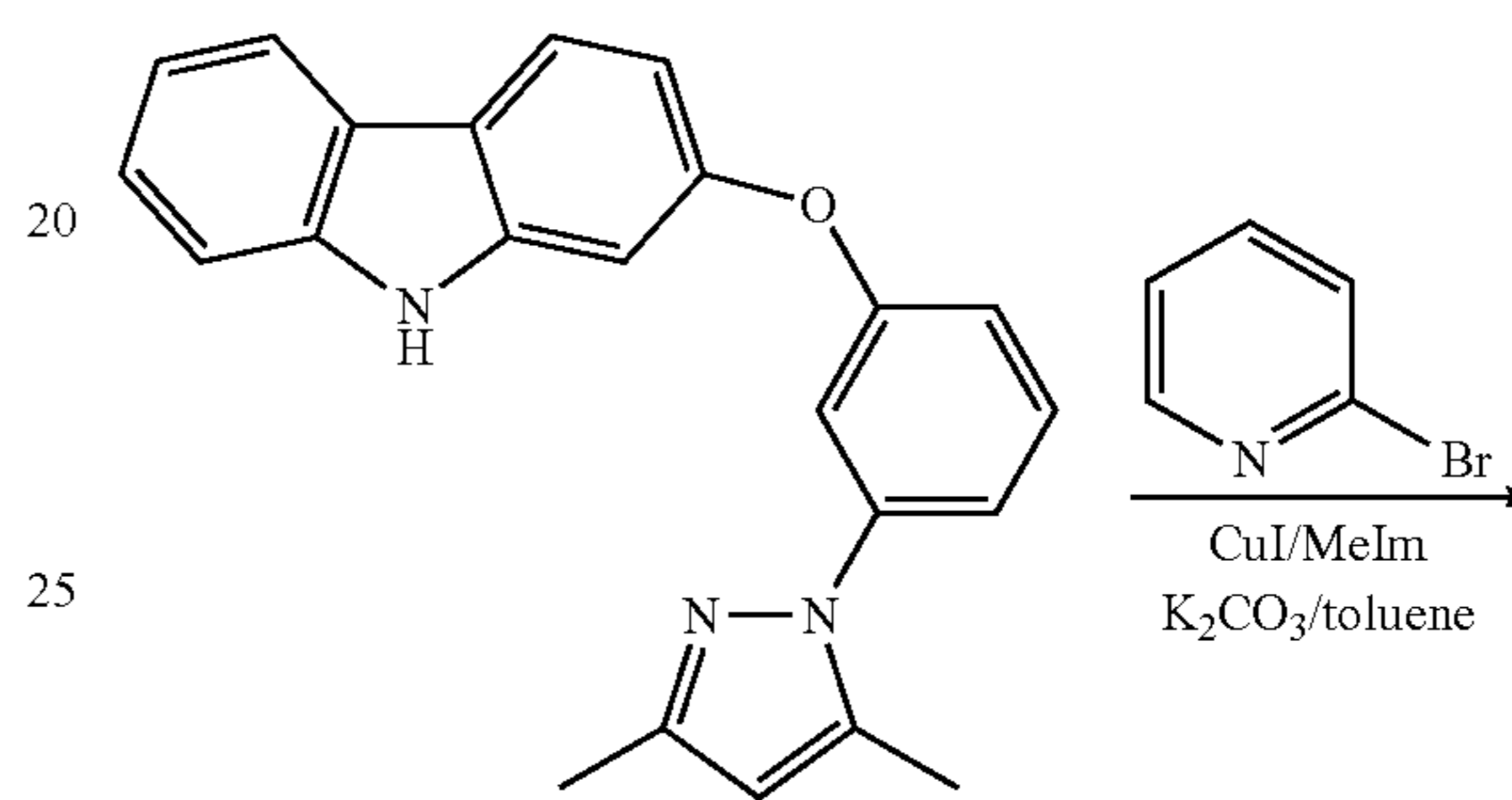
2-[3-(3,5-Dimethylpyrazol-1-yl)-phenoxy]-carbazole
