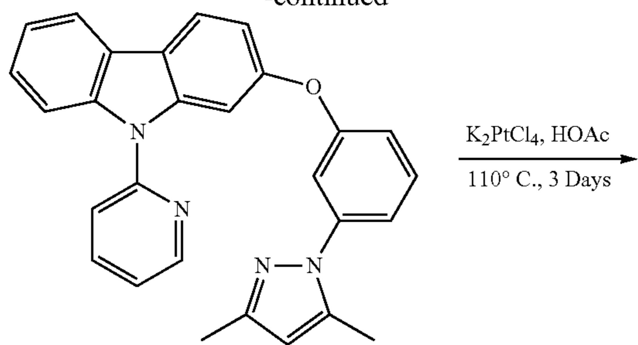
2-[3-(3,5-Dimethylpyrazol-1-yl)- phenoxy]-9-pyridin-2-ylcarbazole
