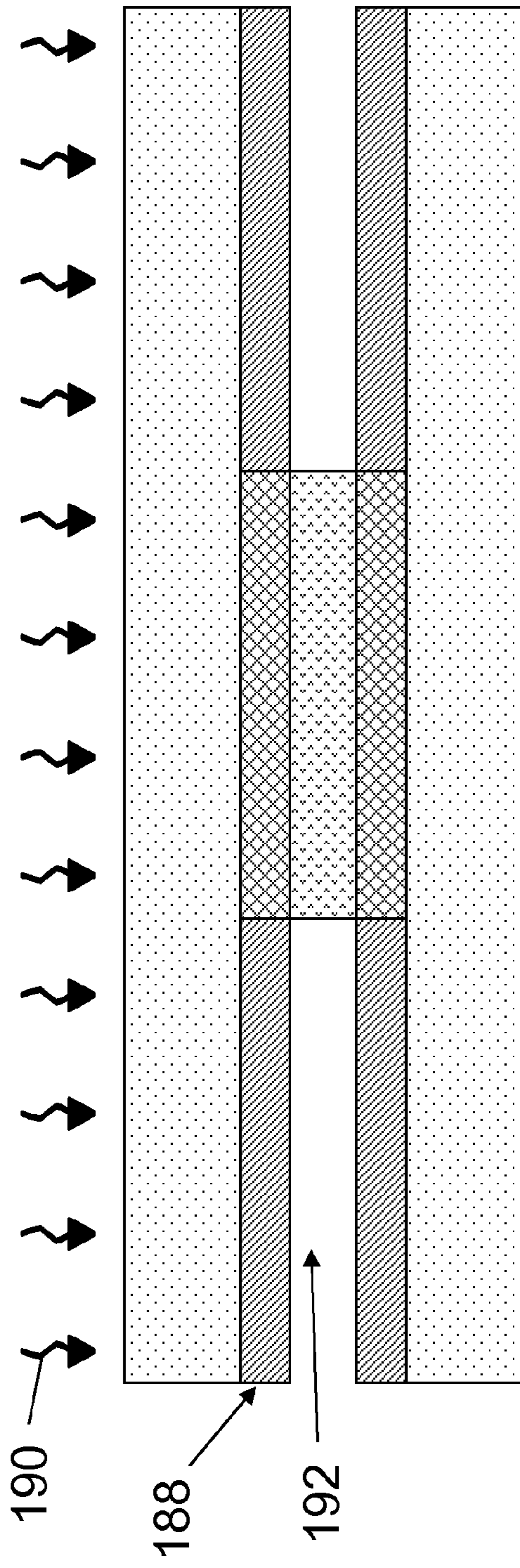
FIG. 16A
