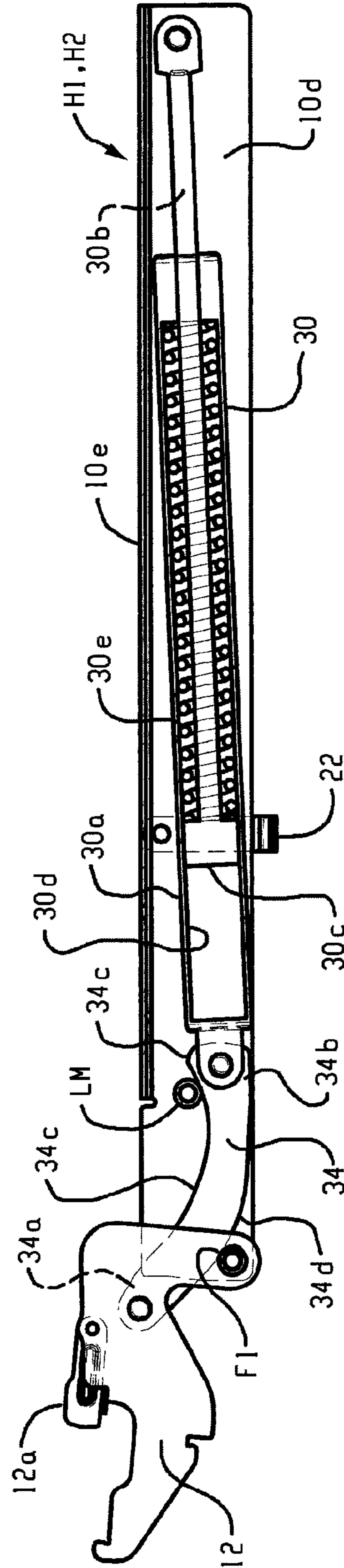
Fig. 7
