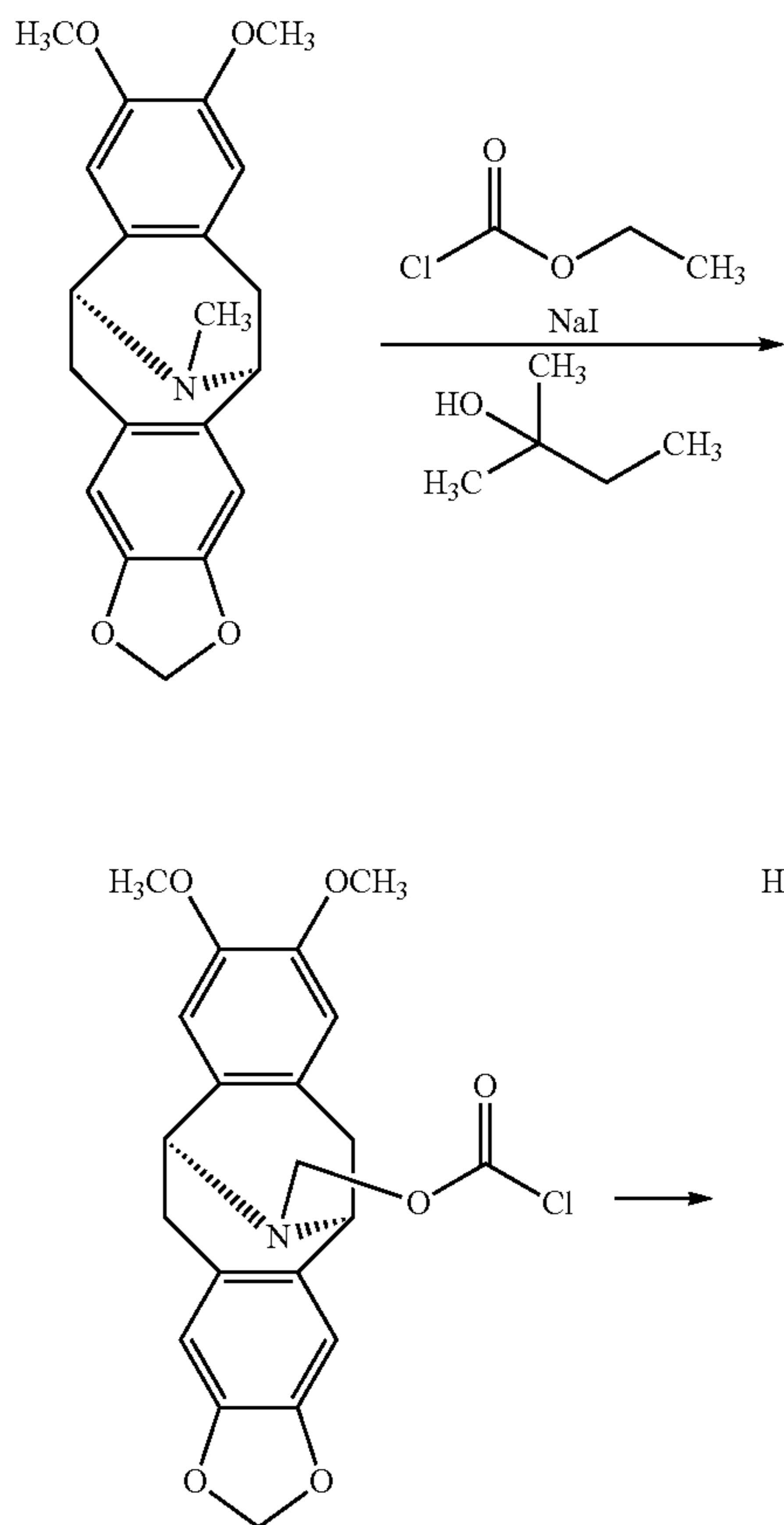
Scheme 17: (+)-Eschscholtzidine
