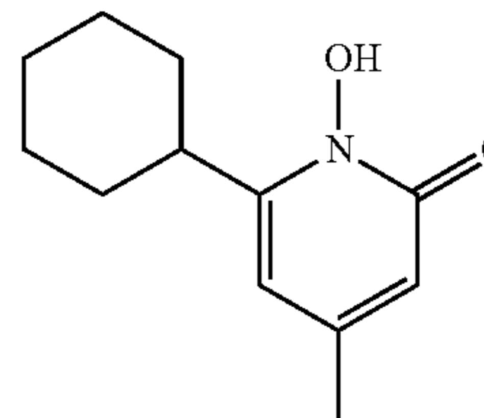
ciclopirox (II-b) (CAS 29342-05-0)
