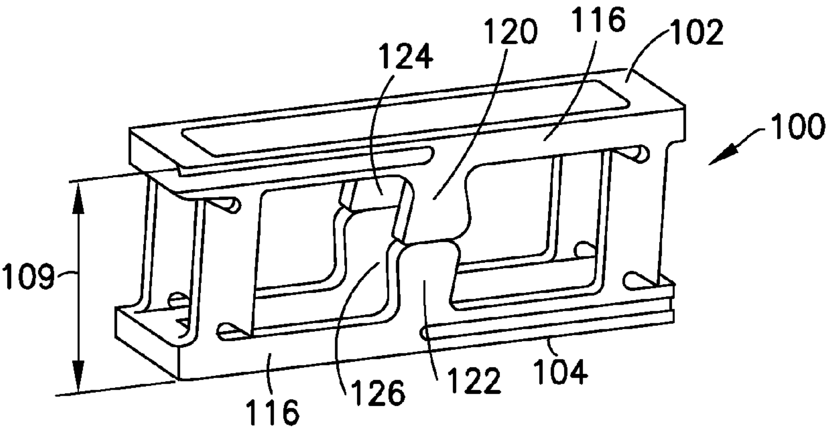
FIG. 1C
