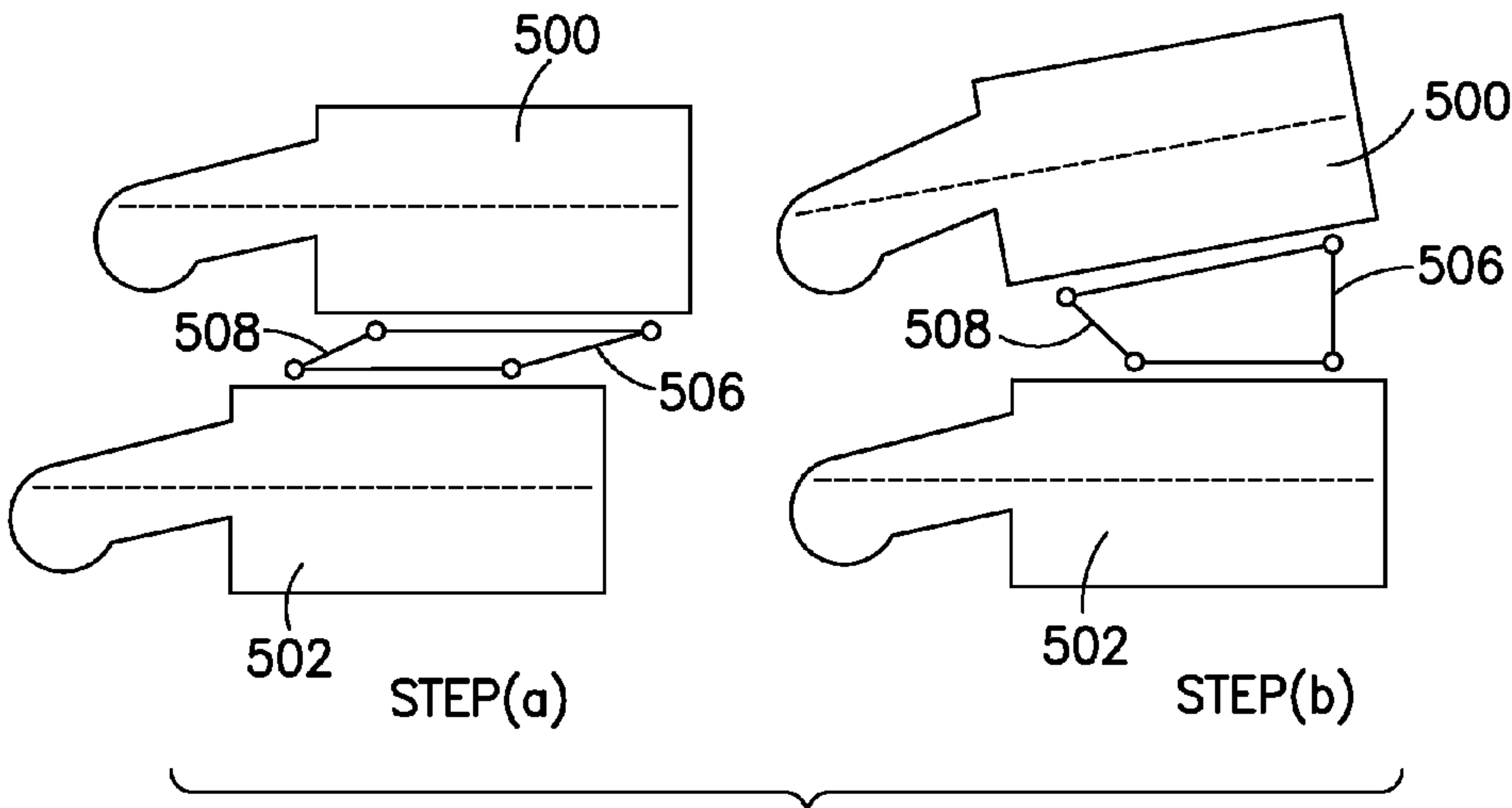
FIG.14
