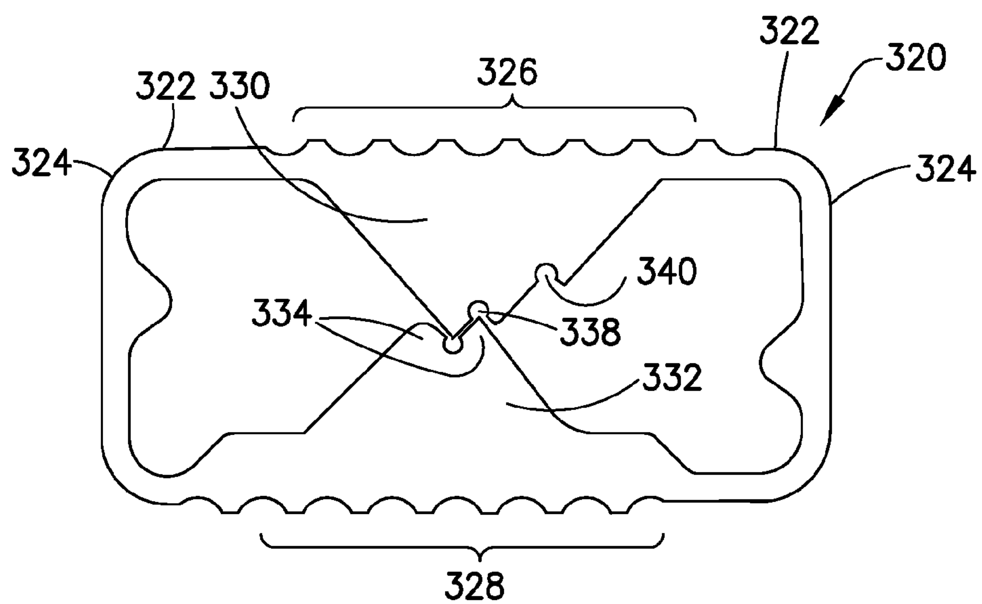
FIG. 10C
