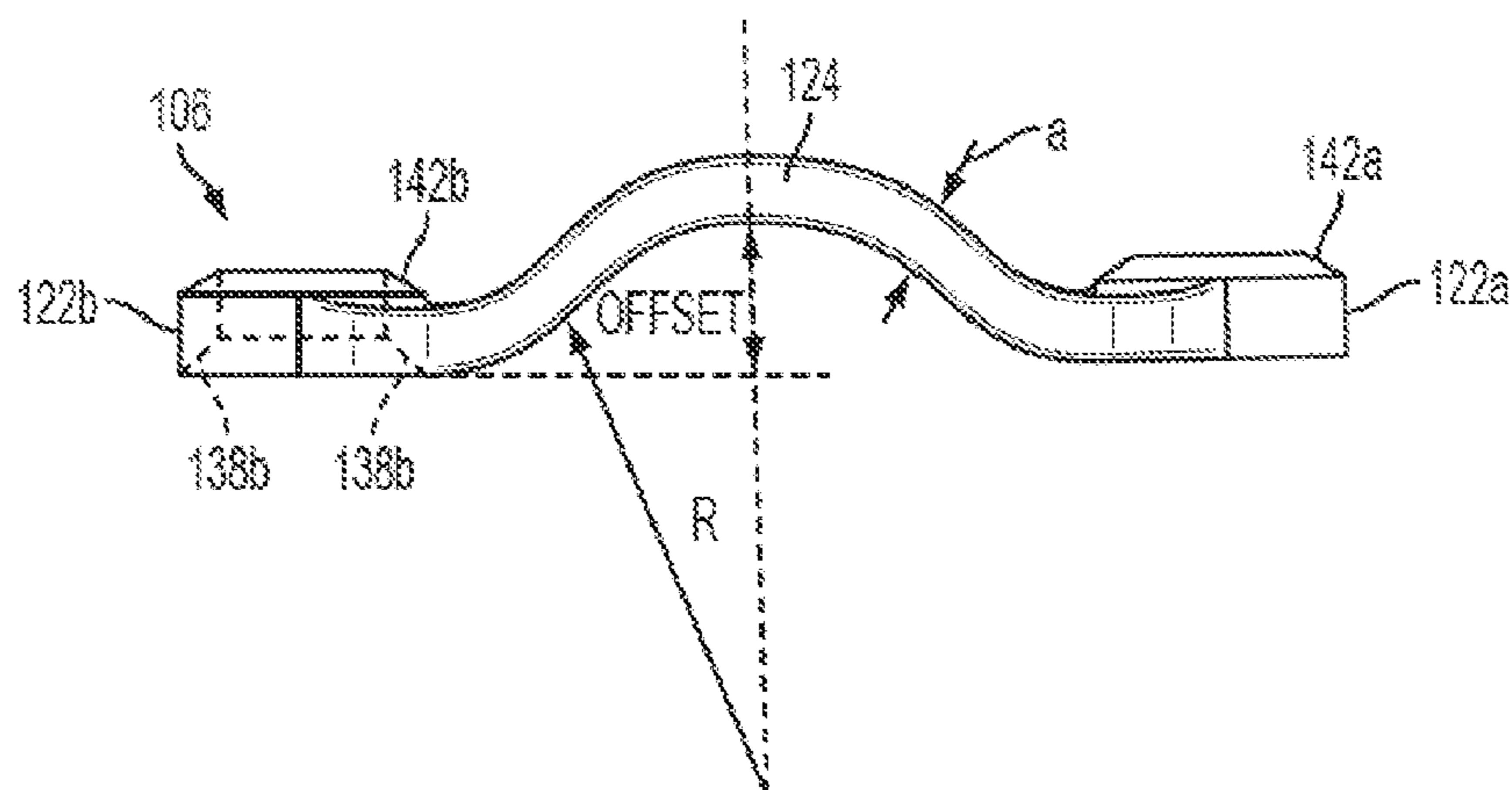
FIG. 2C
