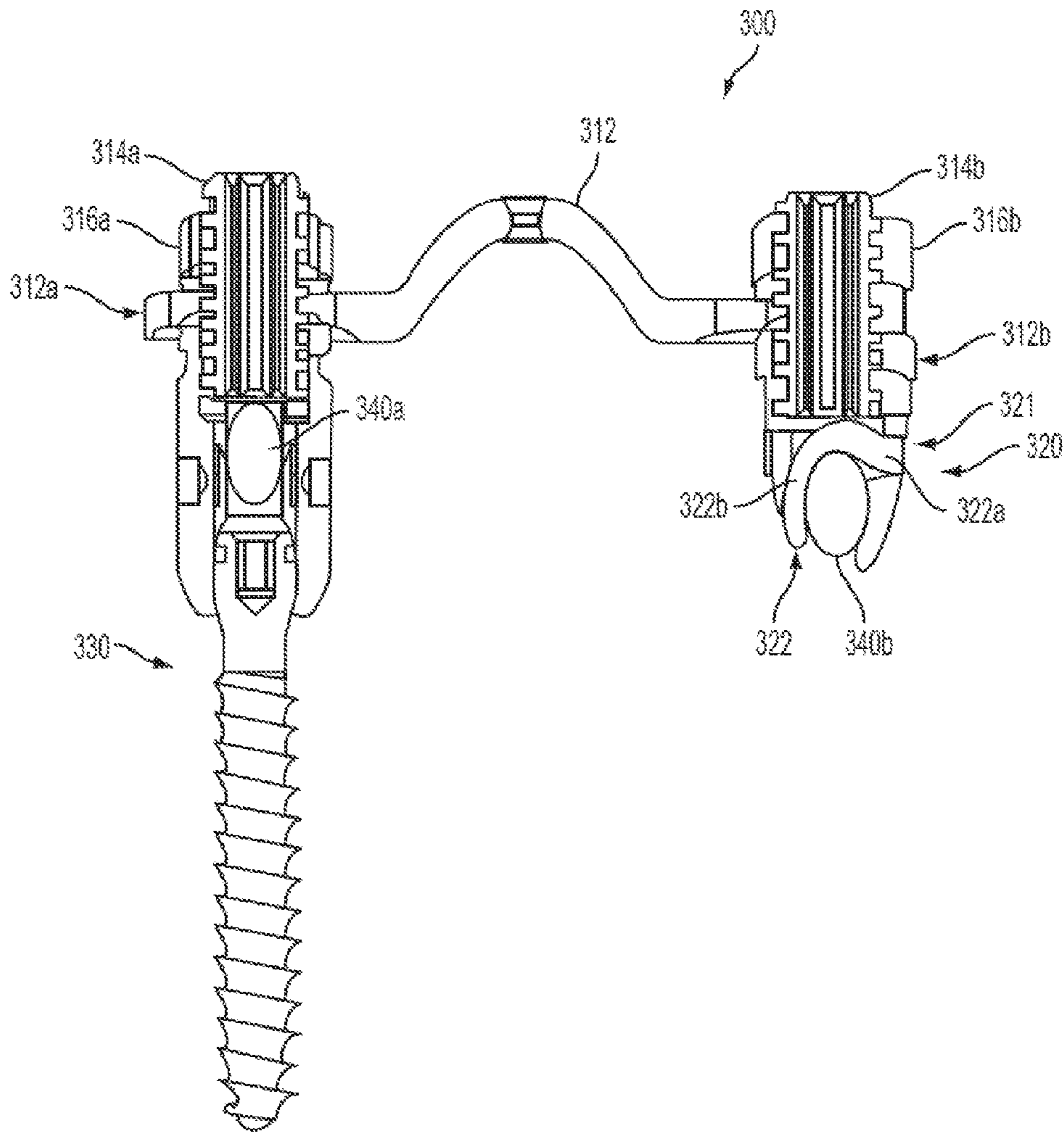
FIG. 19A
