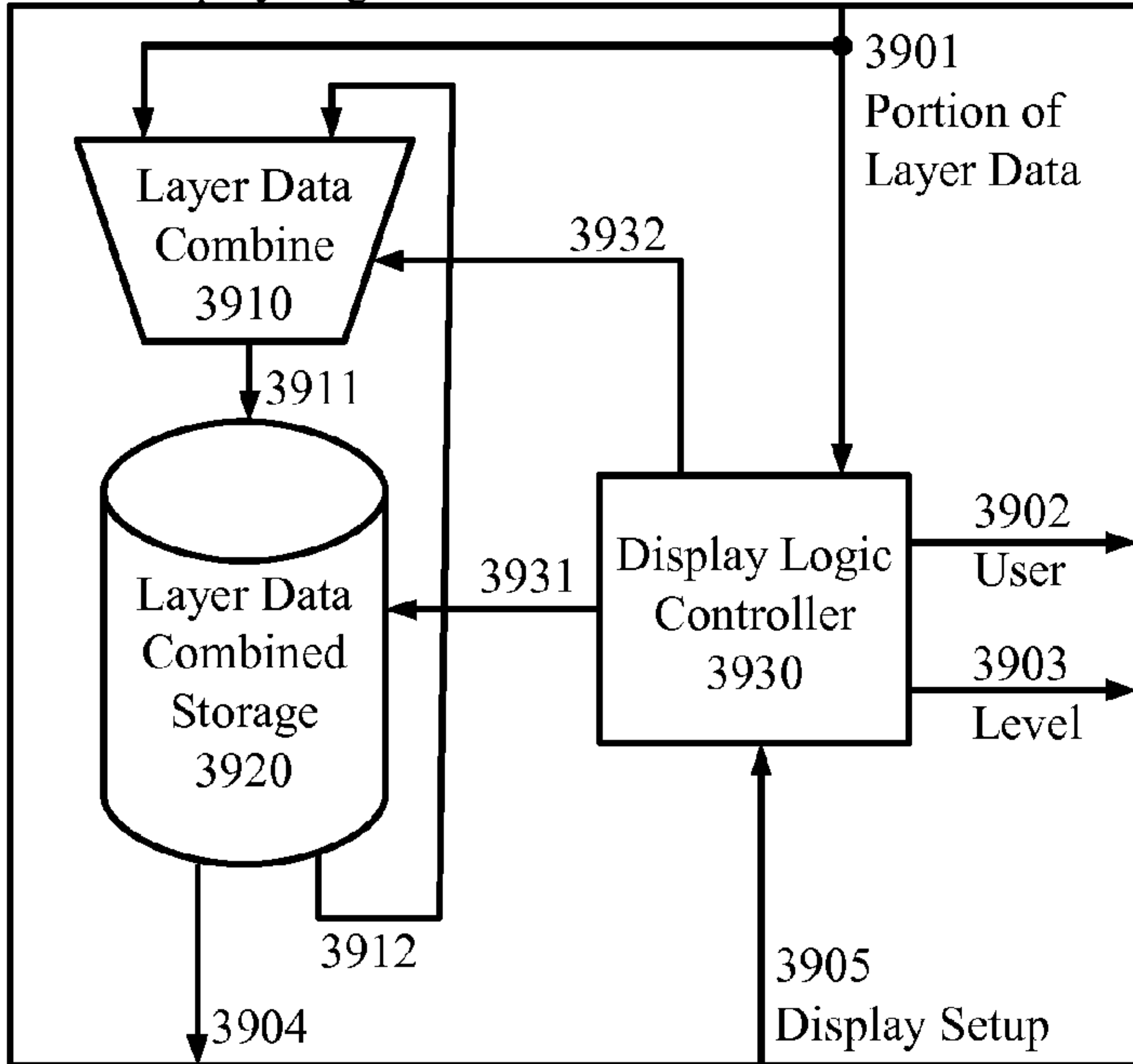
3900 Display Logic
