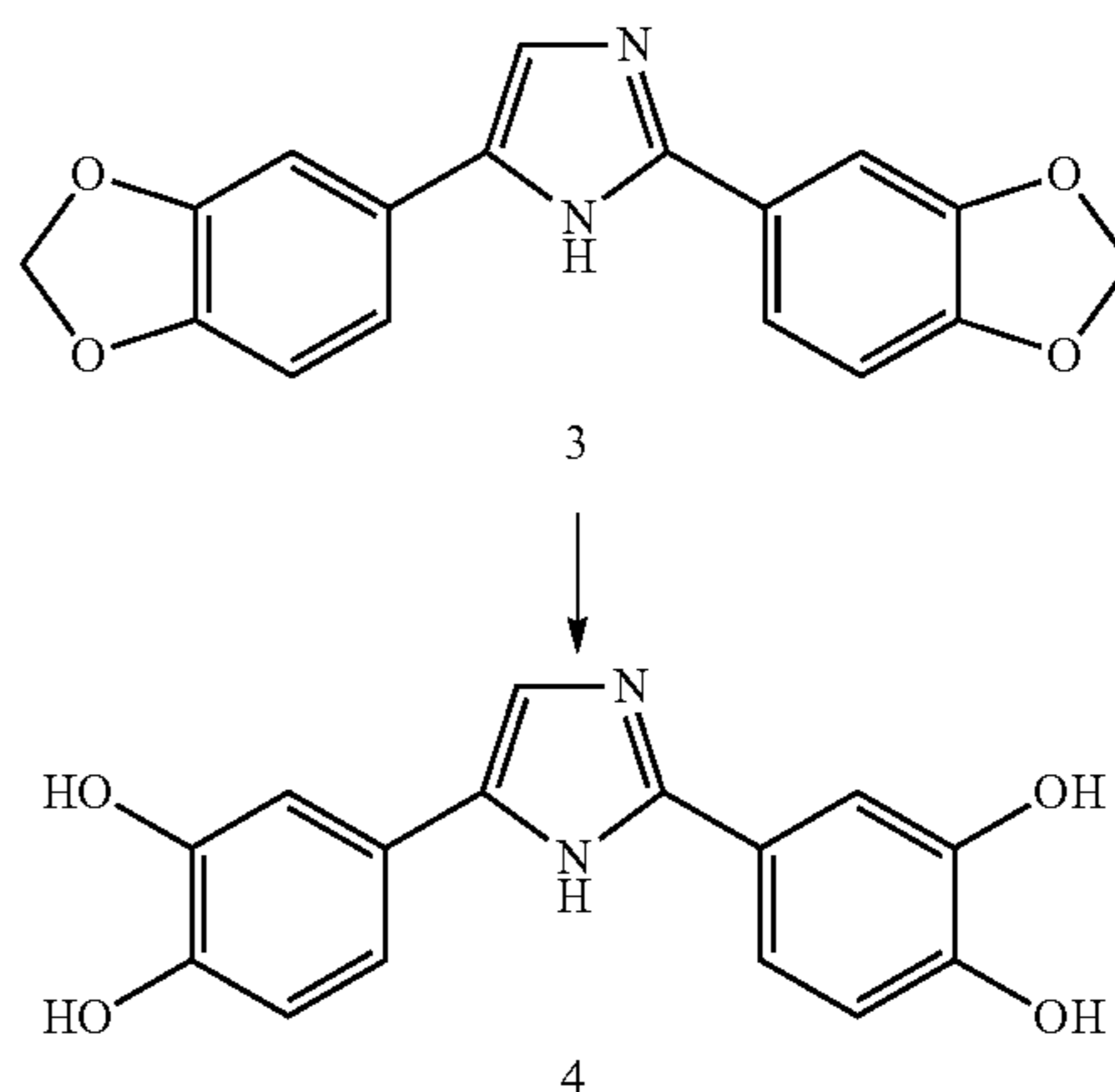
2,4 bis (3,4 dihydroxyphenyl) imidazole
