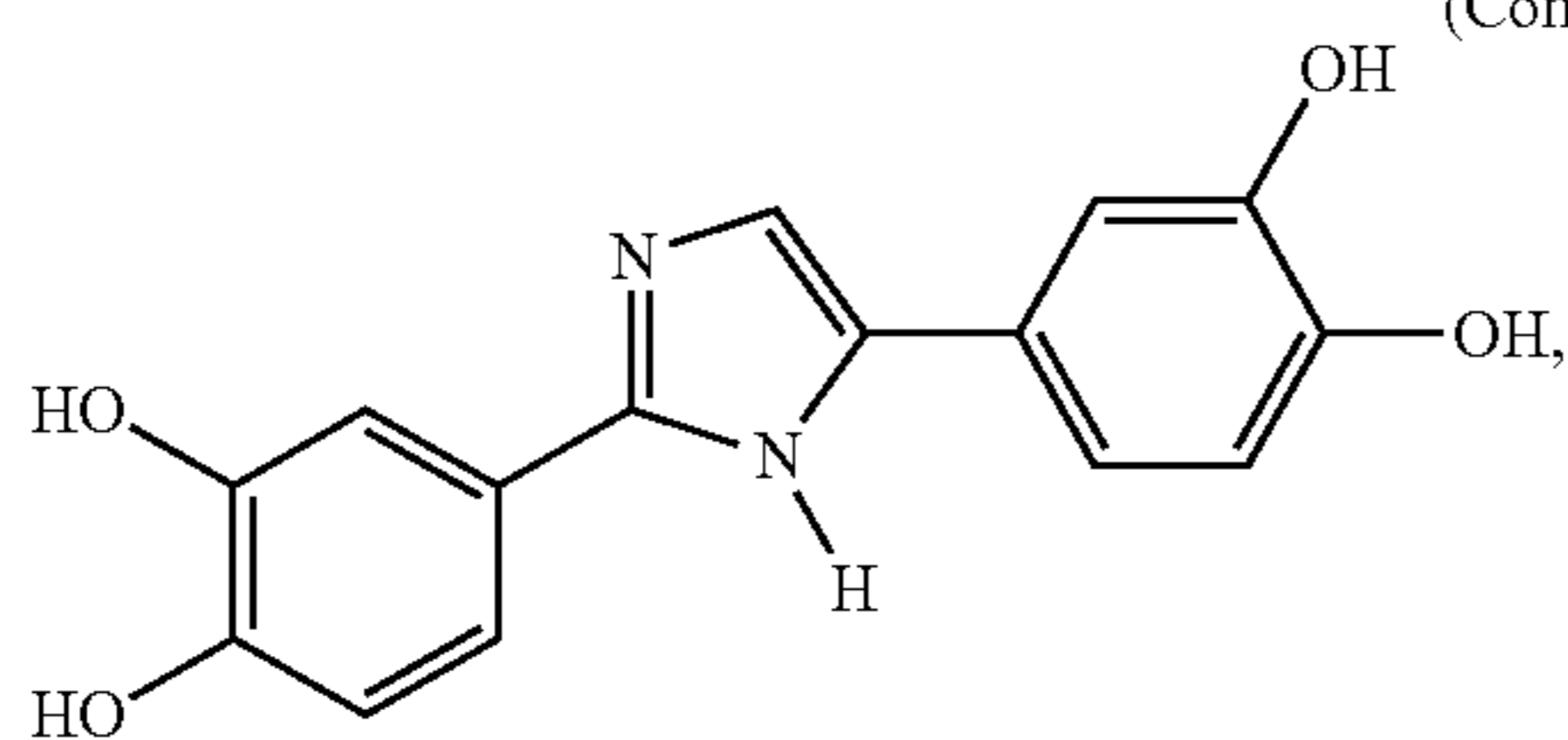
2,4 bis (3,4 dihydroxyphenyl) imidazole
