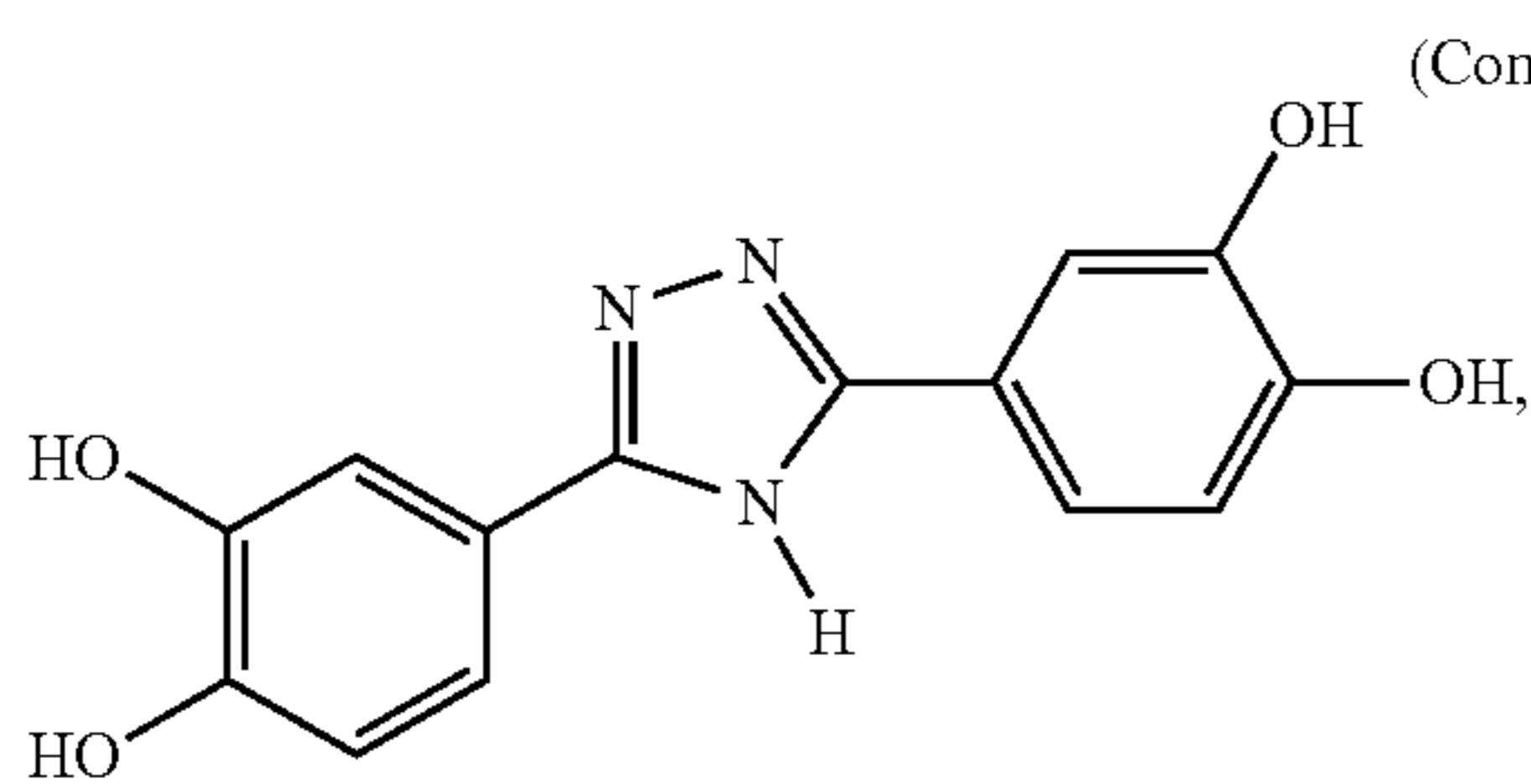
3,5, bis (3,4 dihydroxyphenyl) 1,2,4, triazole
