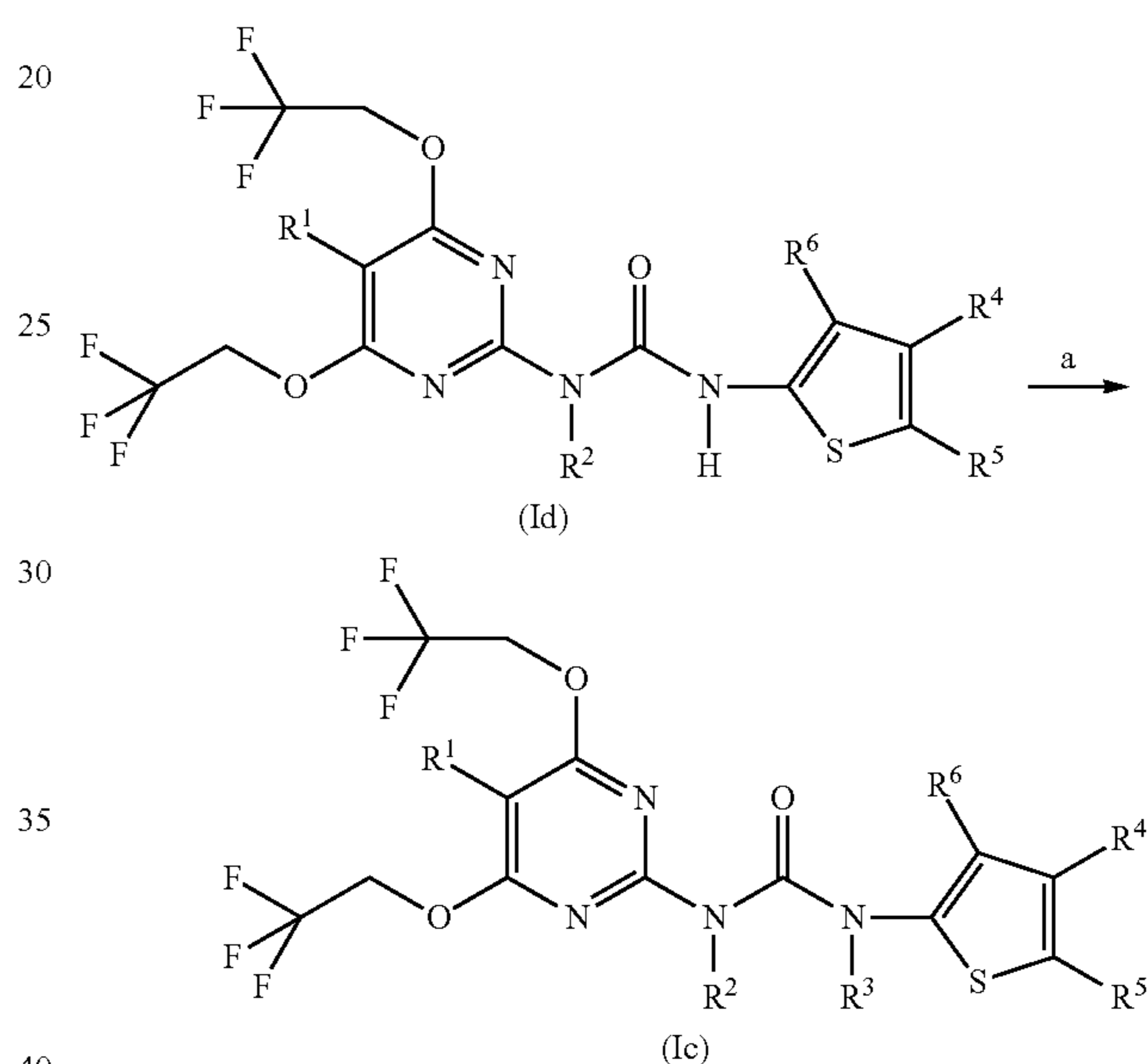
Scheme VI
