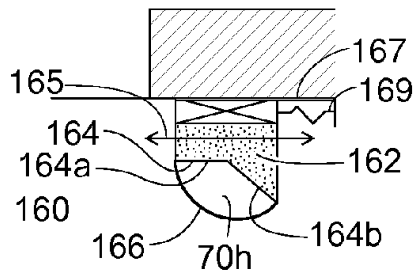
FIG. 40
