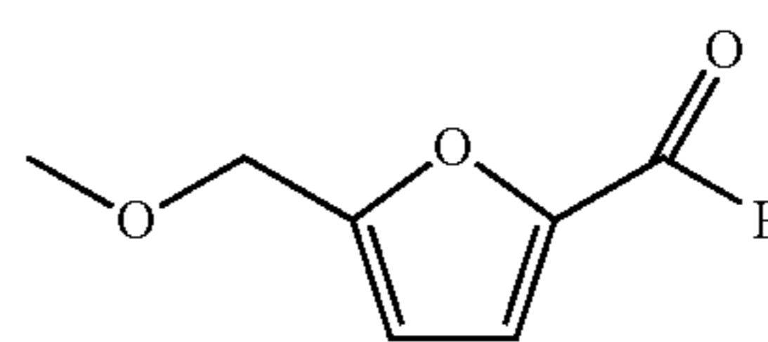
5-methoxymethylfurfural
