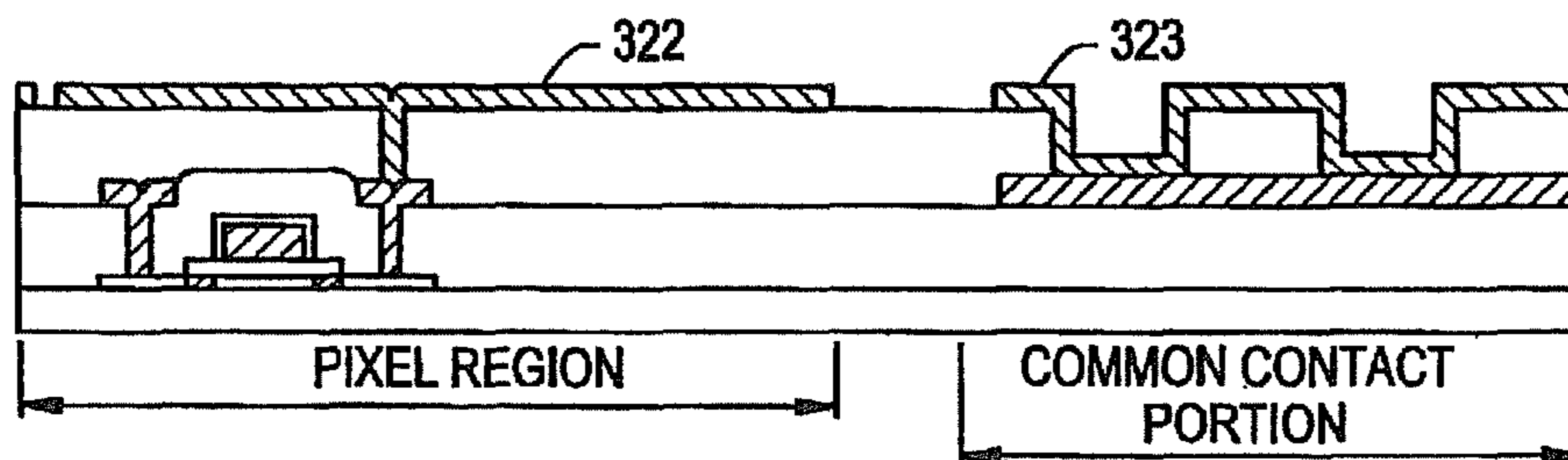
FIG.5G
