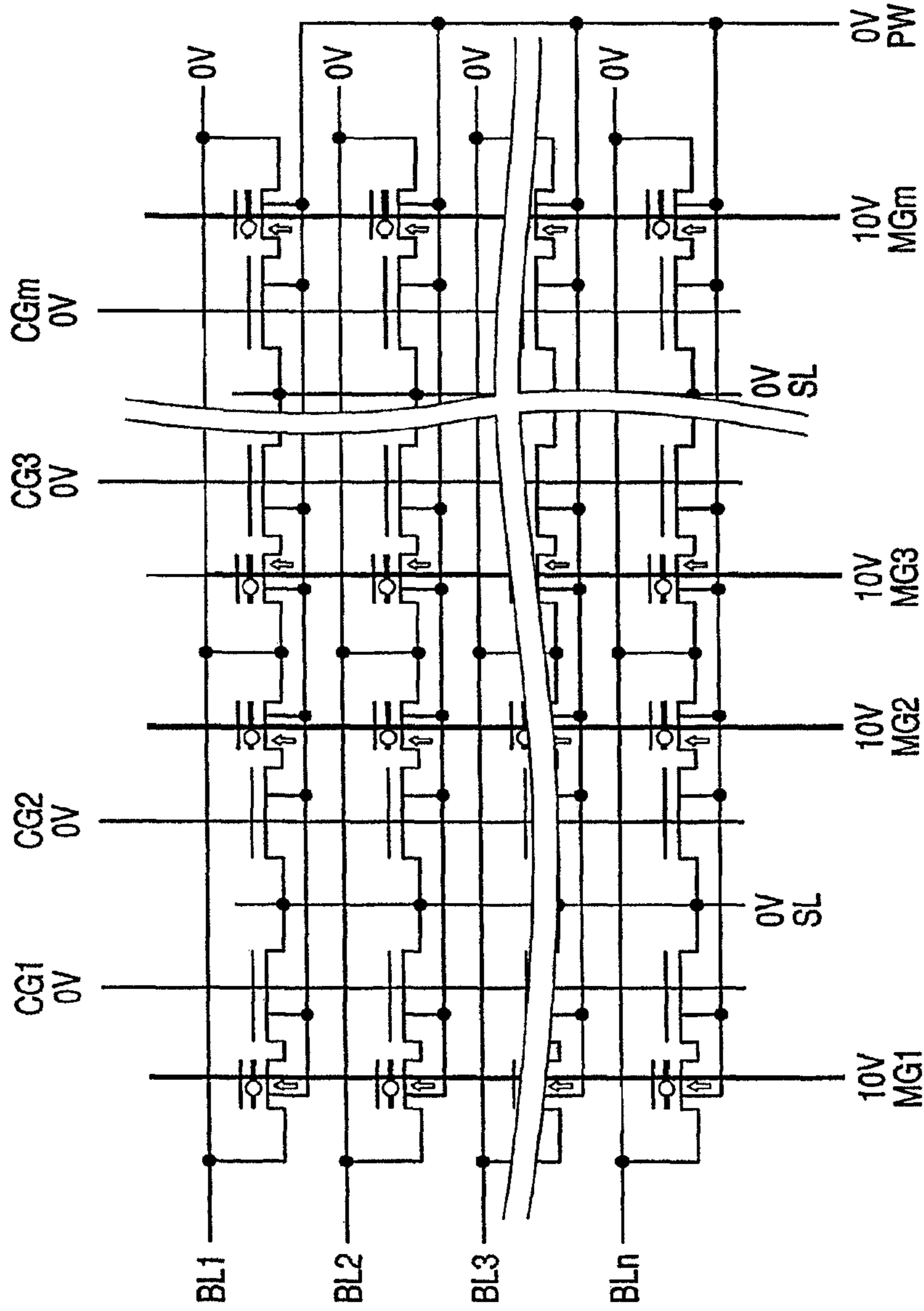
FIG. 10 (ERASE OPERATION)
