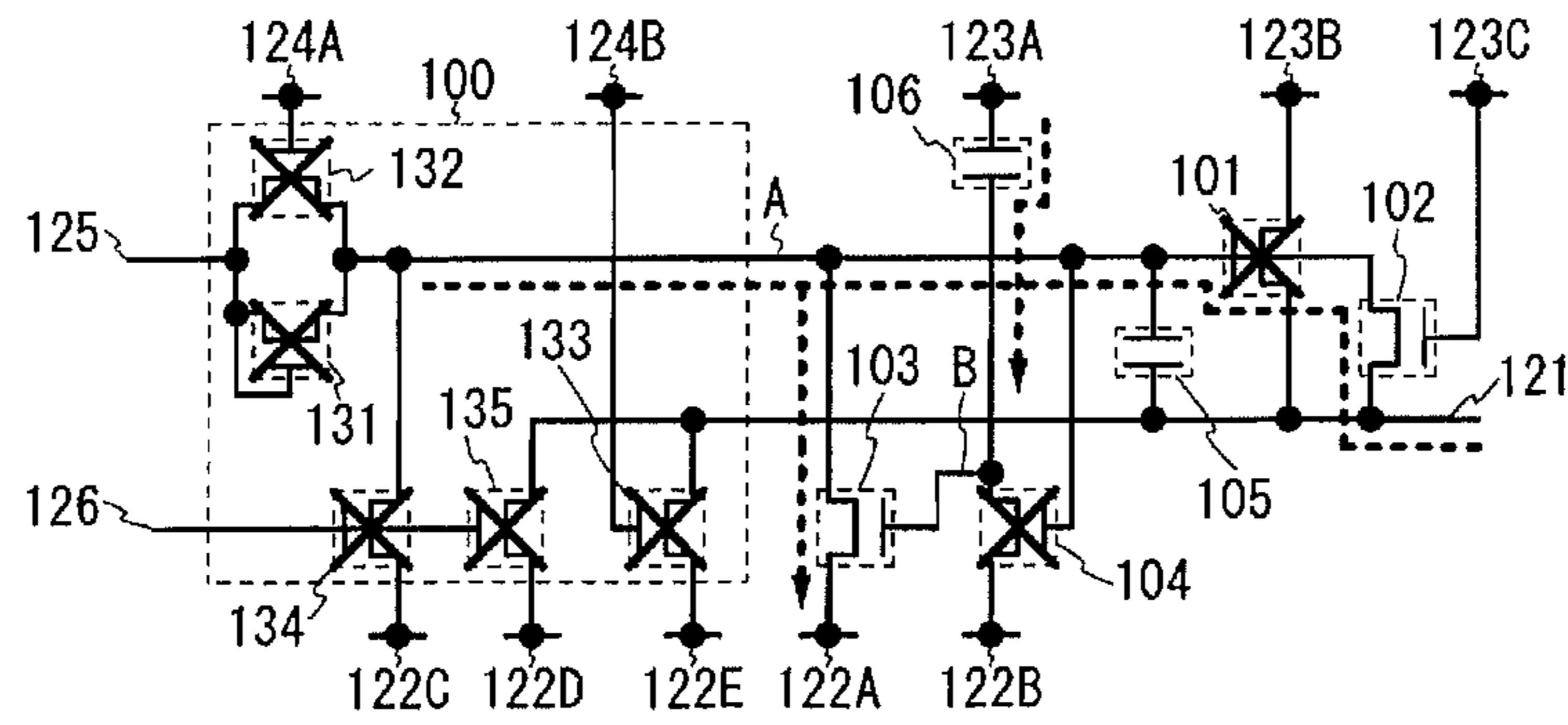
FIG. 8A PERIOD T4
