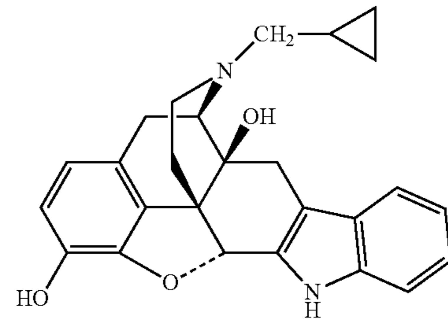
Naltrindole
