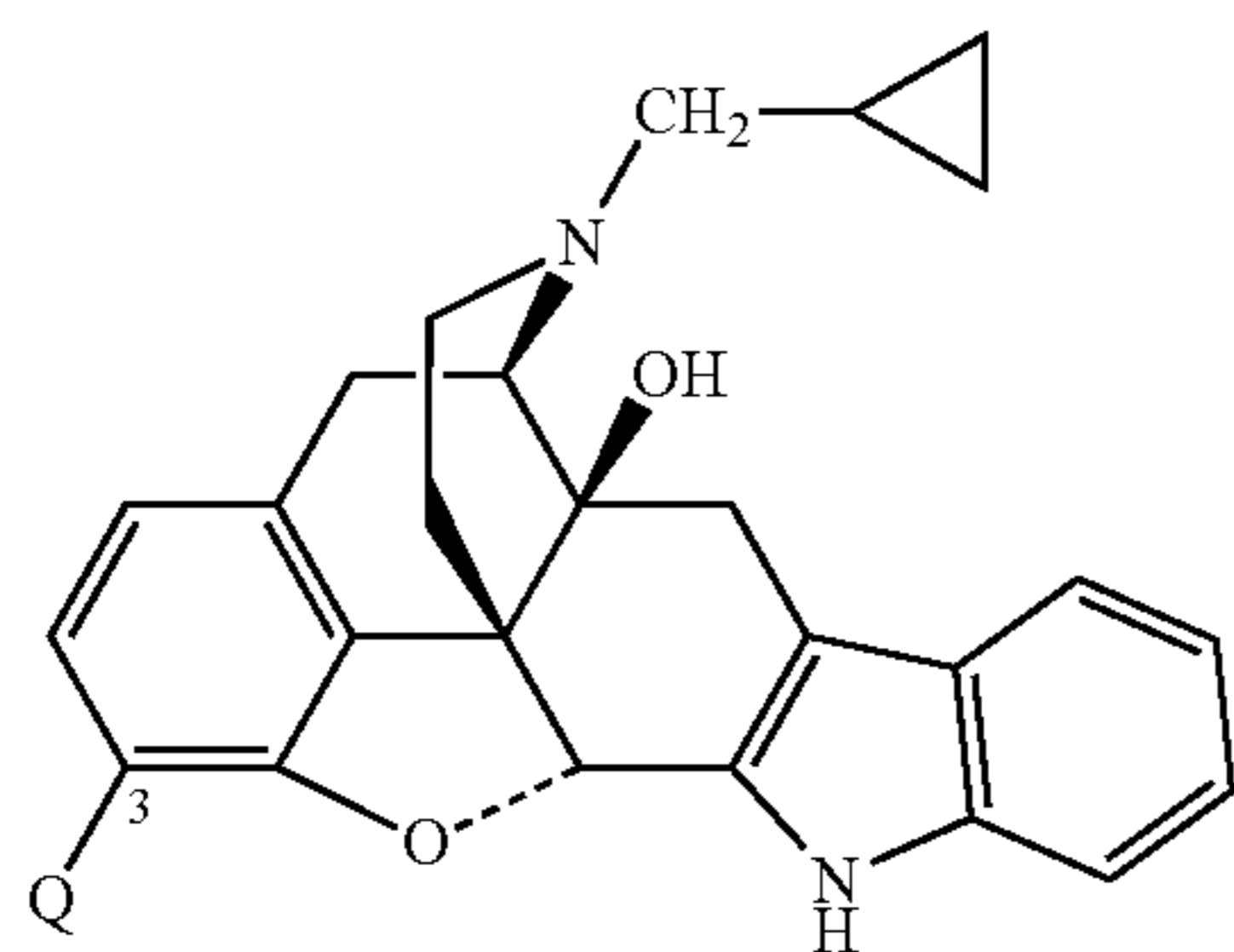
Naltrindole core
