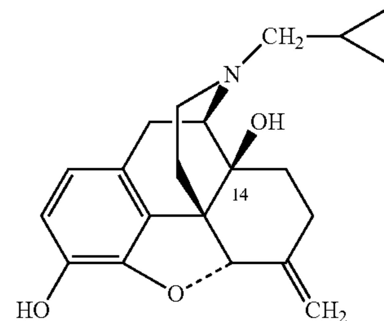
Nalmefene
