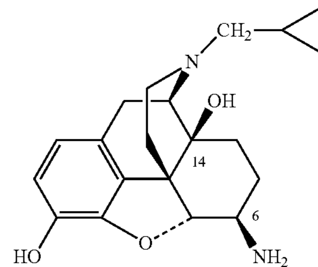
β-Naltrexamine
