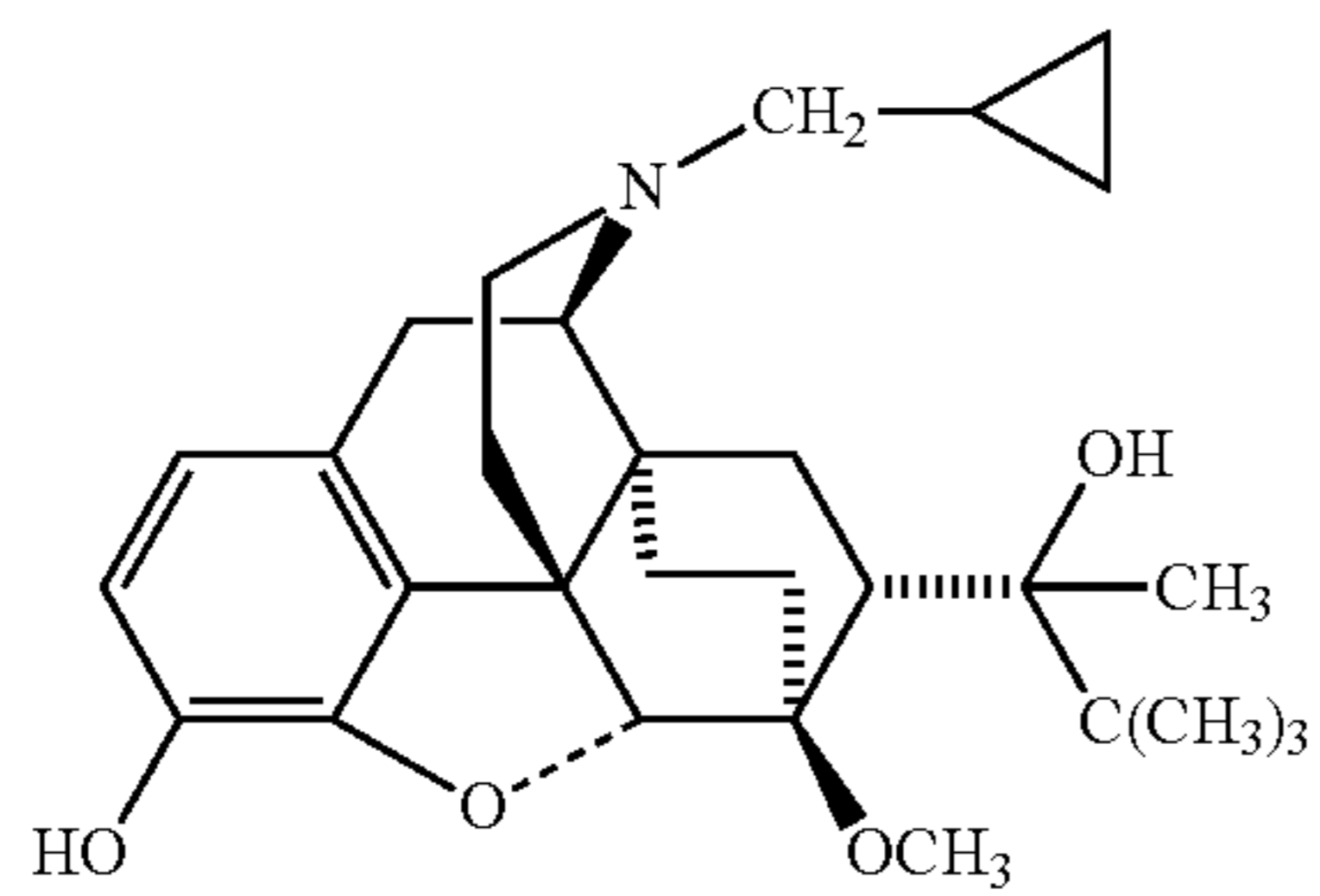
Buprenorphine
