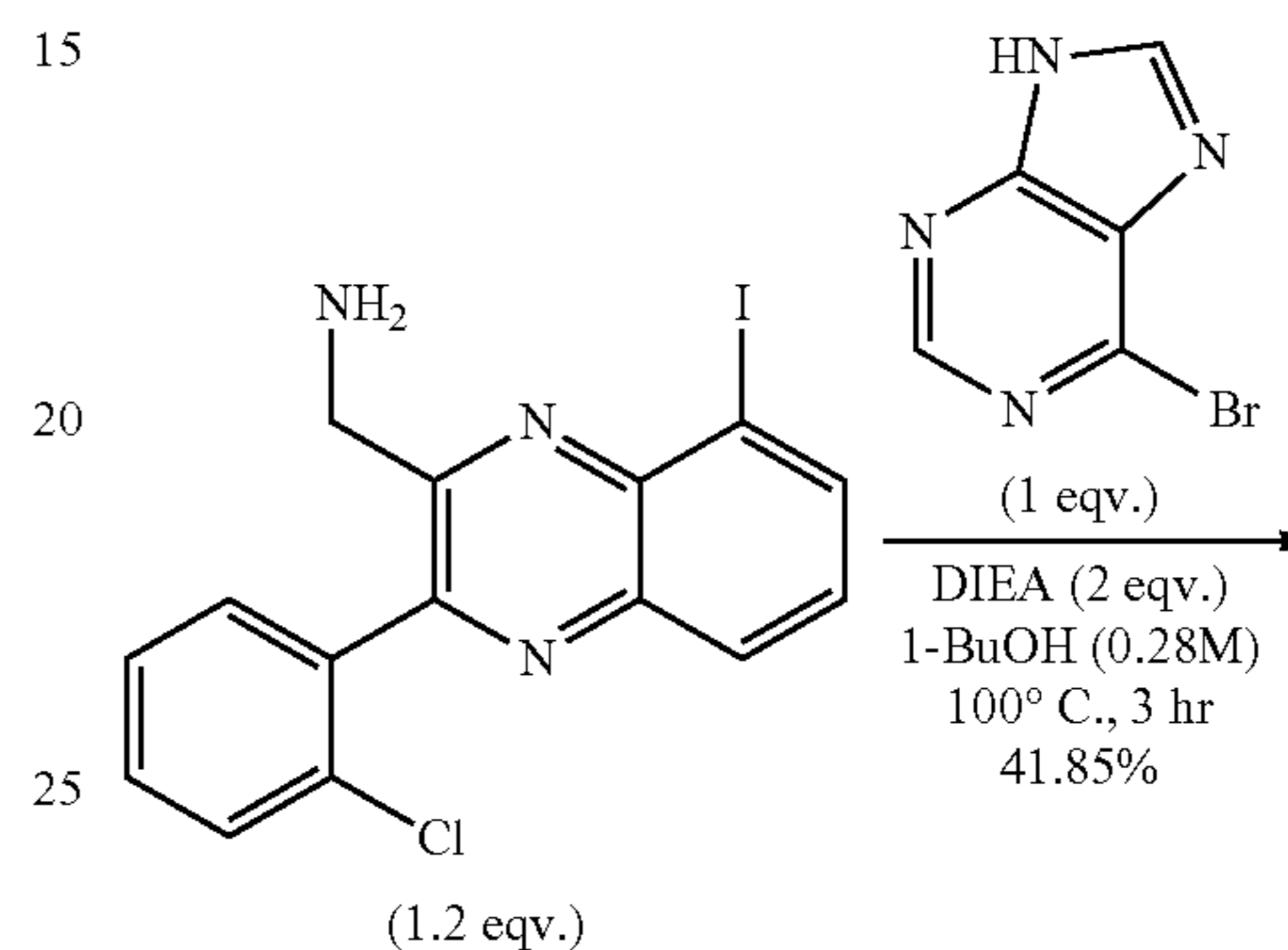
(3-(2-Chlorophenyl)-8-iodoquinoxalin-2-yl)methanamine
