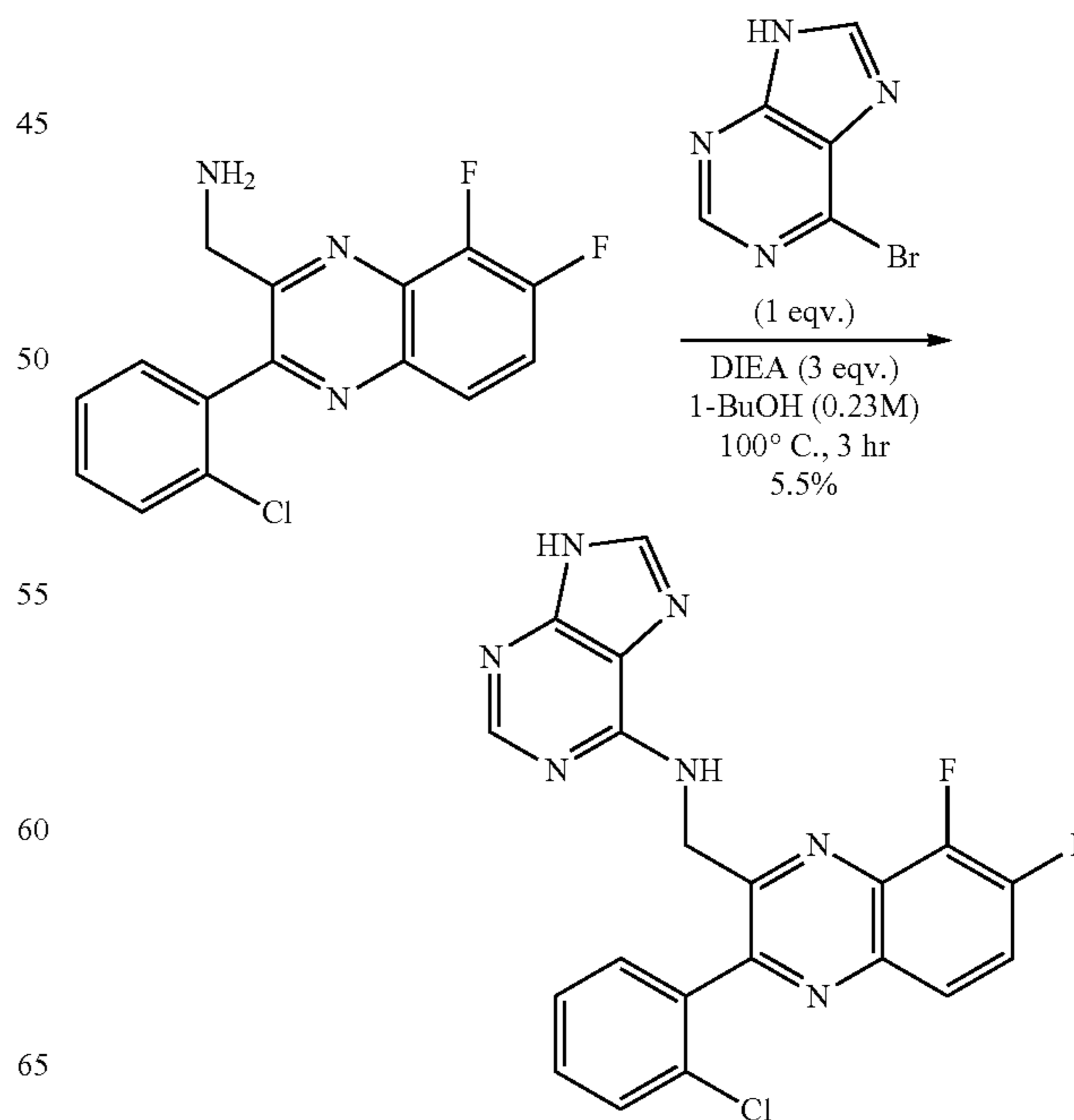
N-((3-(2-Chlorophenyl)-5,6-difluoroquinoxalin-2-yl)methyl)-9H-purin-6-amine
