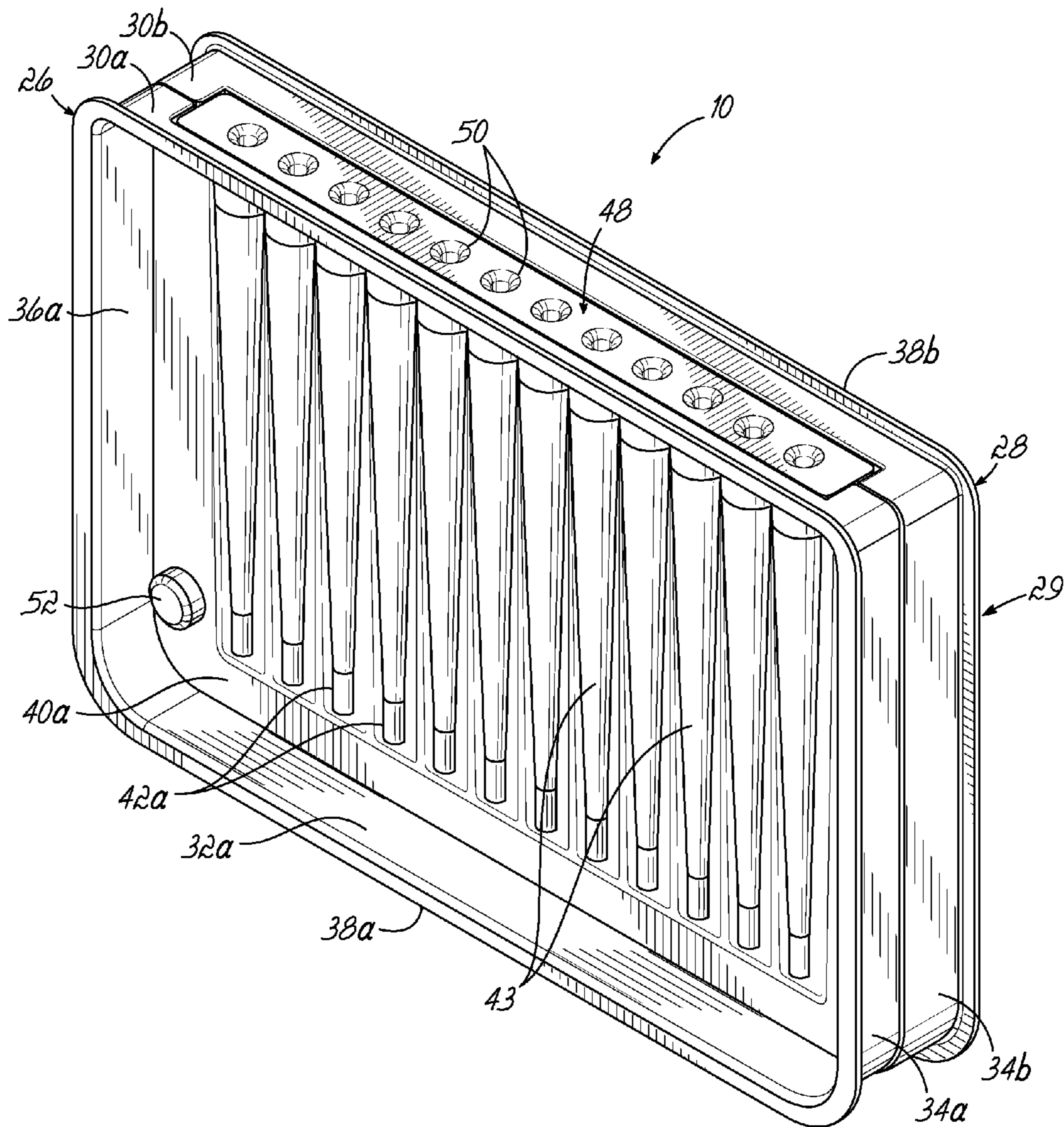
FIG. 4
