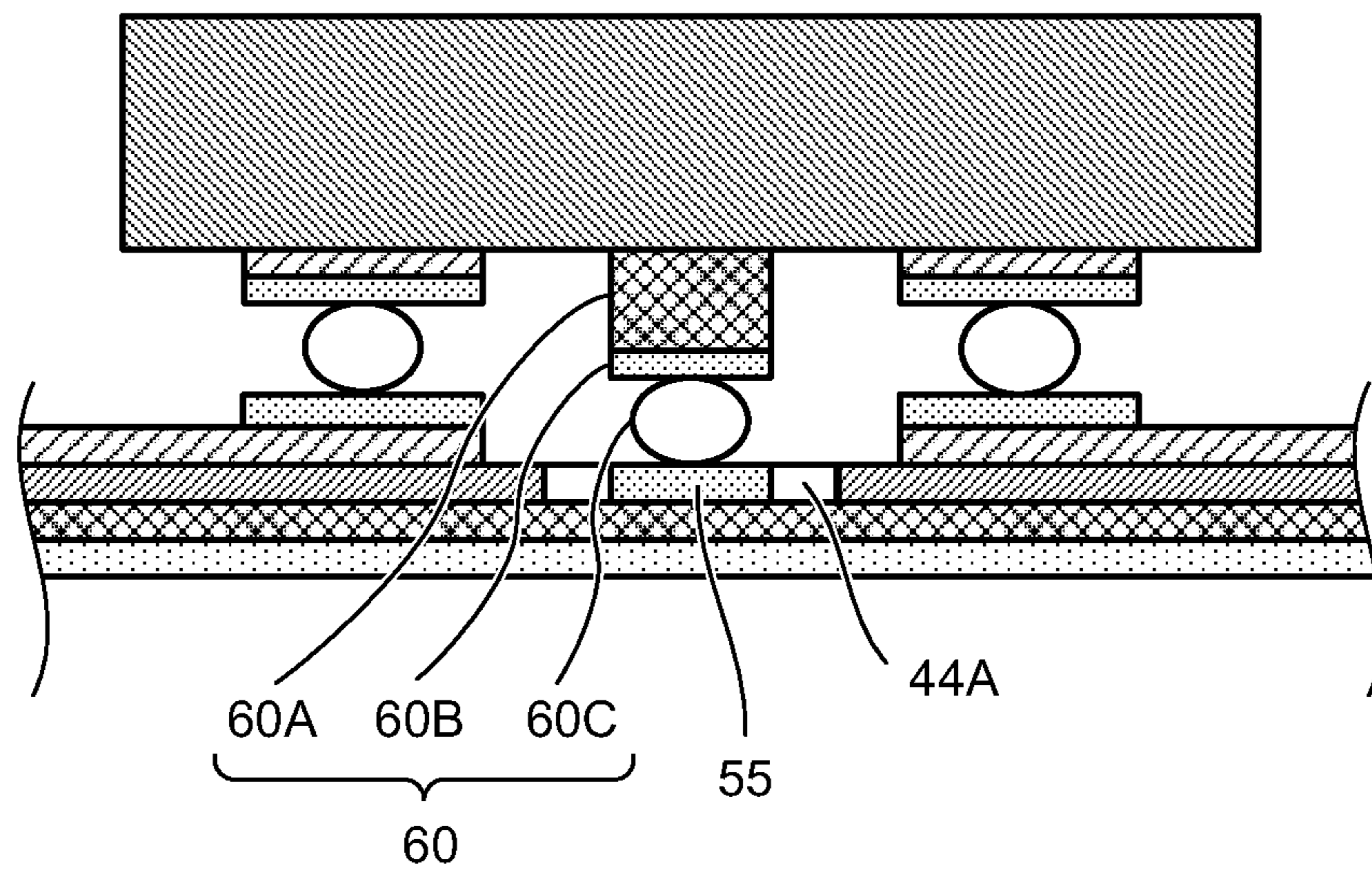
FIG.4
