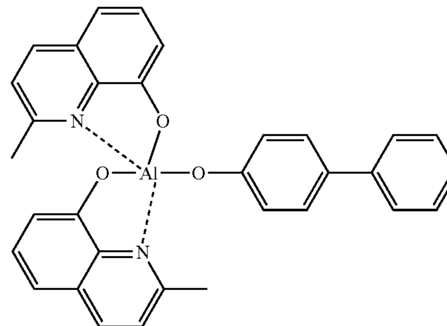
BALq
