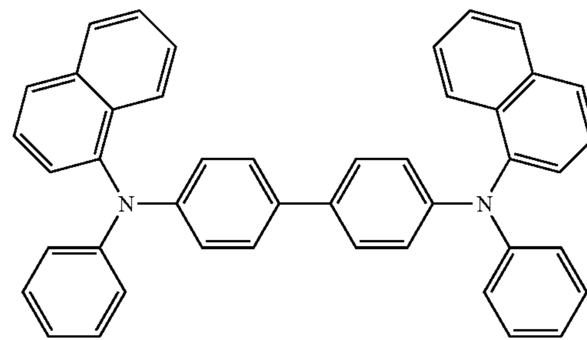
\alpha -NPD
