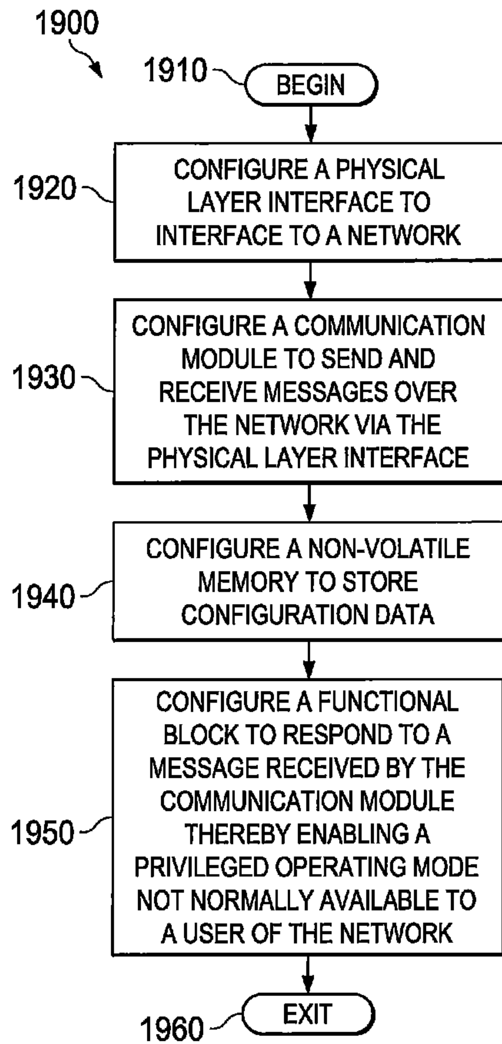
FIG. 19
