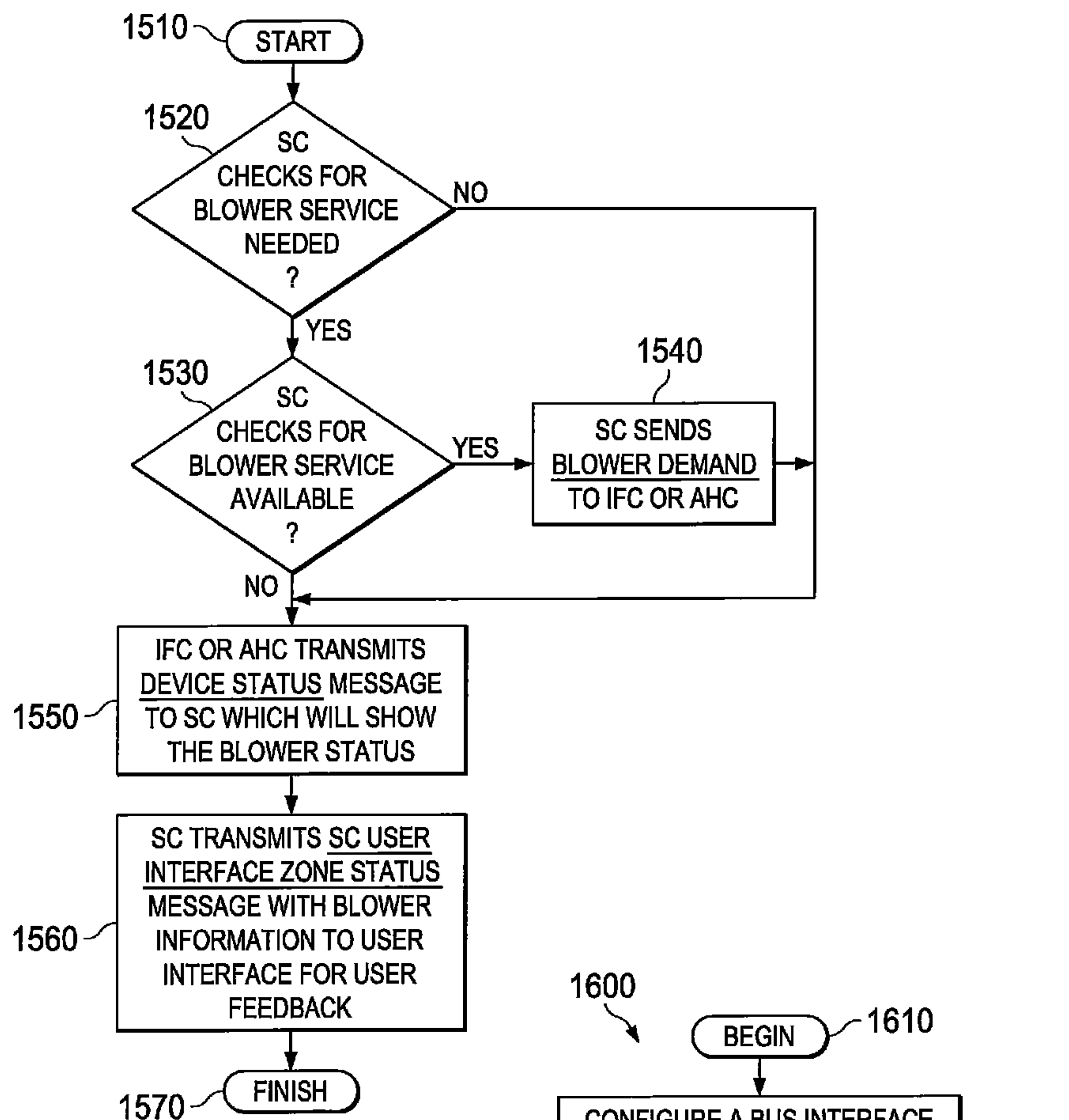
FIG. 15
