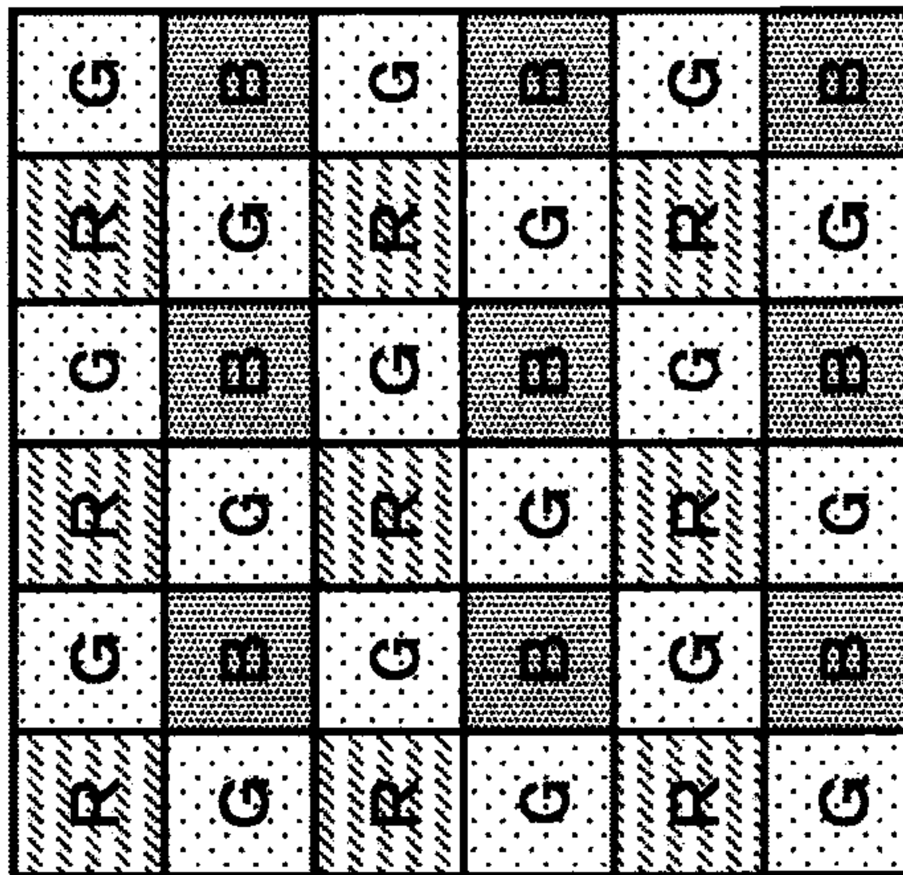
(1) BAYER ARRAY
