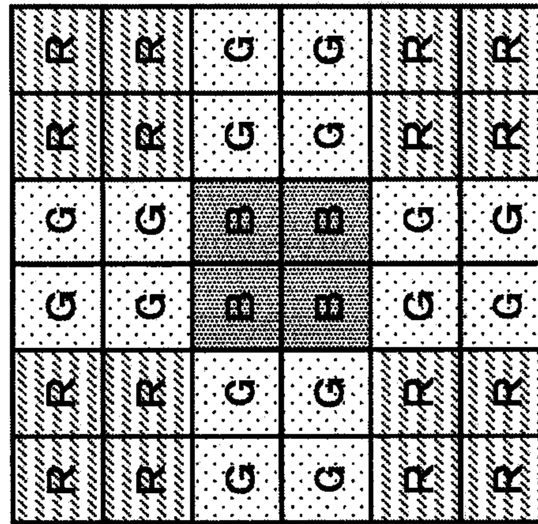
(2) 4-DIVISION BAYER / RGB ARRAY
