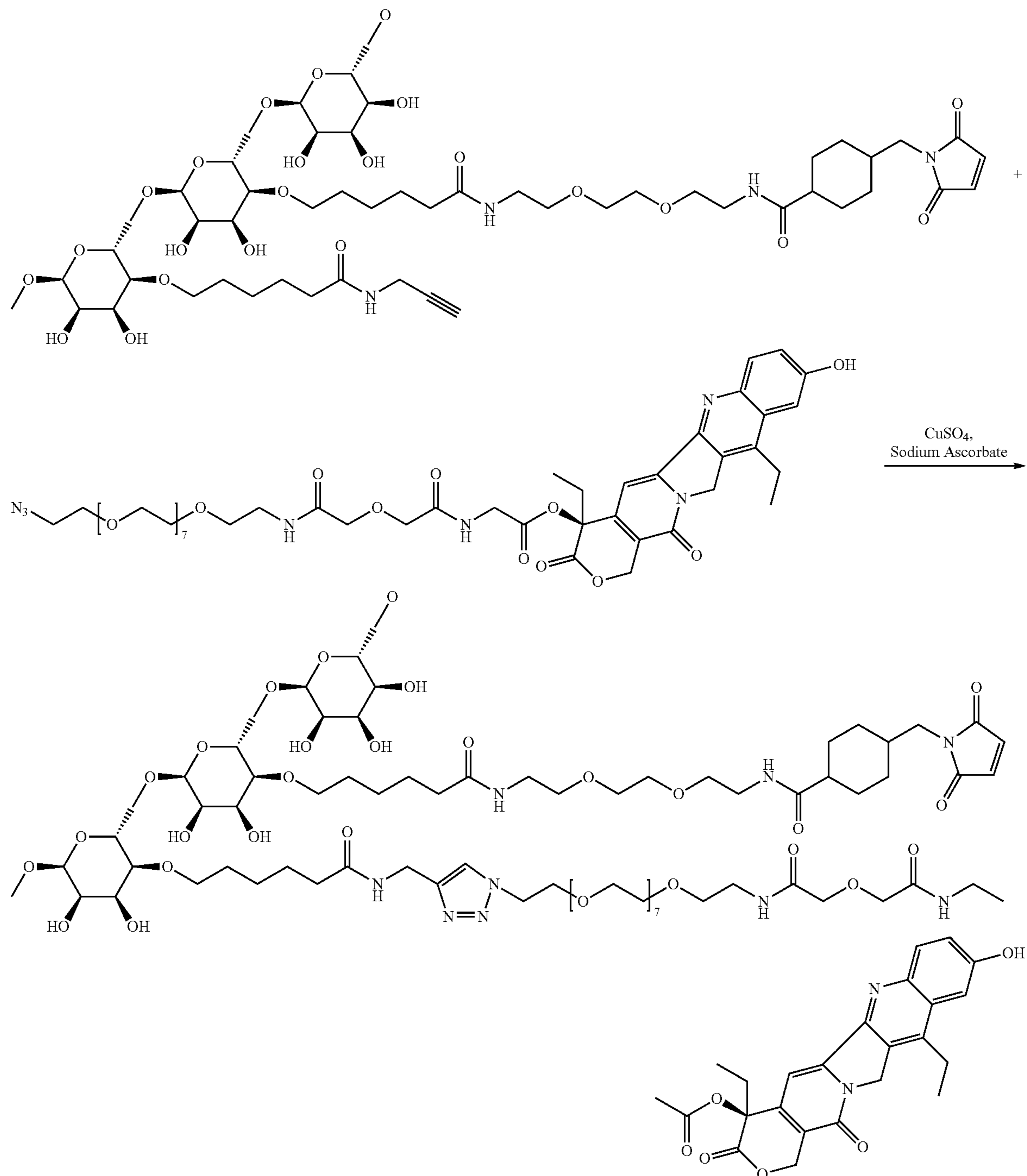
Scheme-8
