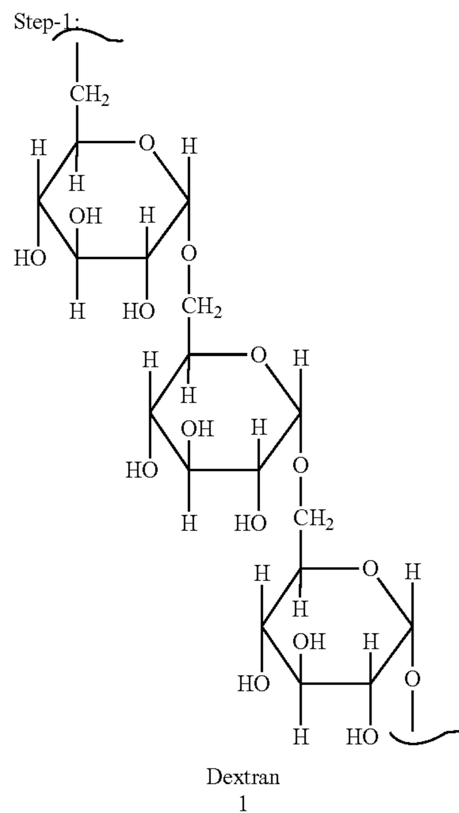
Scheme-1
