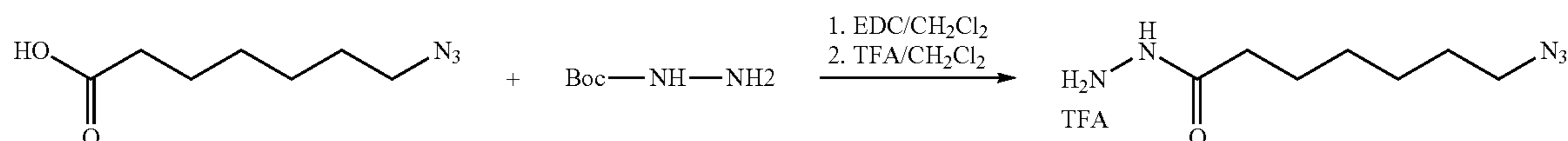
Scheme-2
