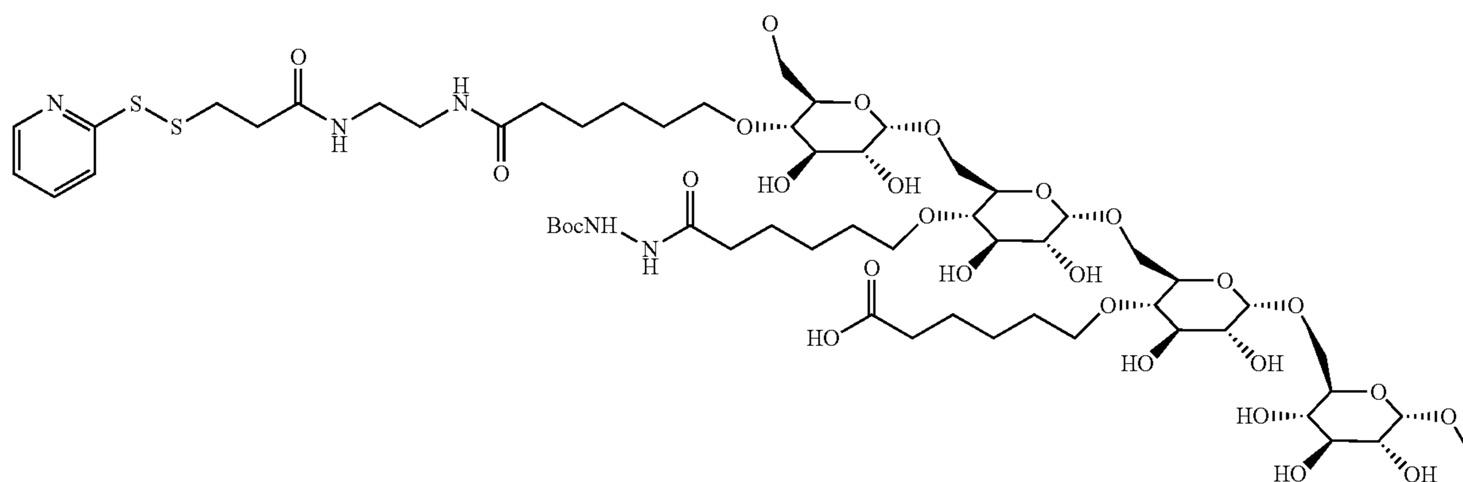
Structure-7
