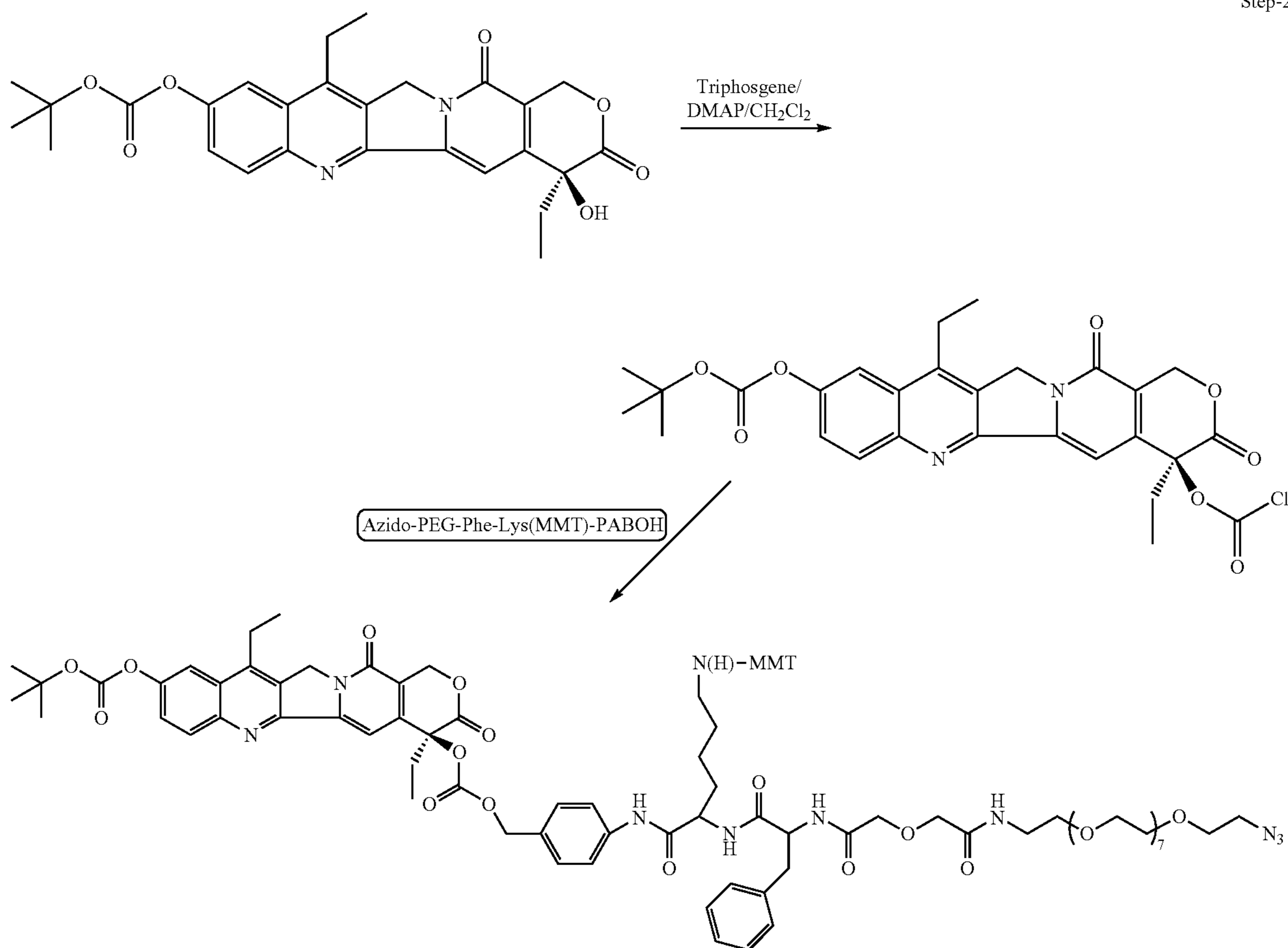
Azido-PEG-Phe-Lys(MMT)-PABOH
