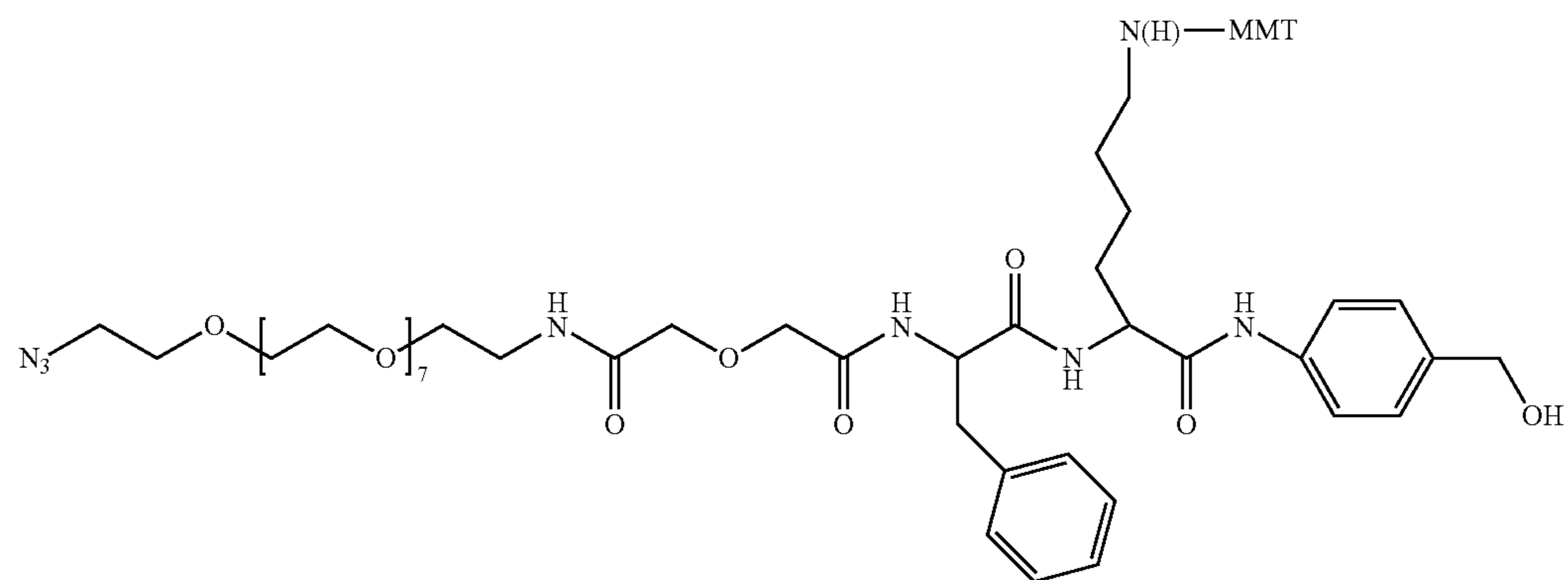
Azido-PEG-Phe-Lys(MMT)-PABOH
