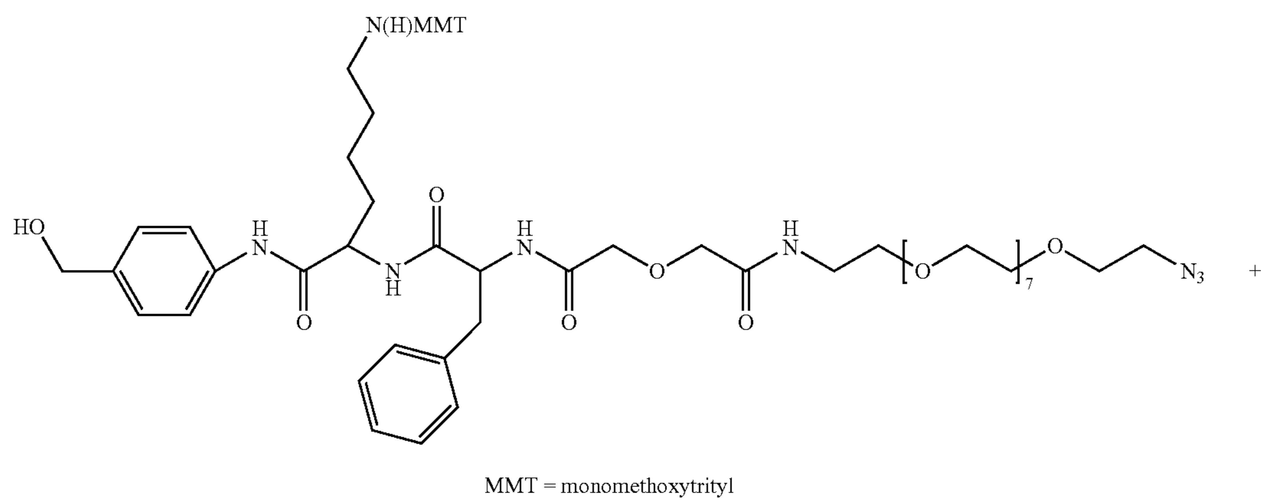
Scheme-5
