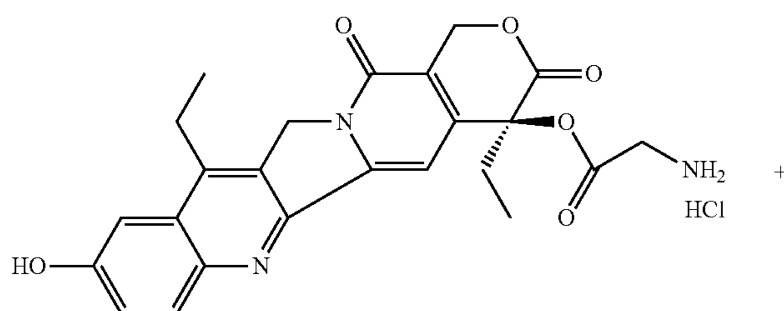
Scheme-3
