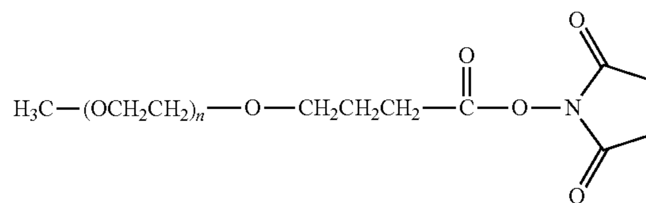
mPEG-Succinimidyl Butanoate
