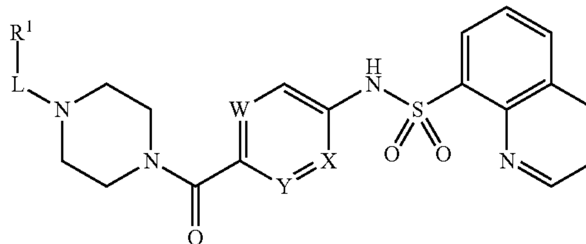
Formula Ij
