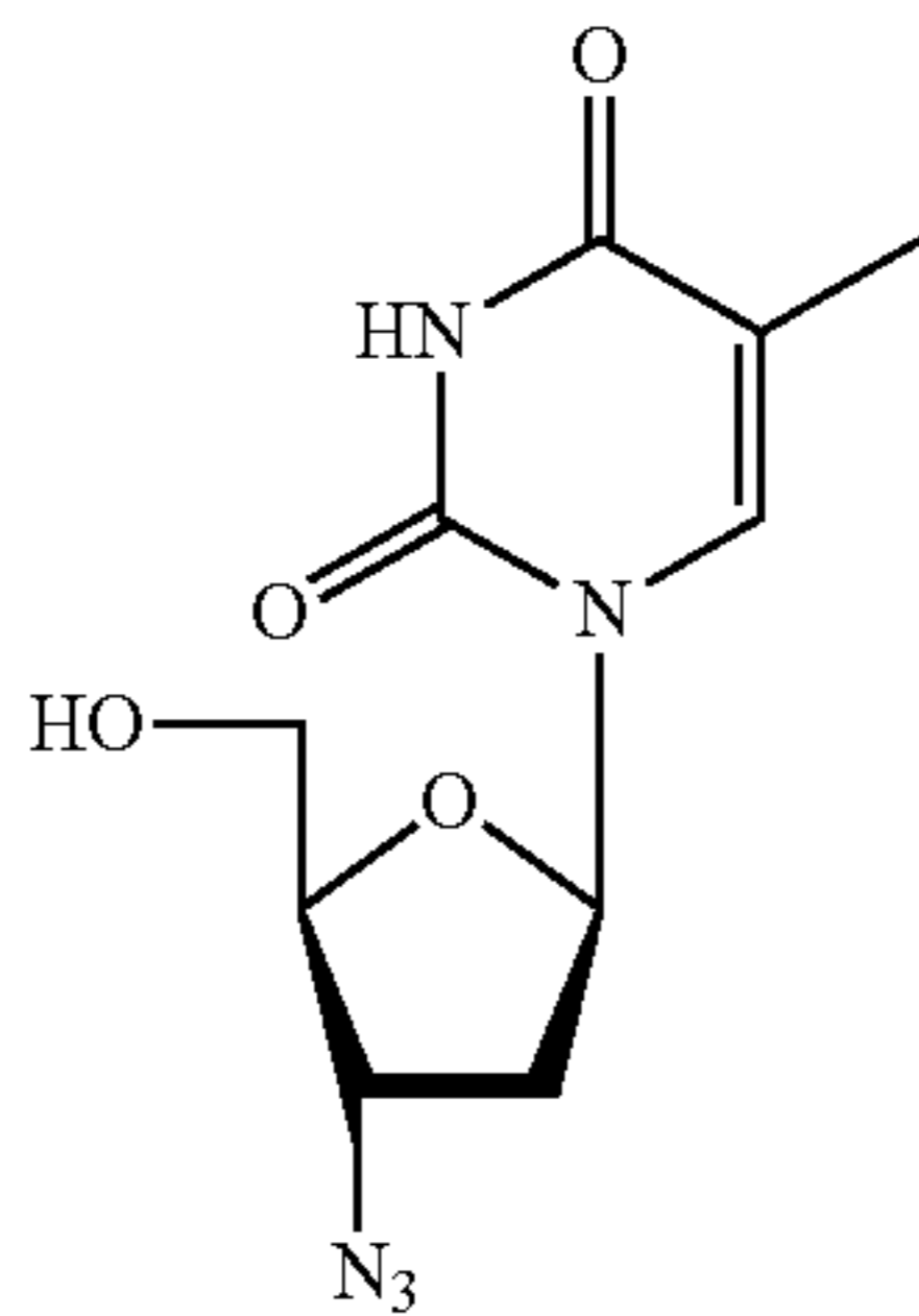
AZT
