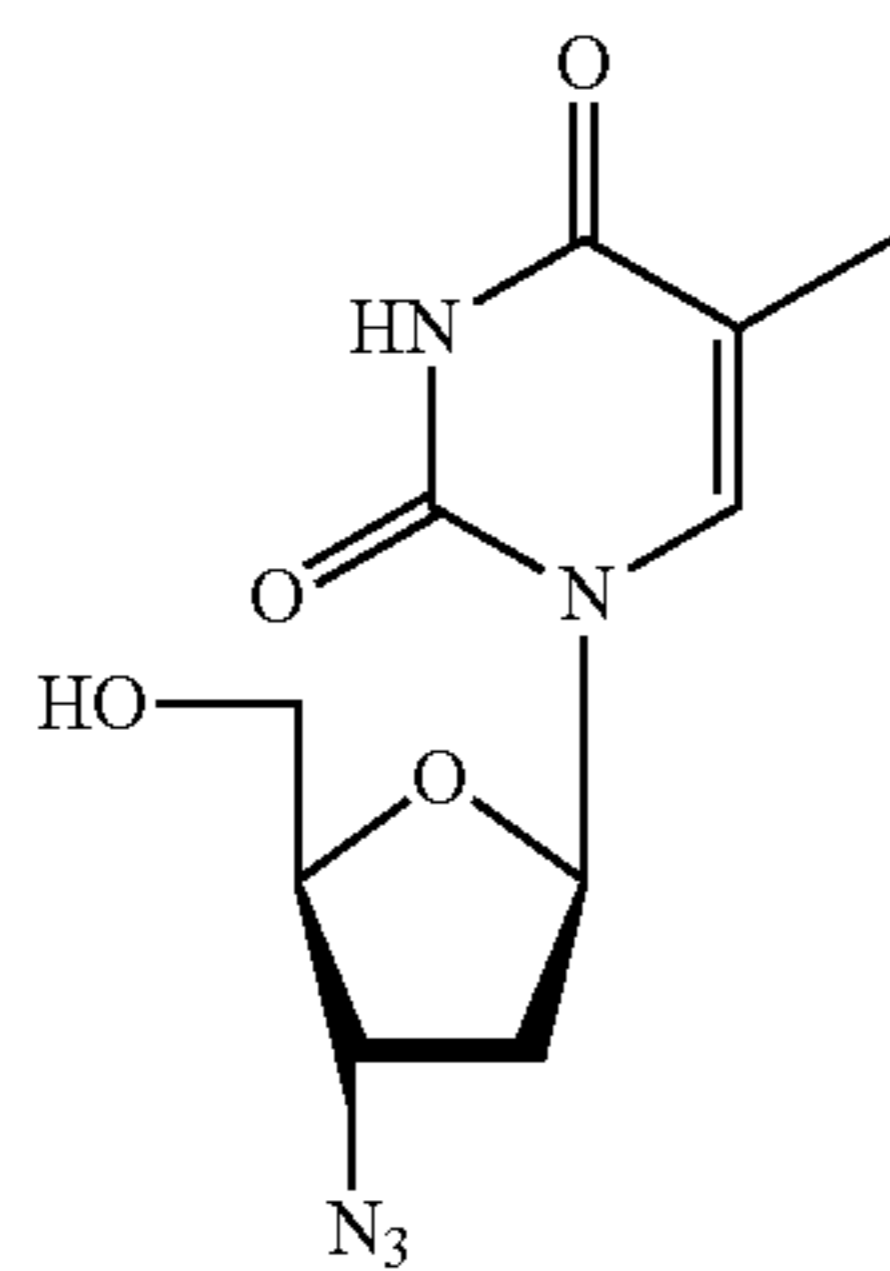
AZT
