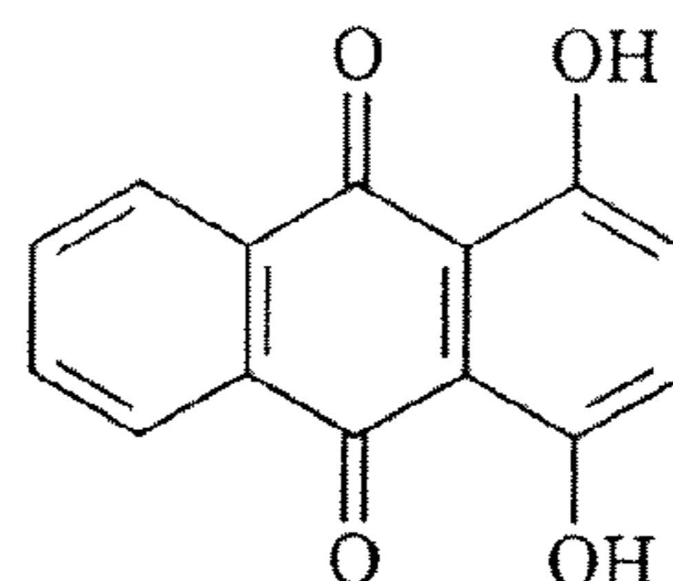
quinizarin 8
