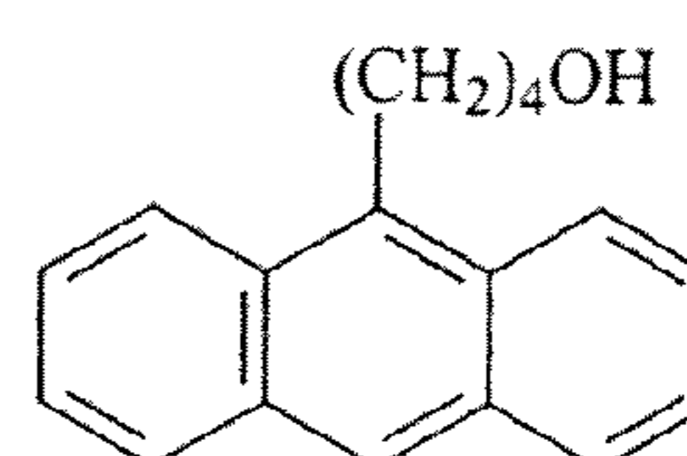
9-anthracene butanol 6
