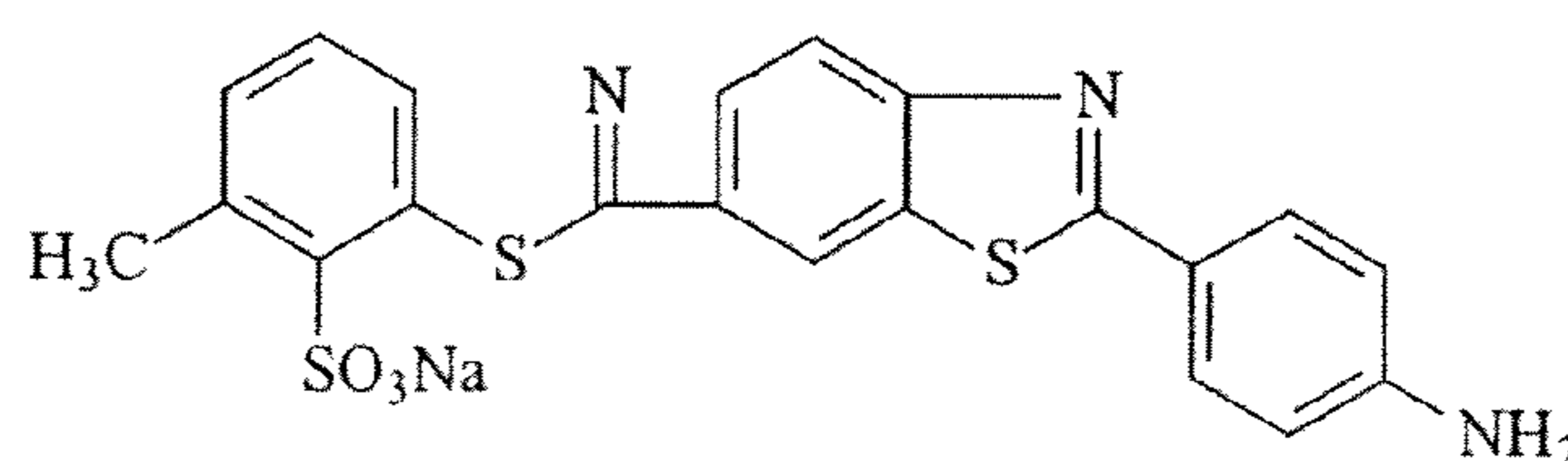
primuline 9
