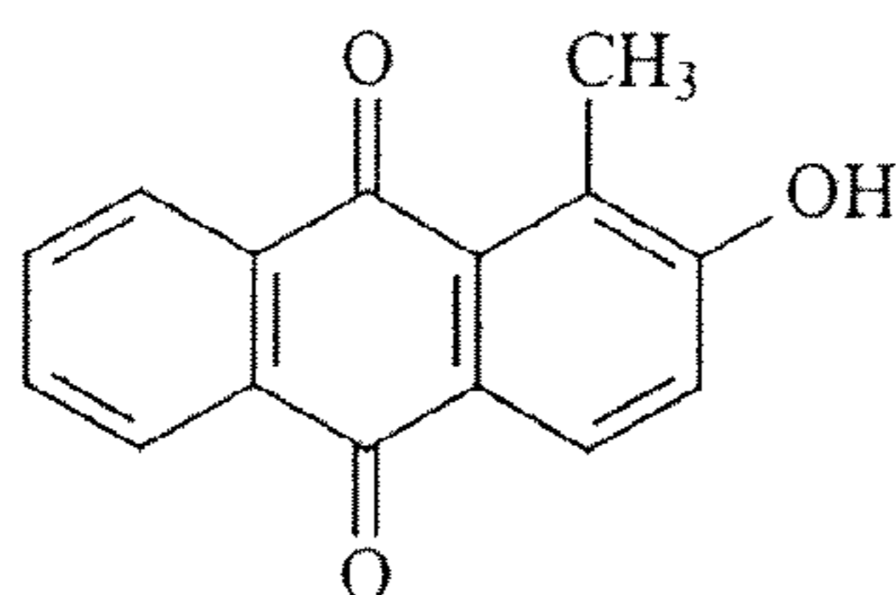
alizarin 7
