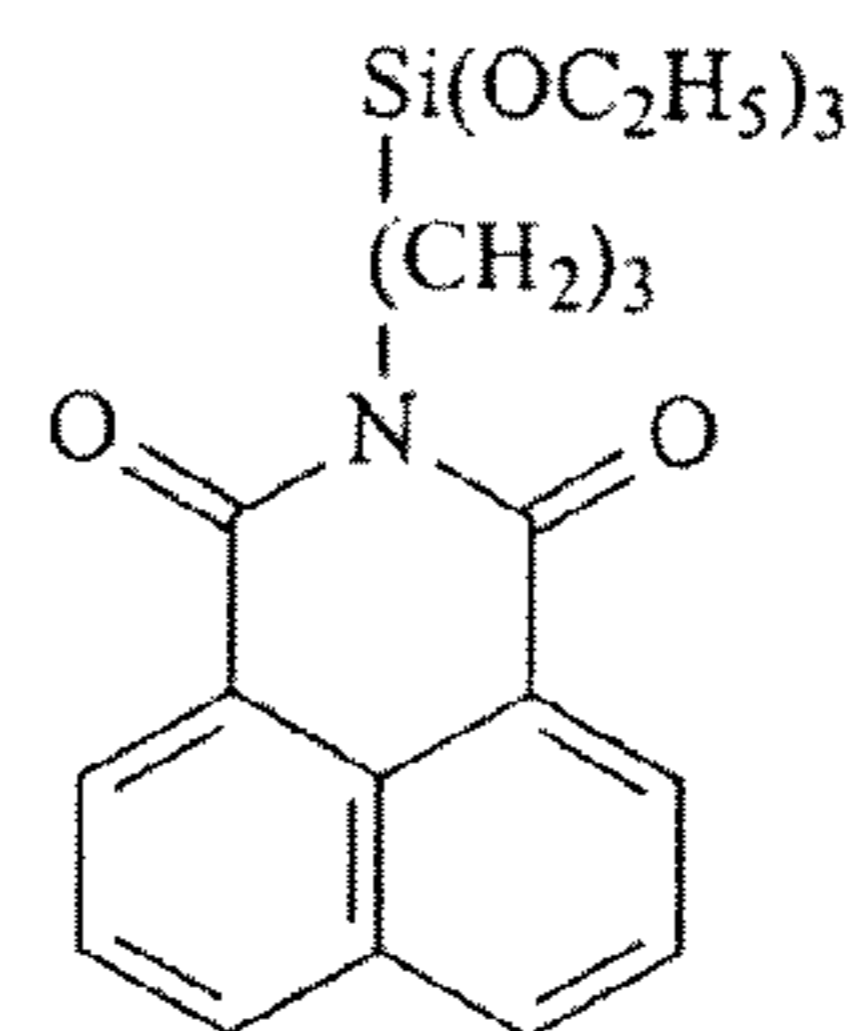
triethoxysilylpropyl-1,8-naphthalimide
