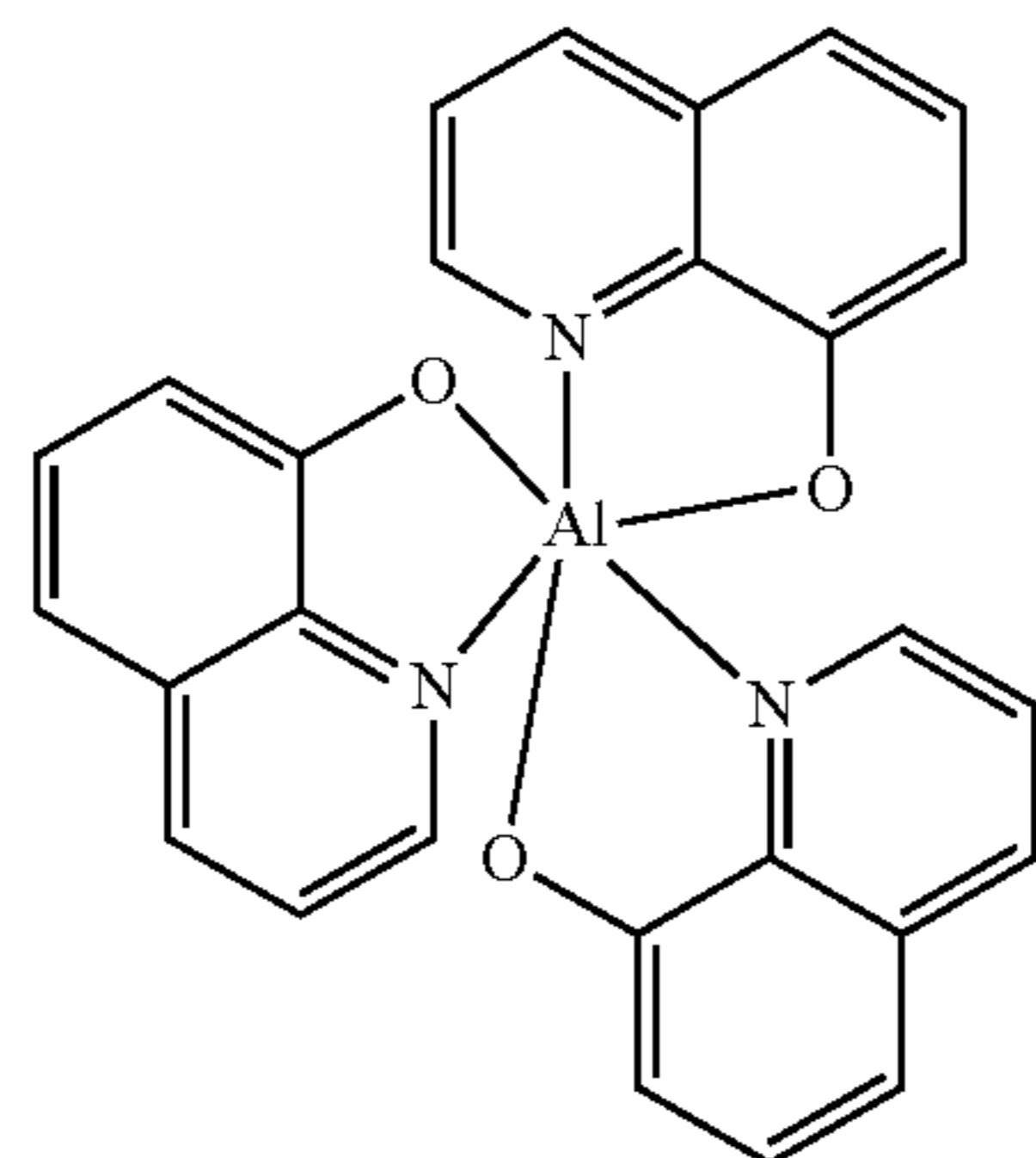
Alq3
