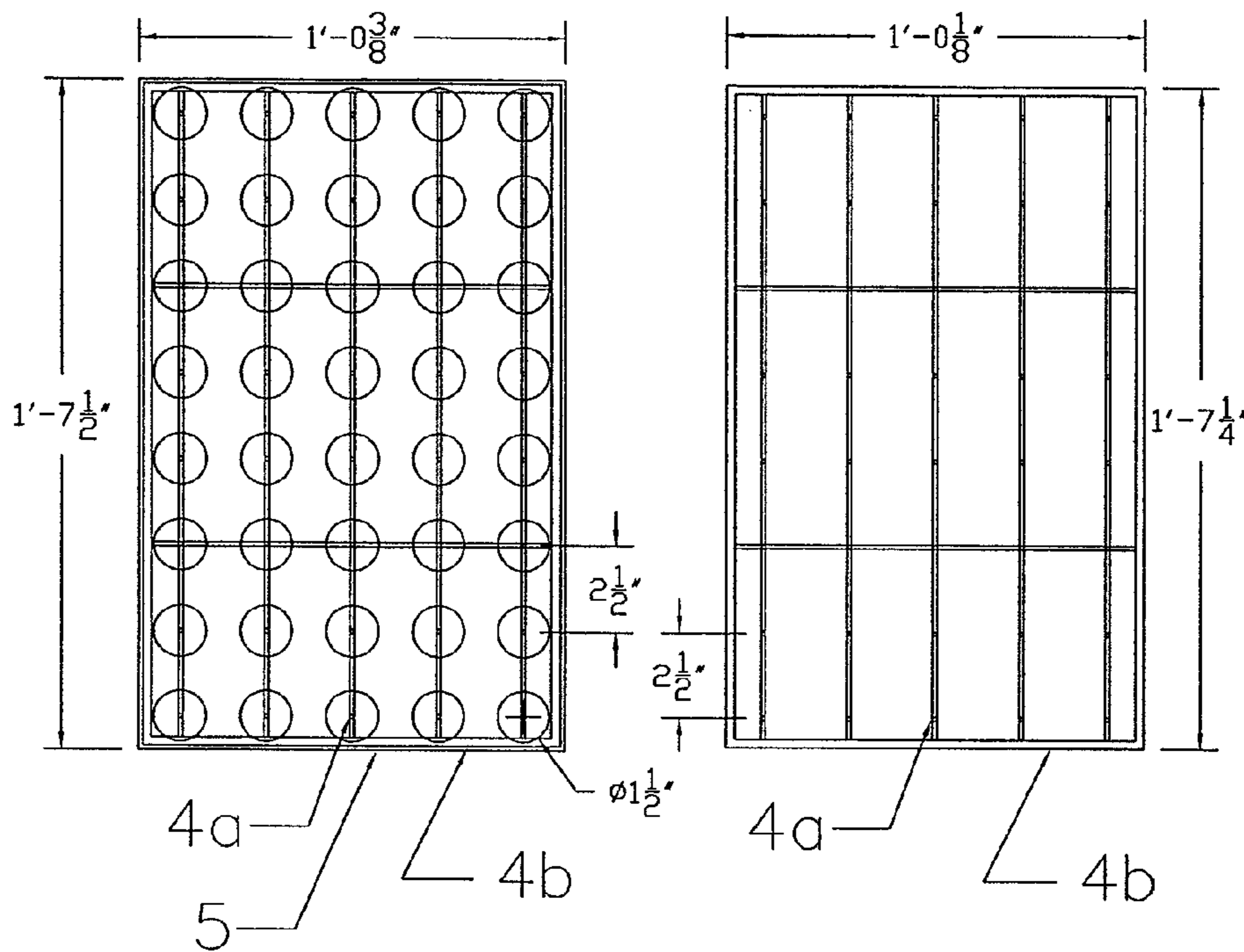
FIG. 8A: TOP VIEW
