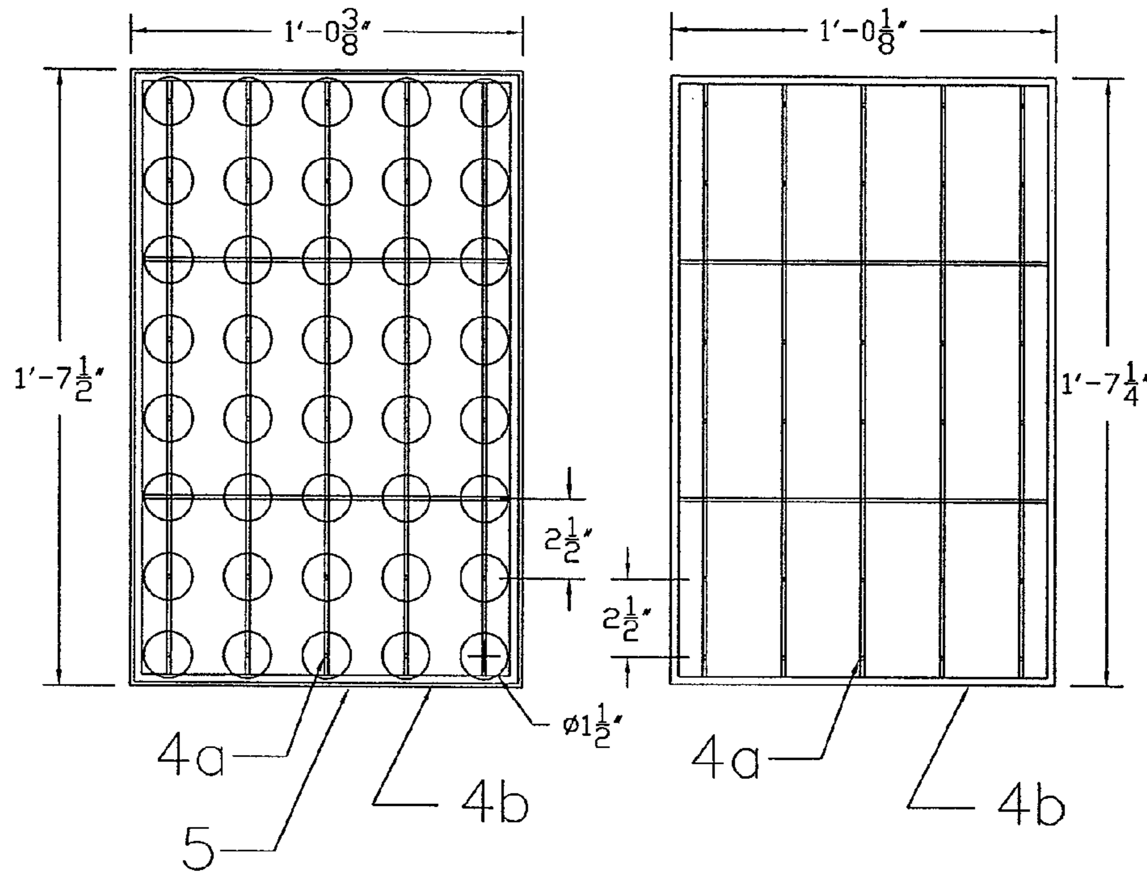
FIG. 8C: IONIZER GRID
