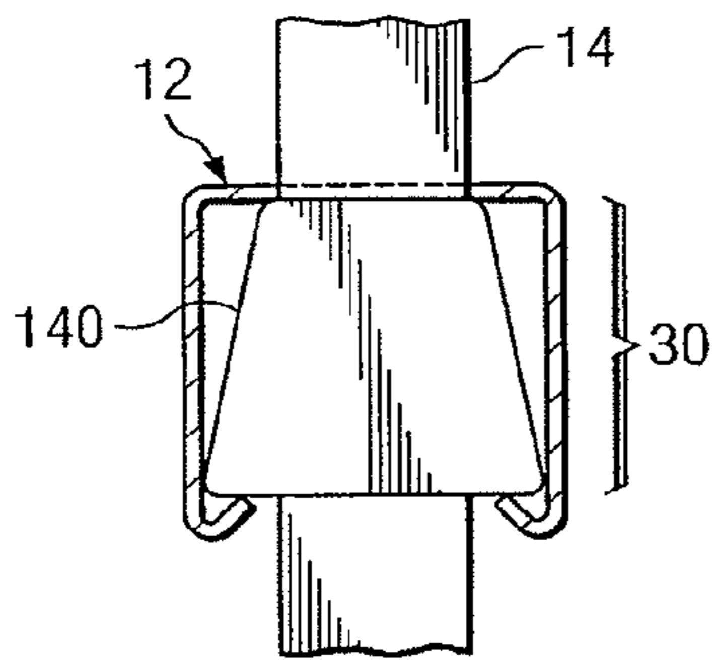
FIG. 12A
