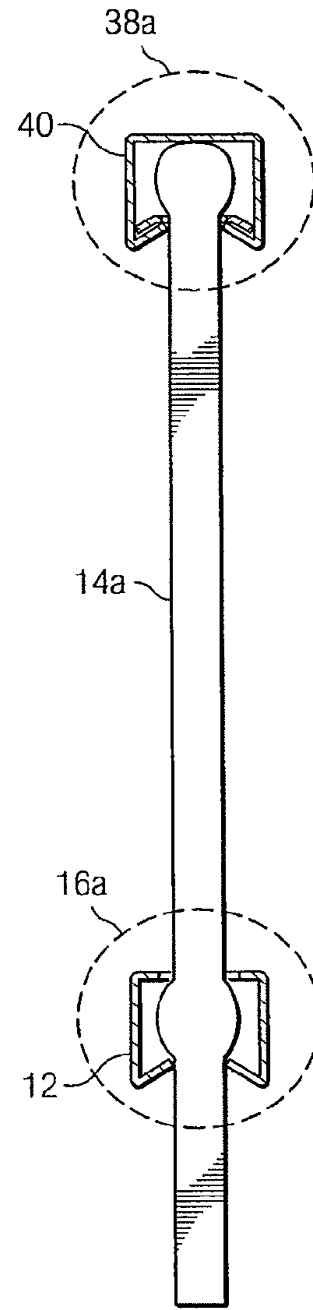
FIG. 6B
