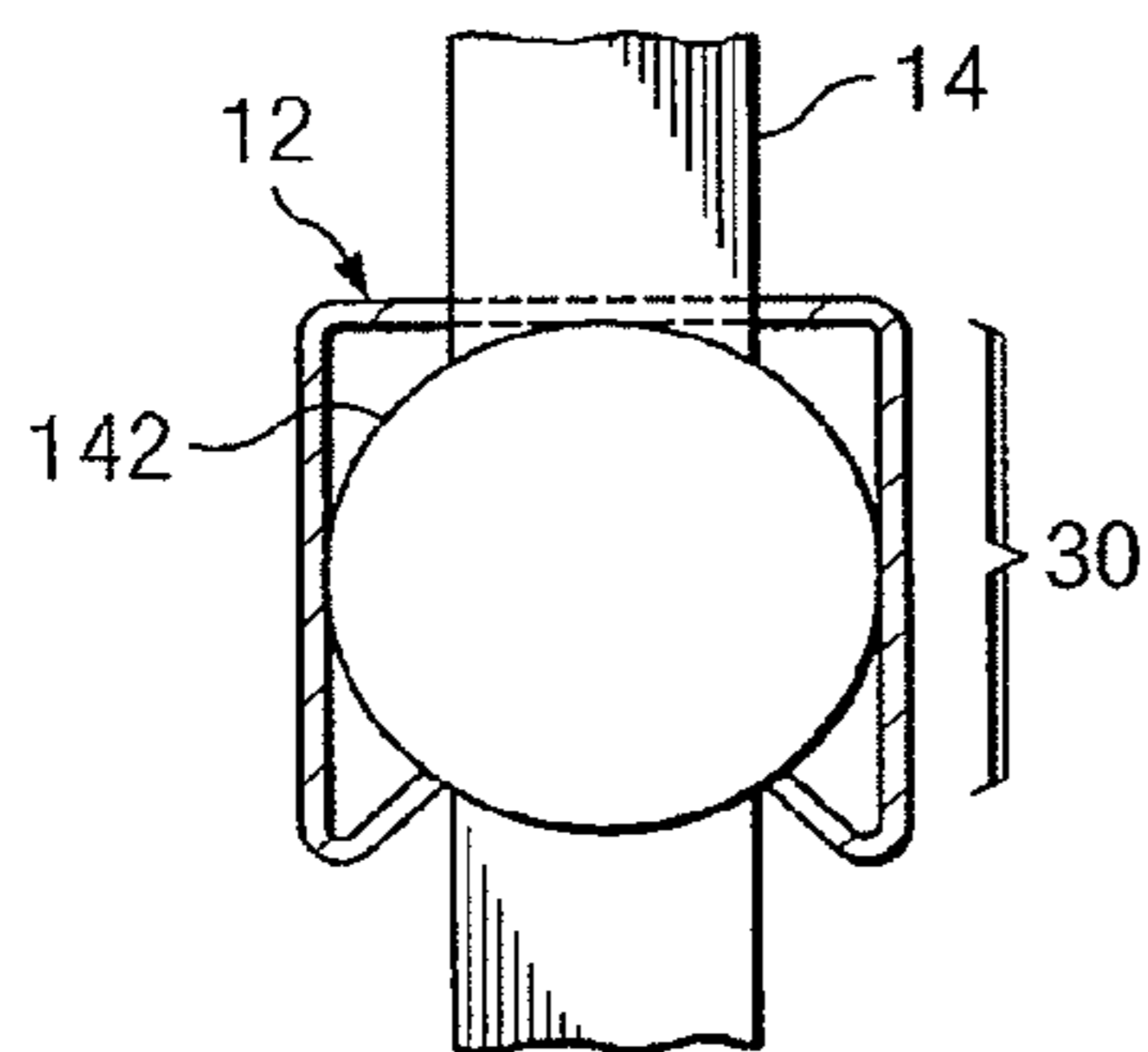
FIG. 13A
