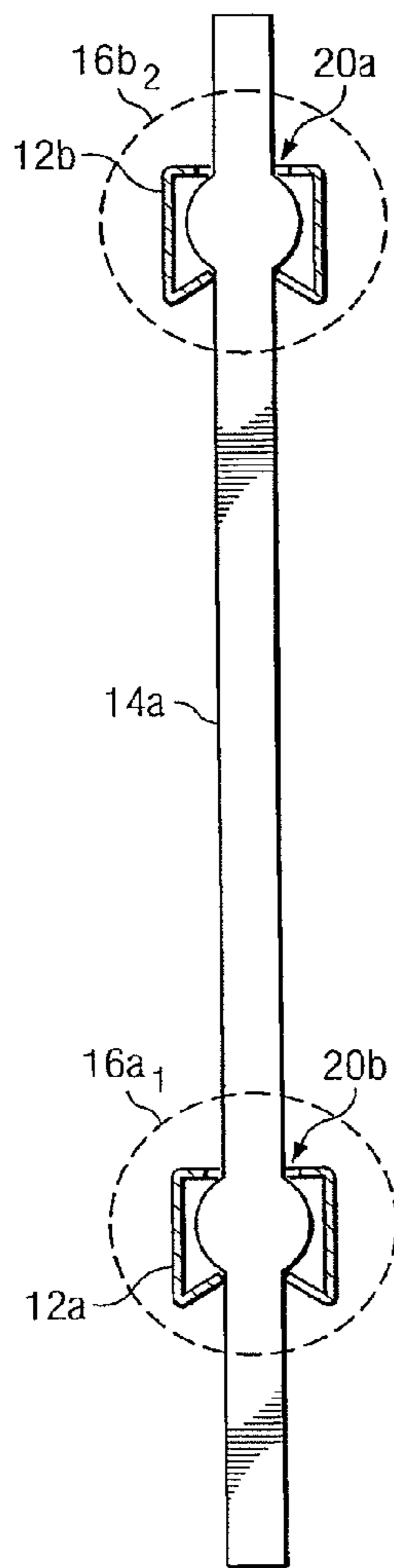
FIG. 3A
