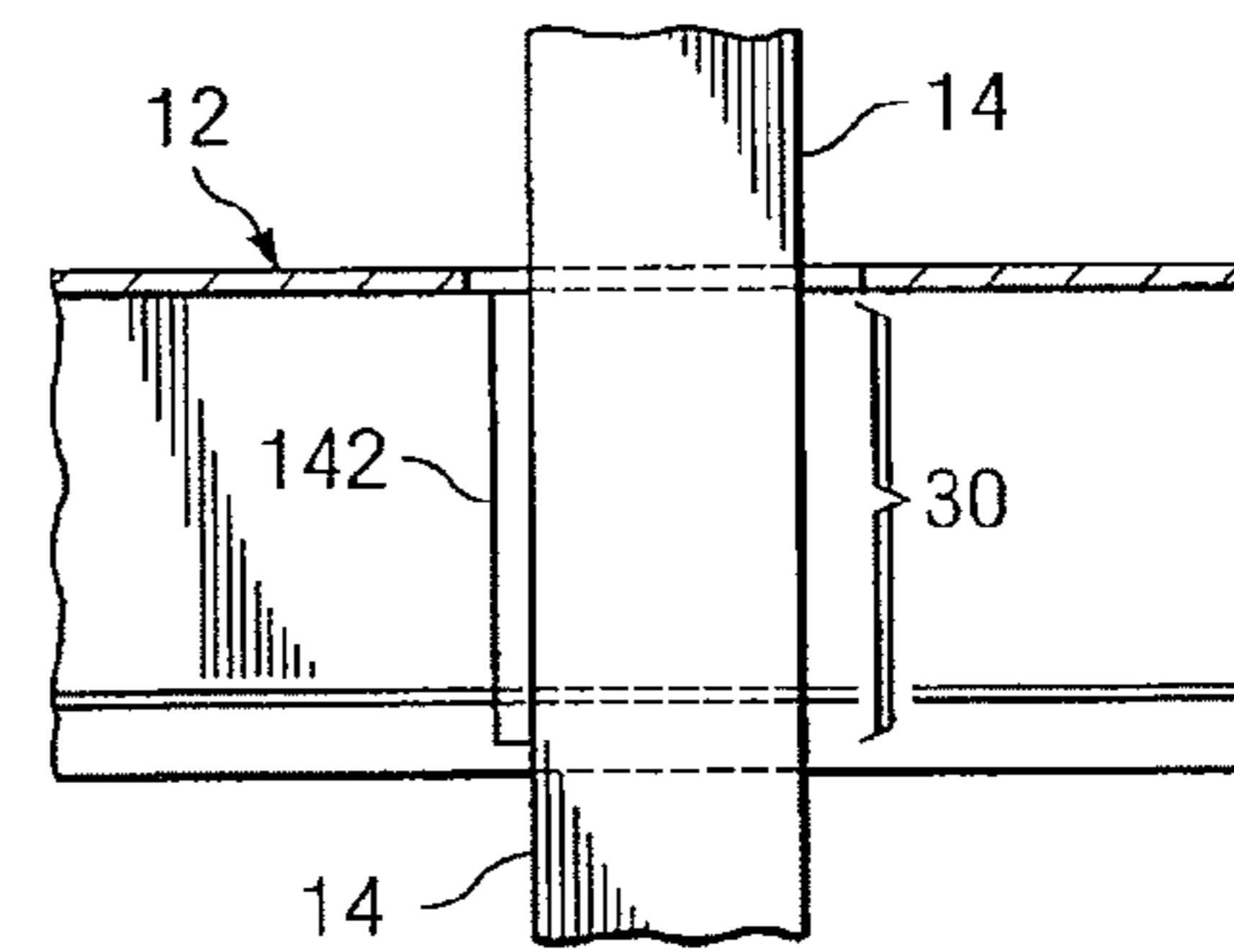
FIG. 13B
