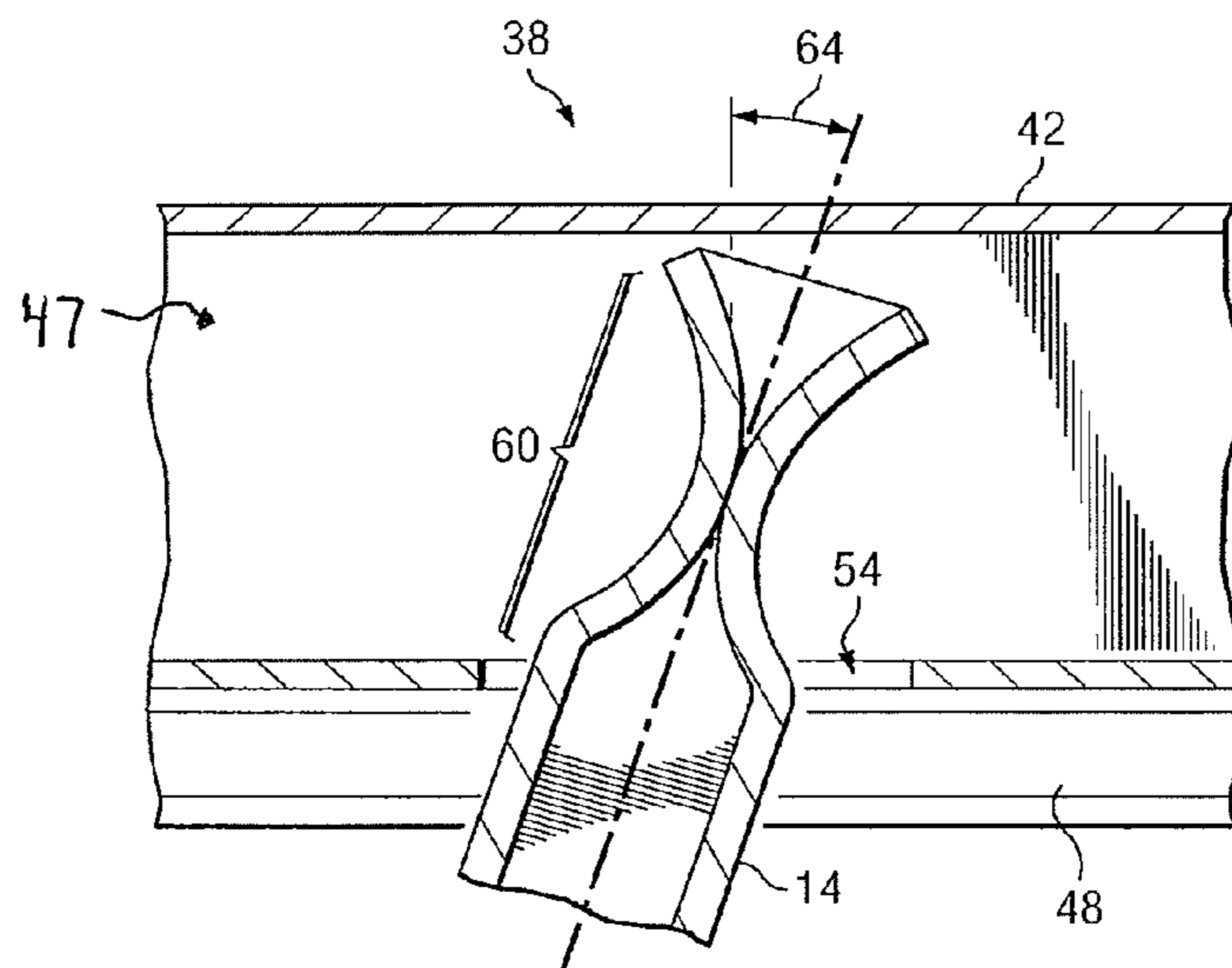
FIG. 5D
