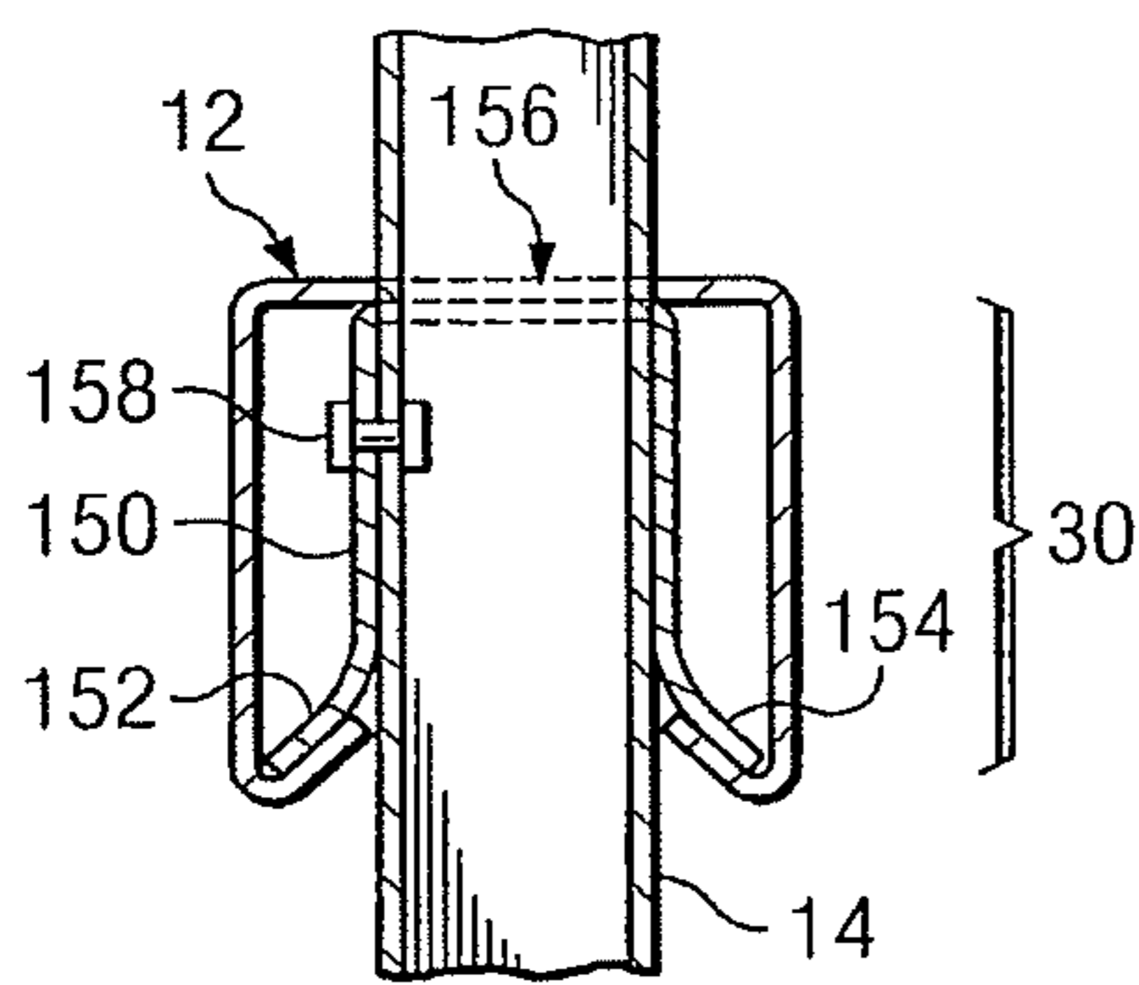
FIG. 15A
