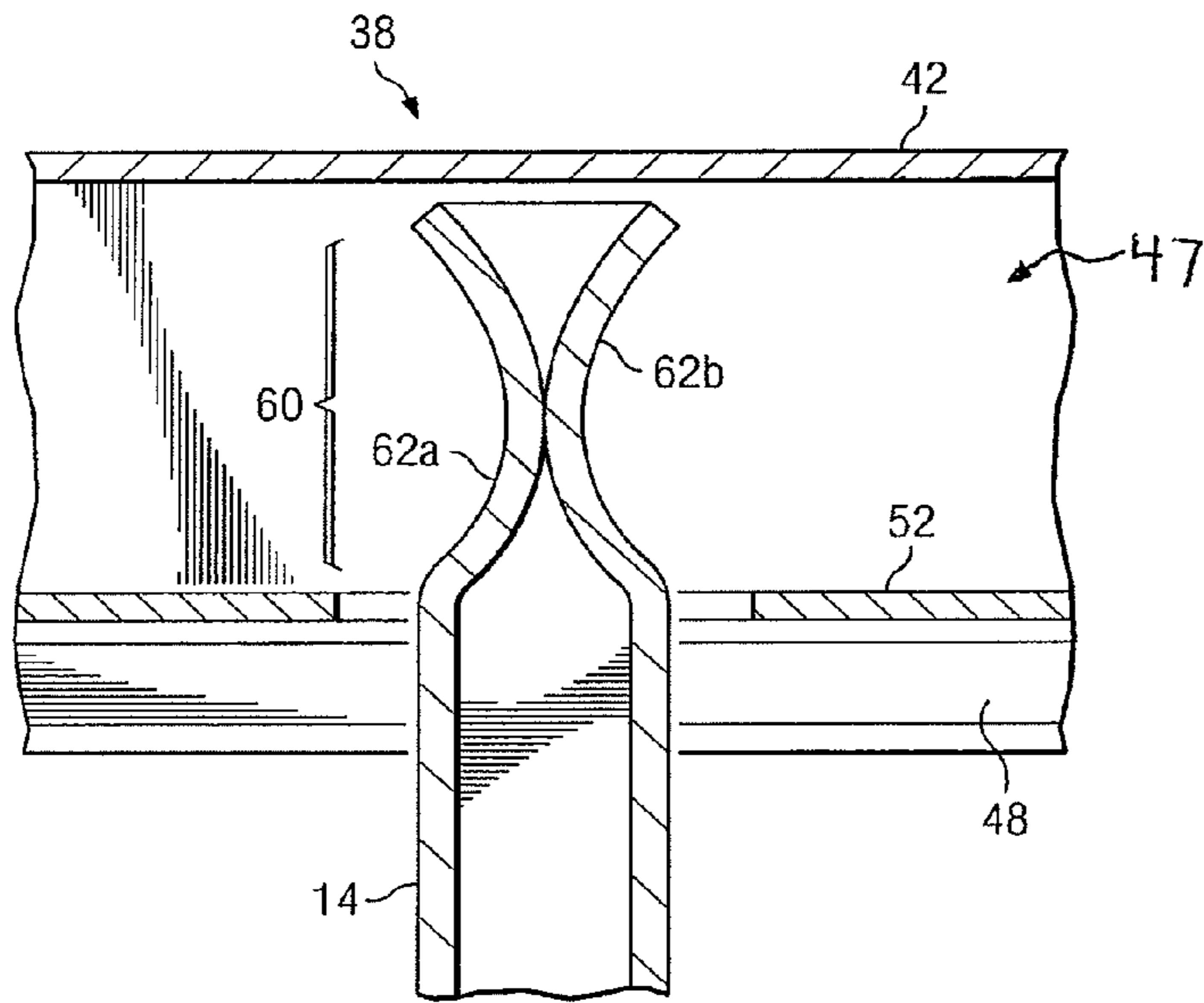
FIG. 5C
