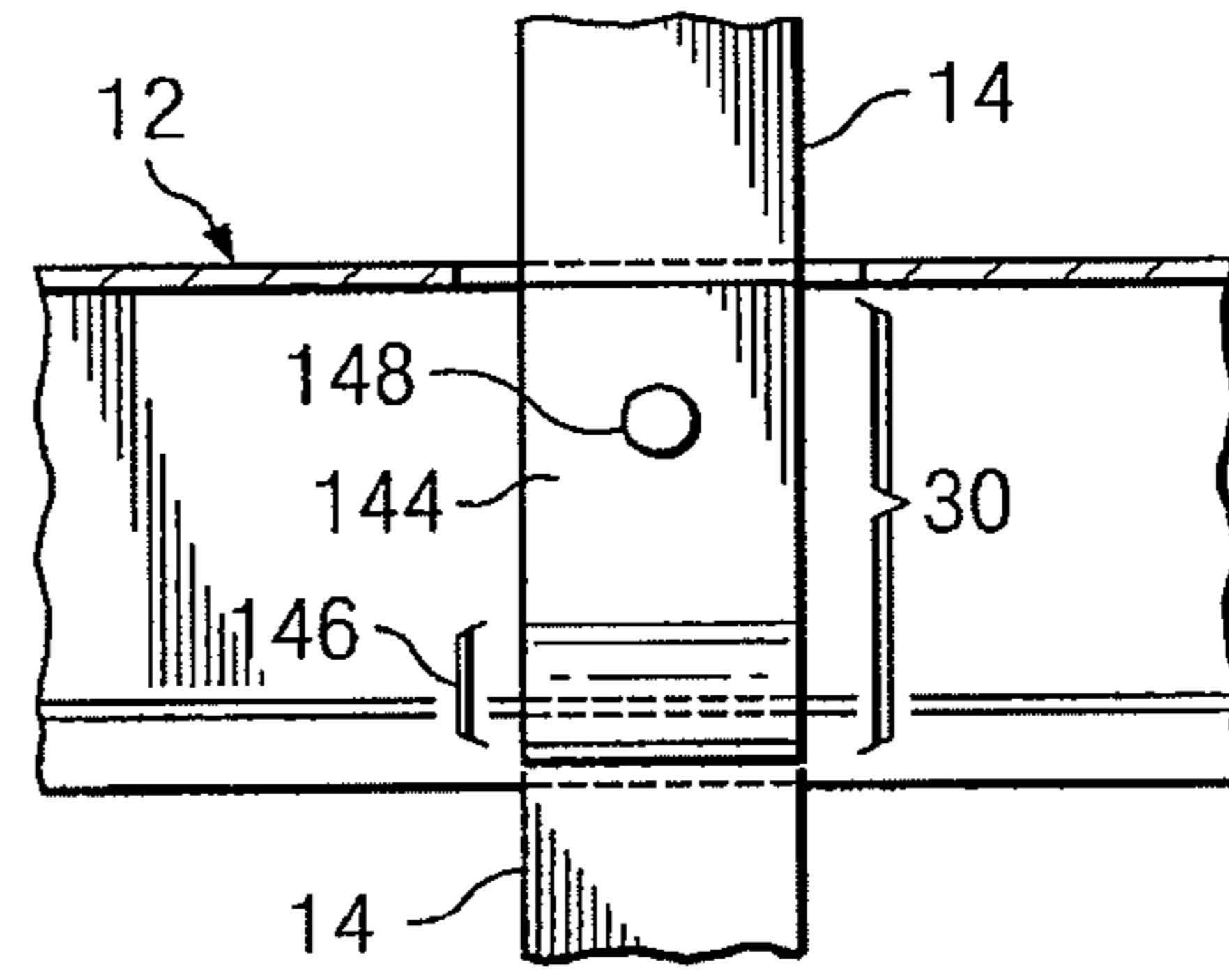
FIG. 14B
