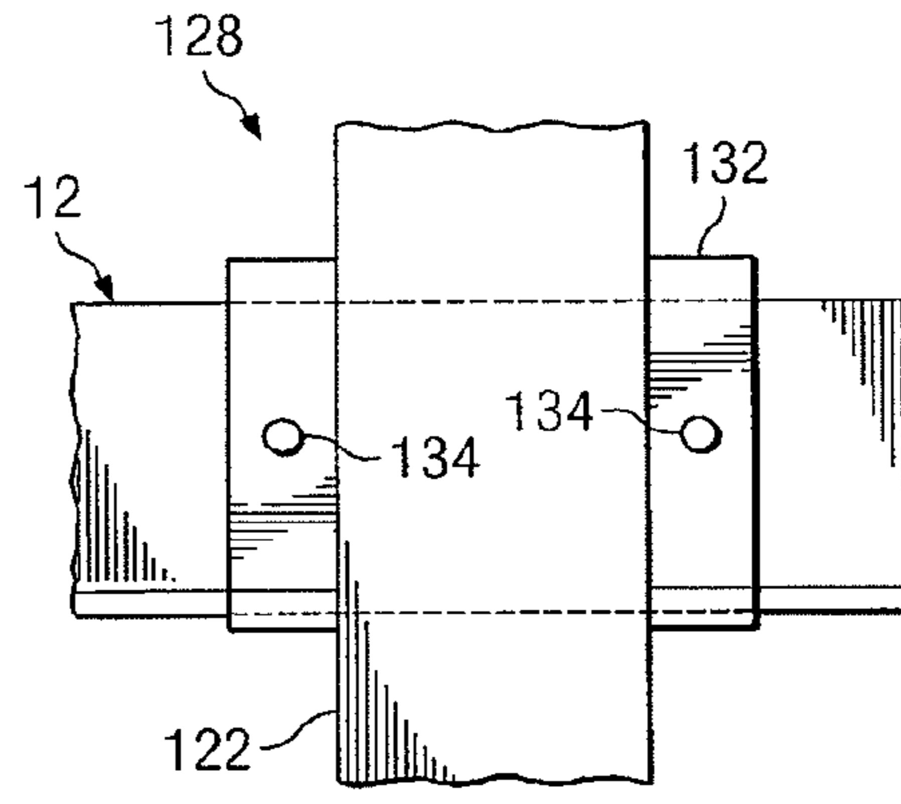
FIG. 11E
