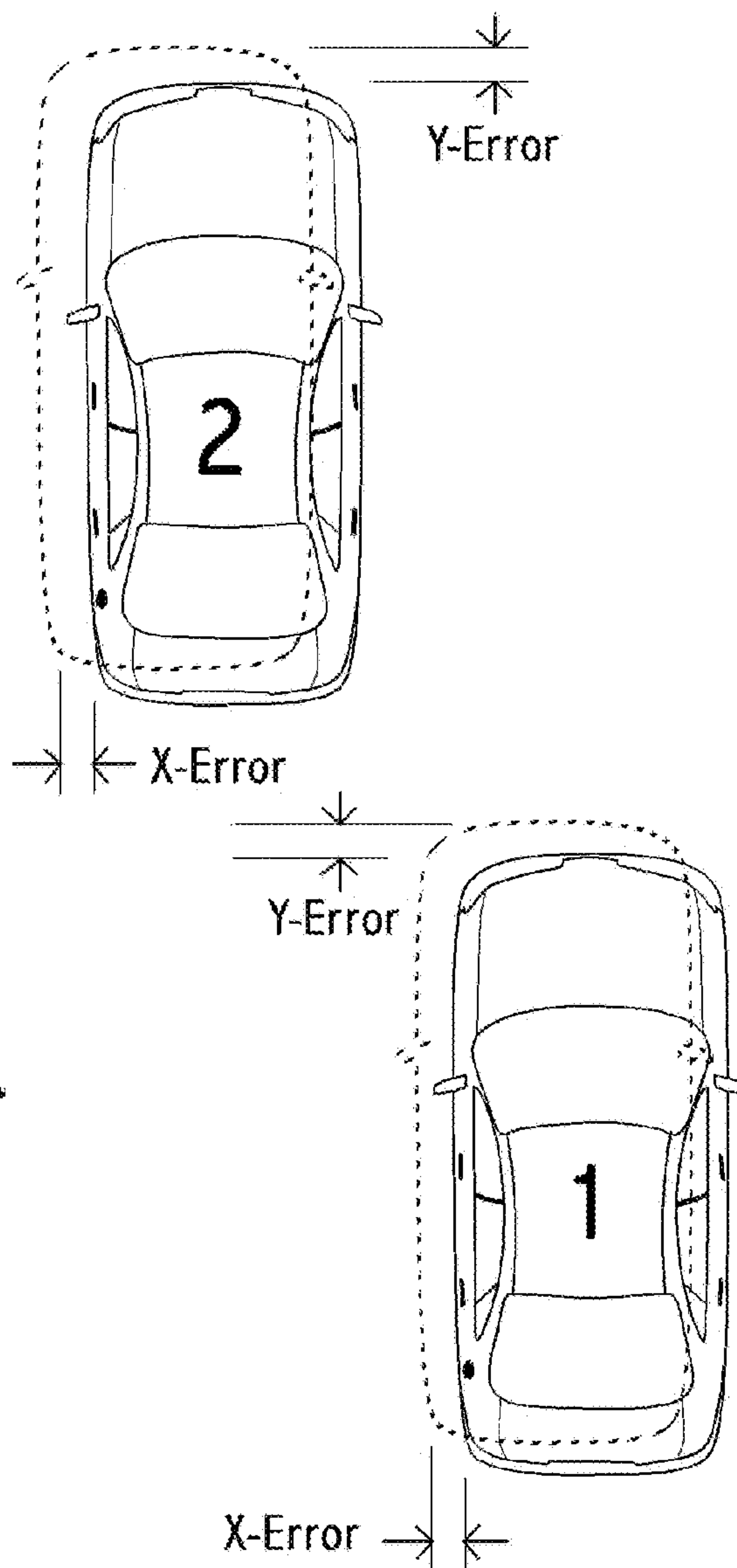
Fig. 11B
