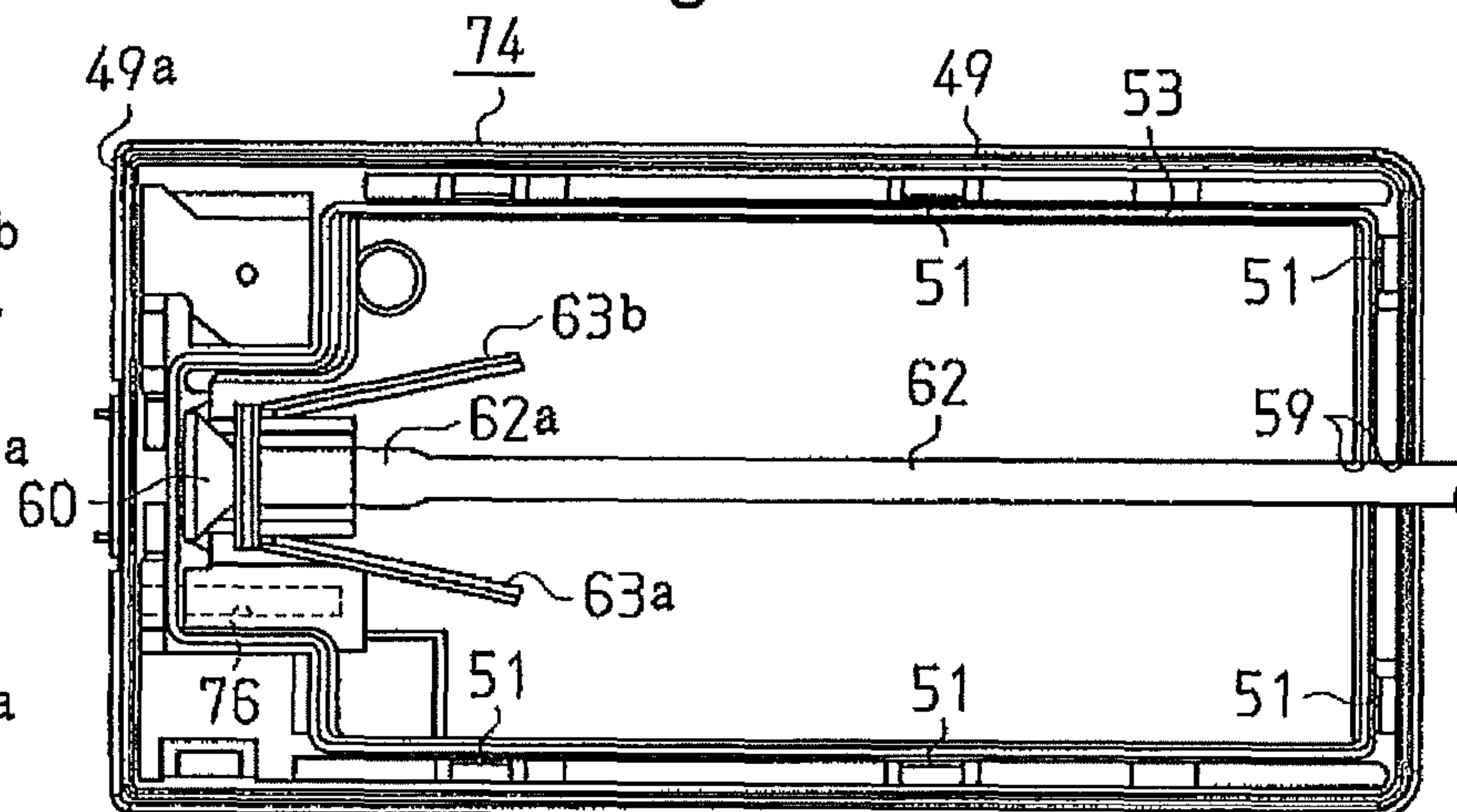
Fig. 7B
