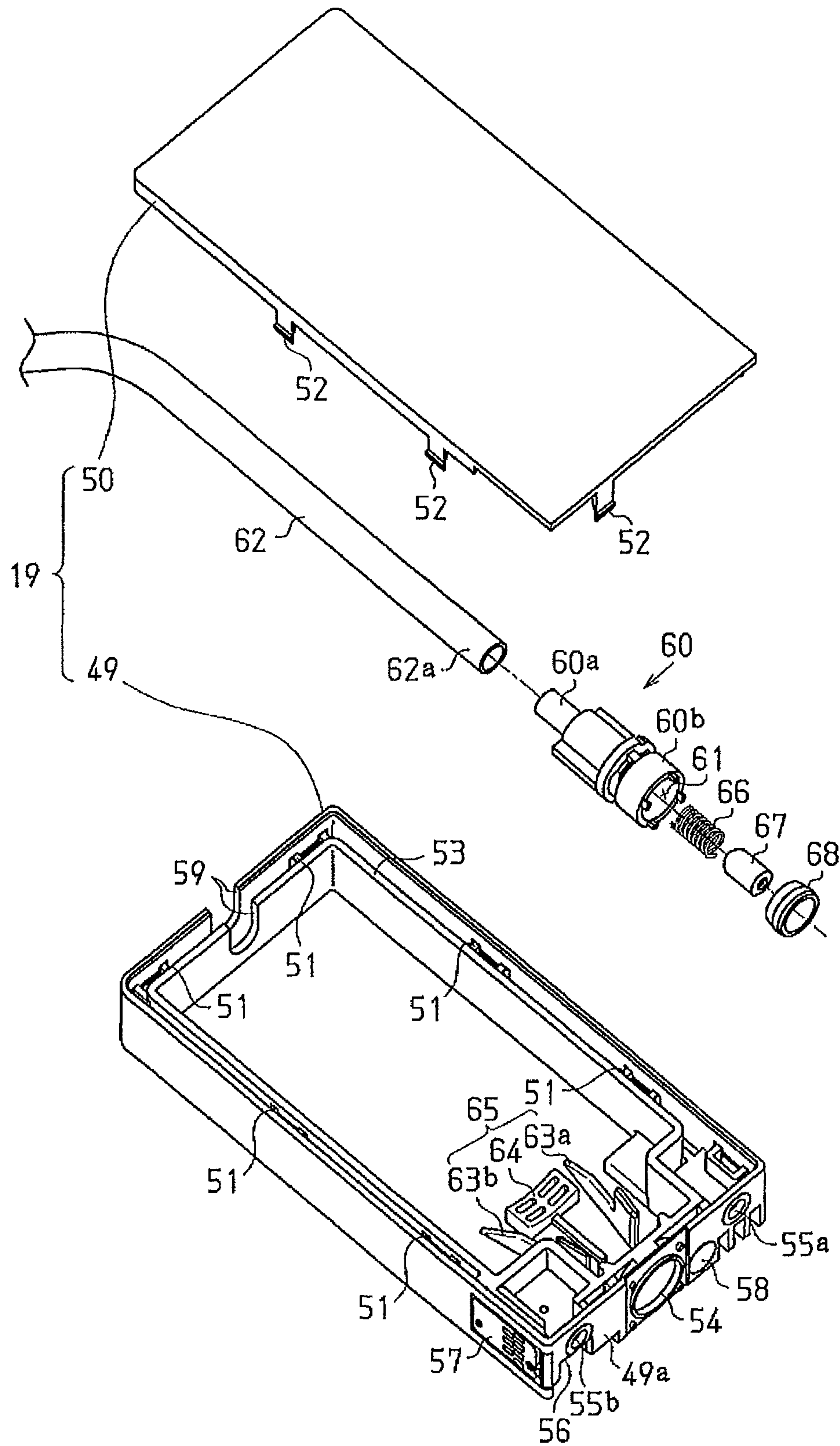
Fig. 5
