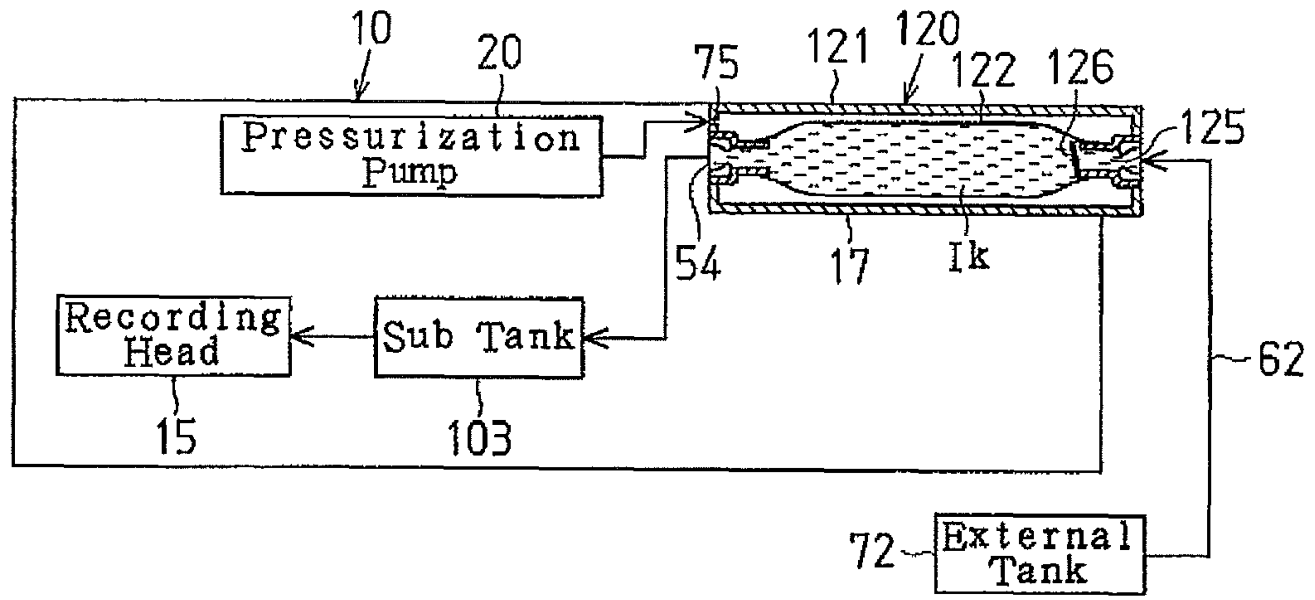
Fig. 16
