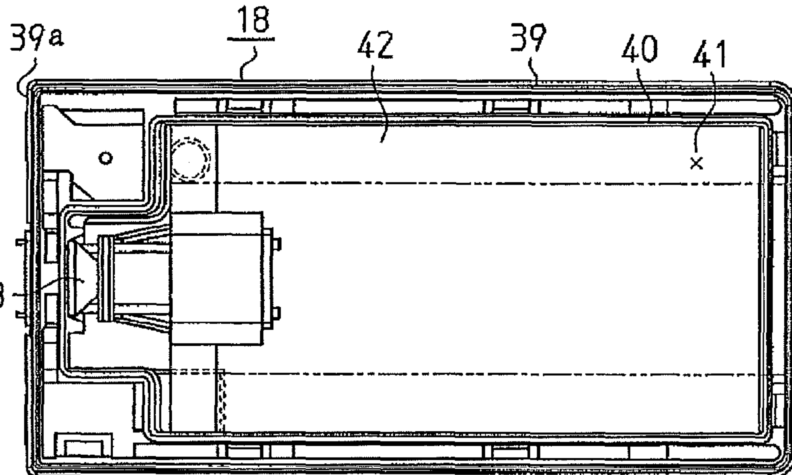
Fig. 4B
