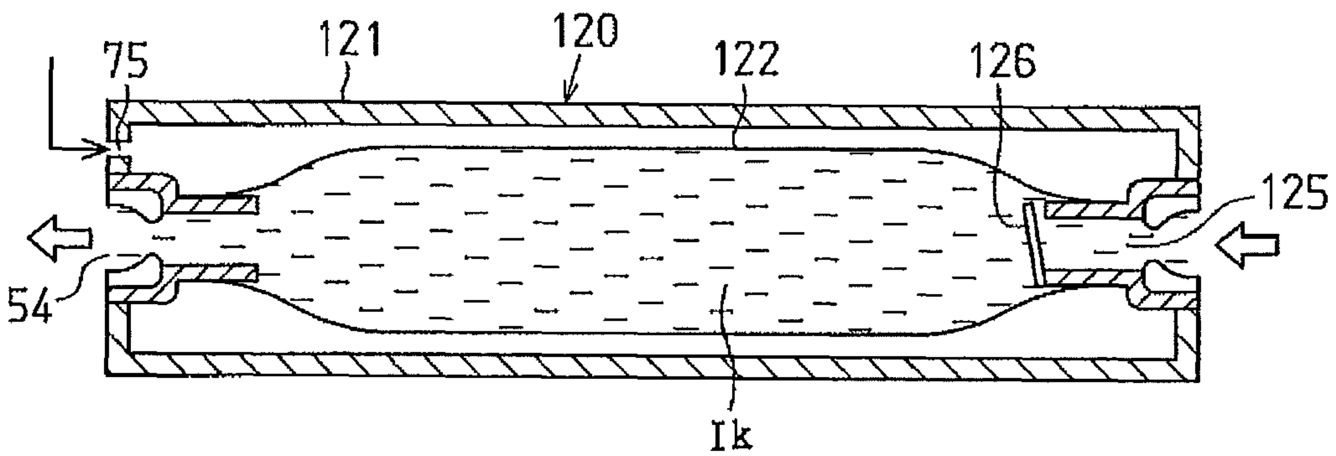
Fig. 17
