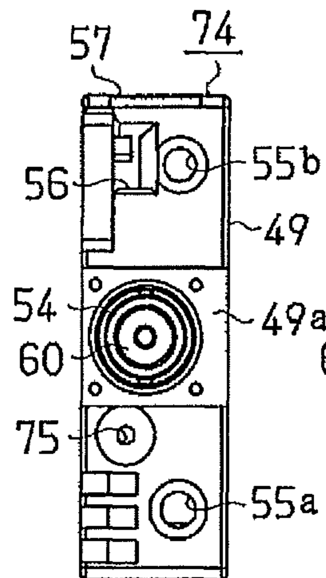
Fig. 7A
