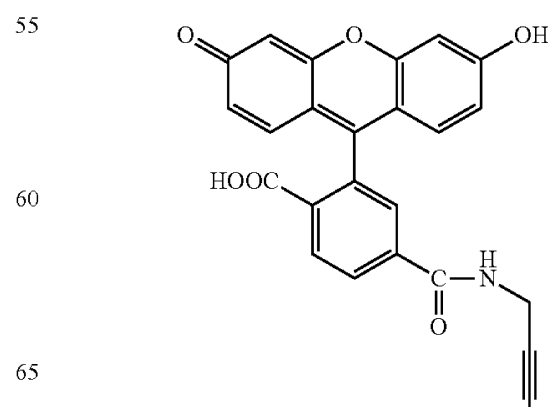
Scheme 27.
