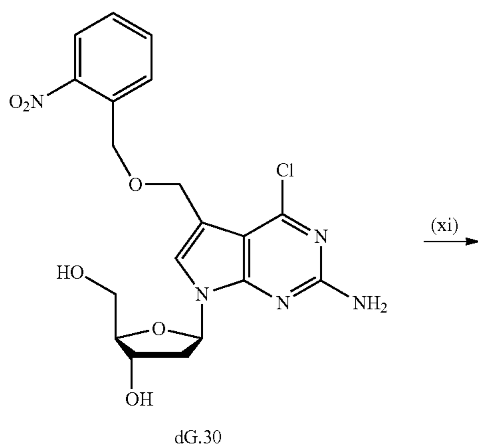
Scheme 20.
