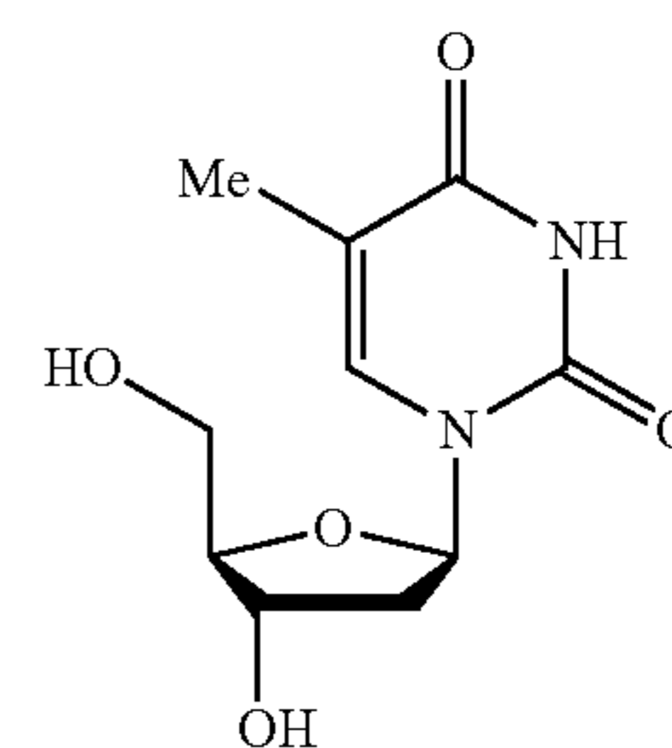
Thymidine
