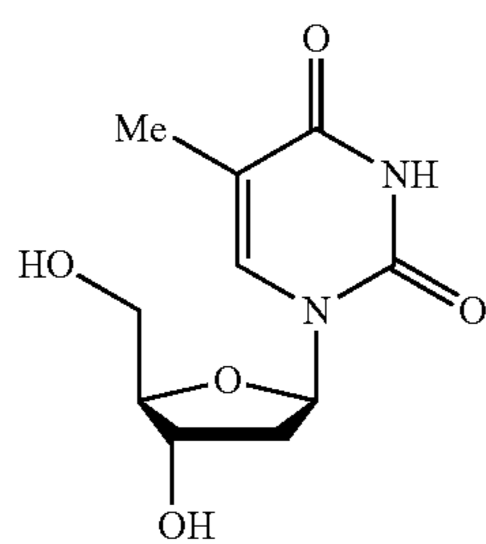
Thymidine
