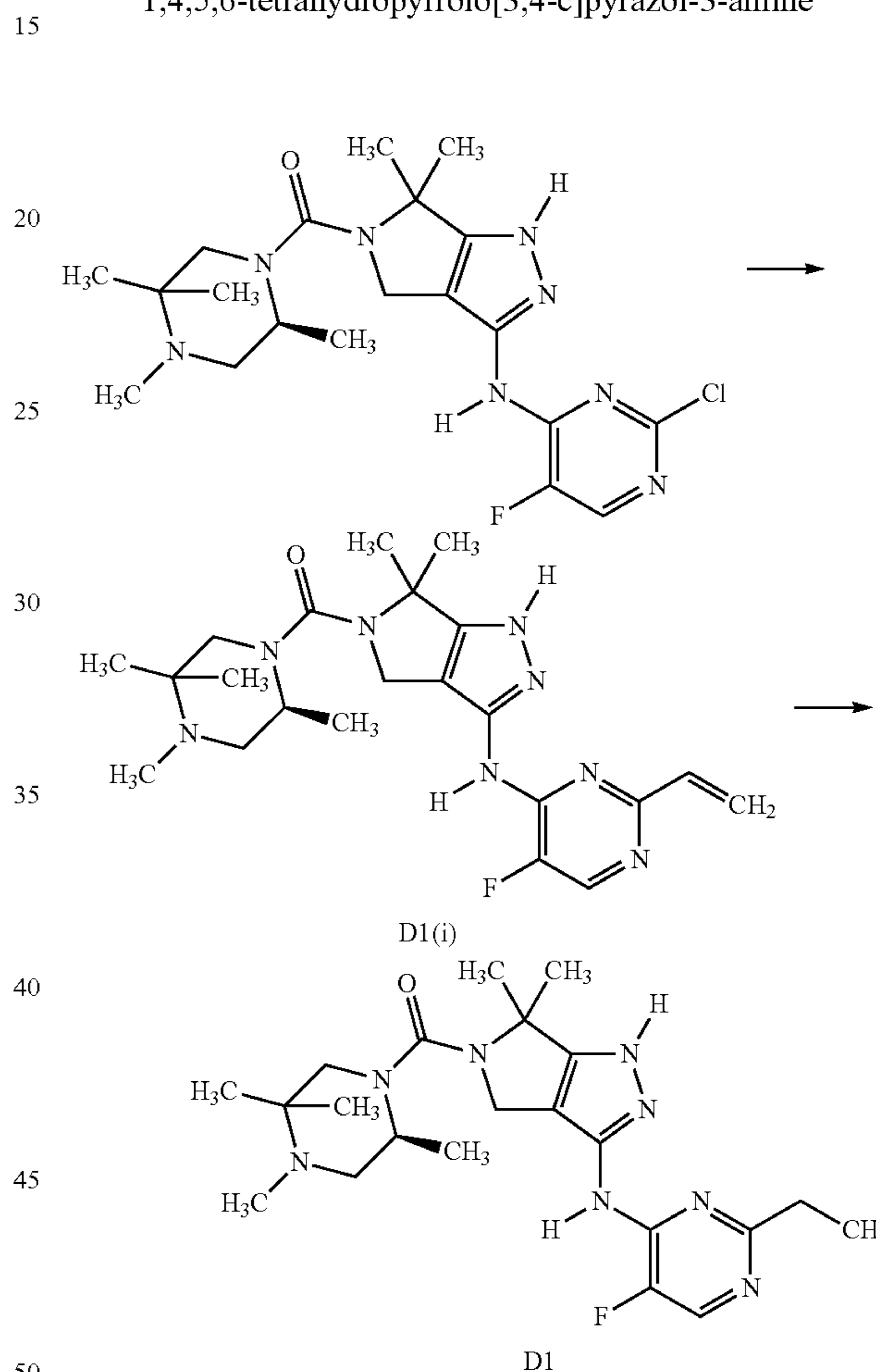
Intermediate D1(i)
