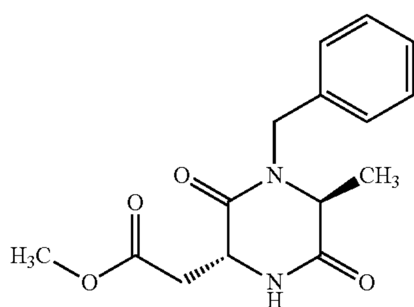
E5(v)
