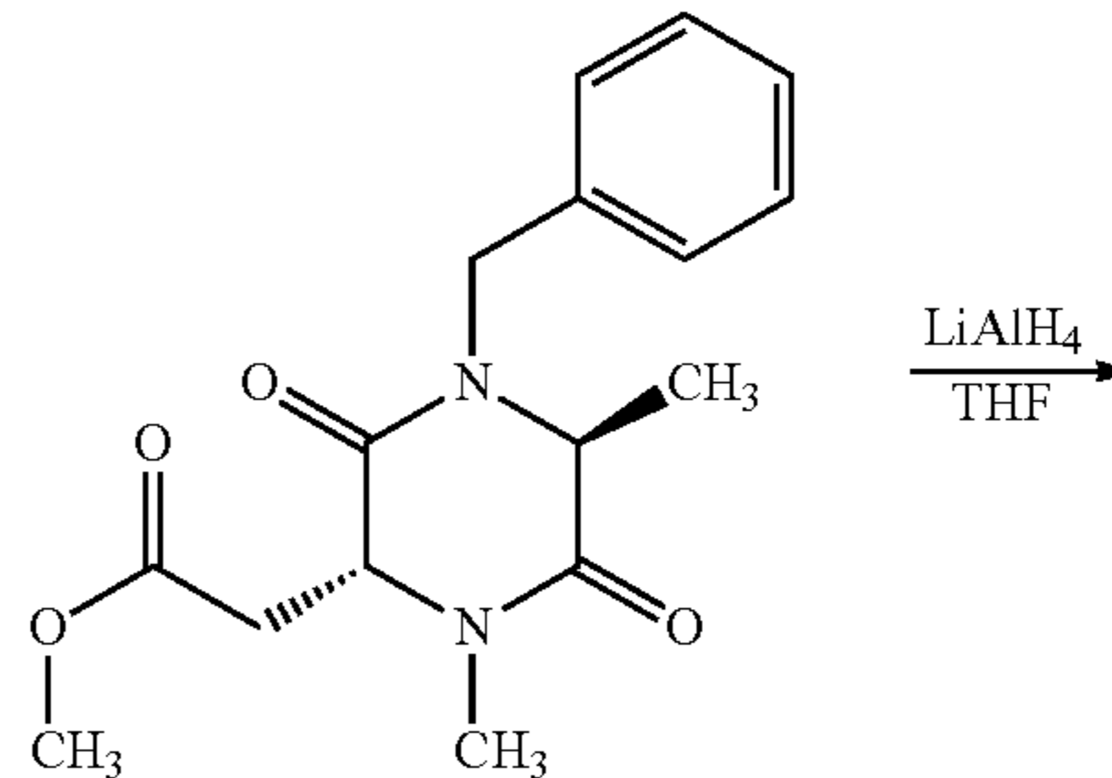
E5(viii)
