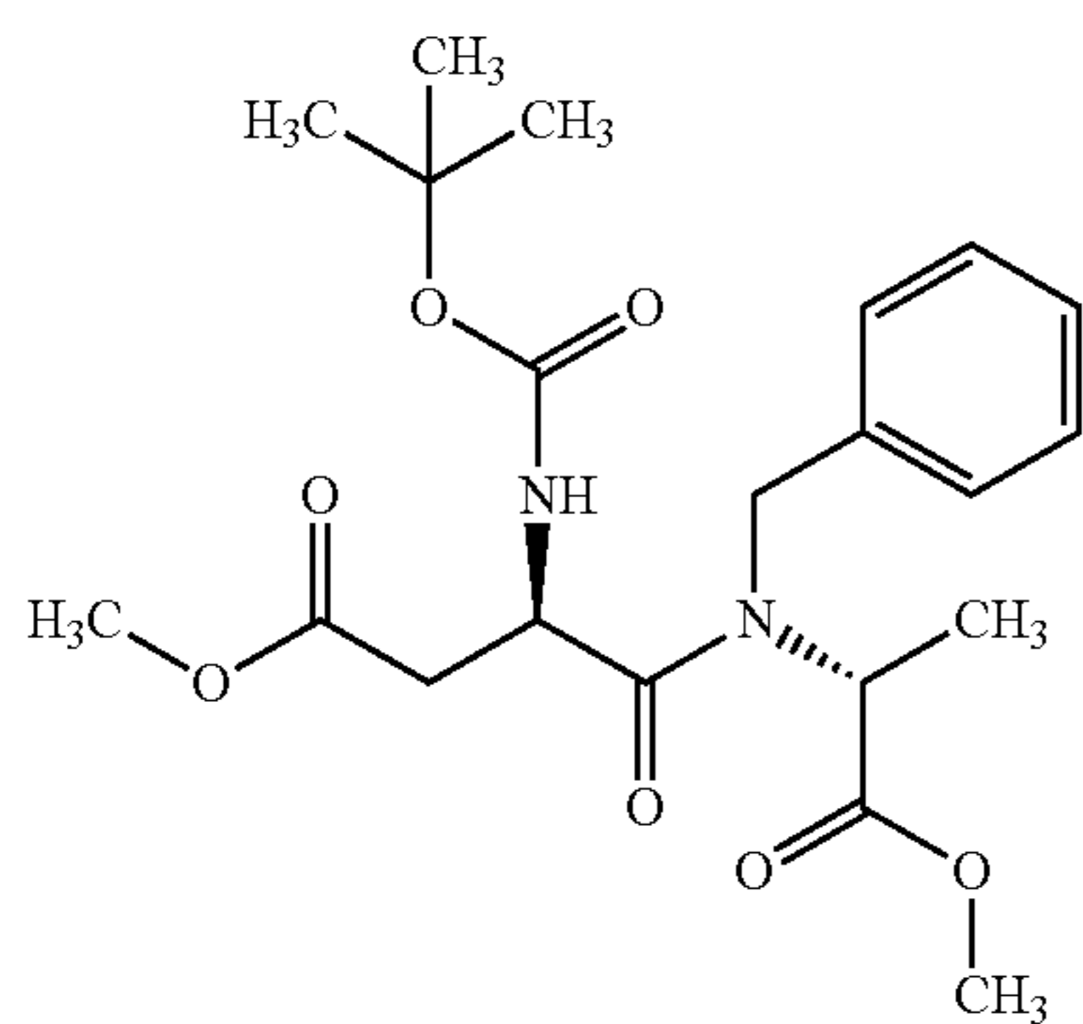
E5(v)
