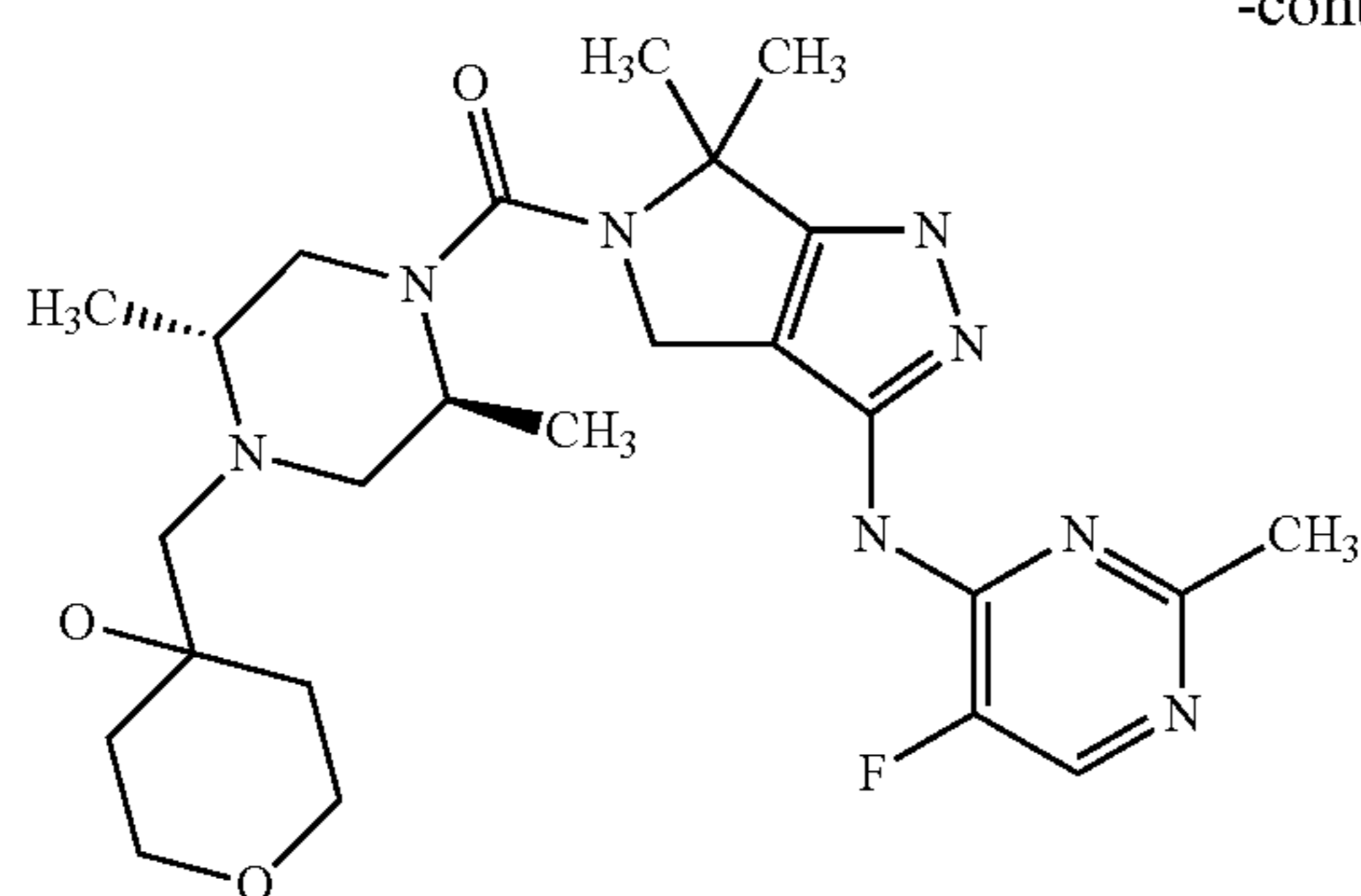
H8
