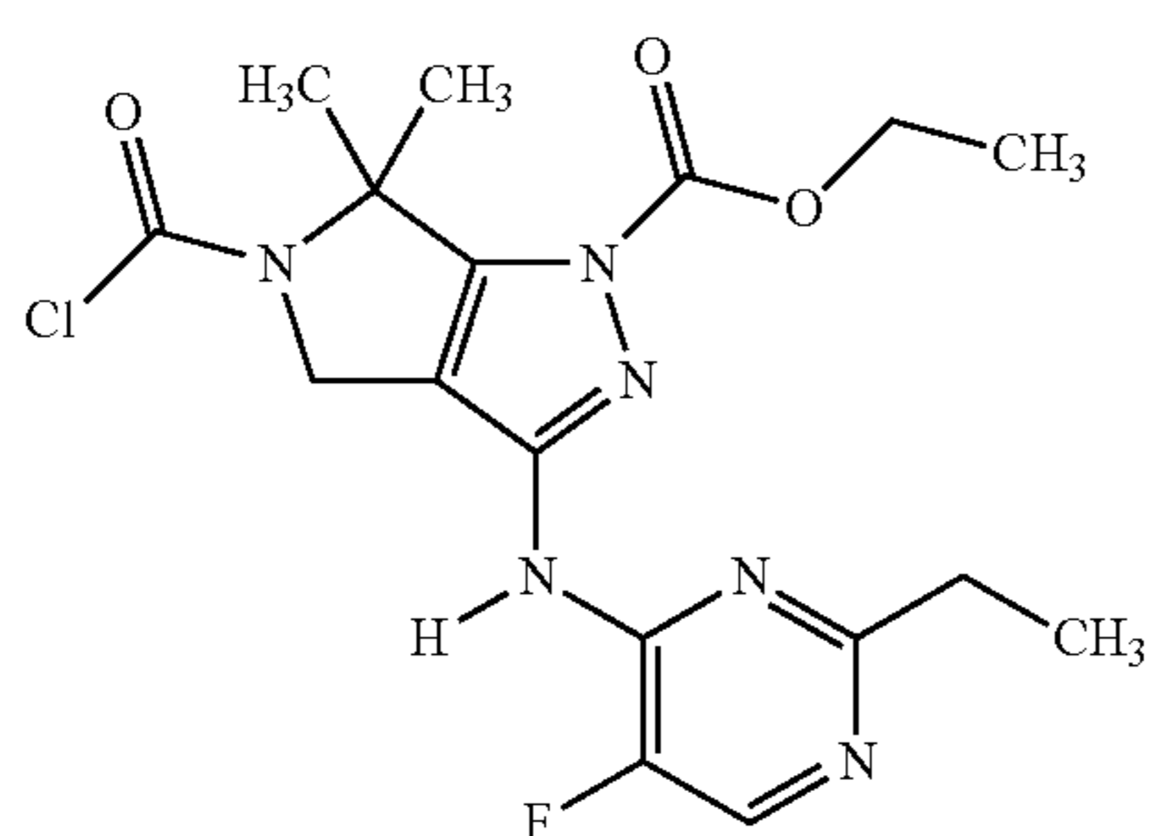
E1(iv)
