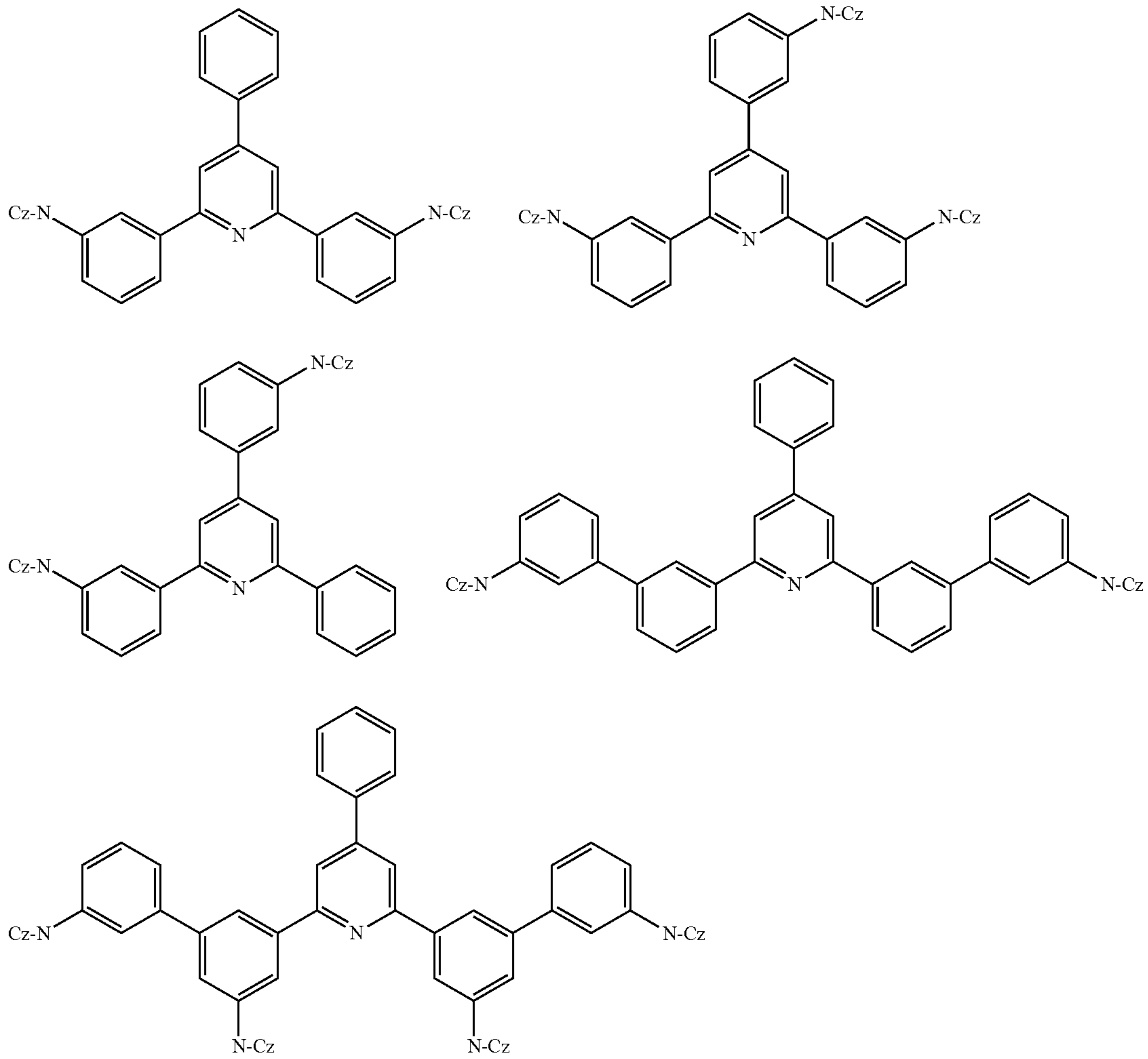
[Chem 9]
