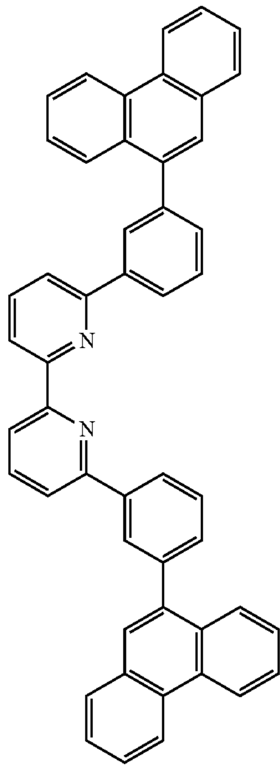
[Chem 9]
