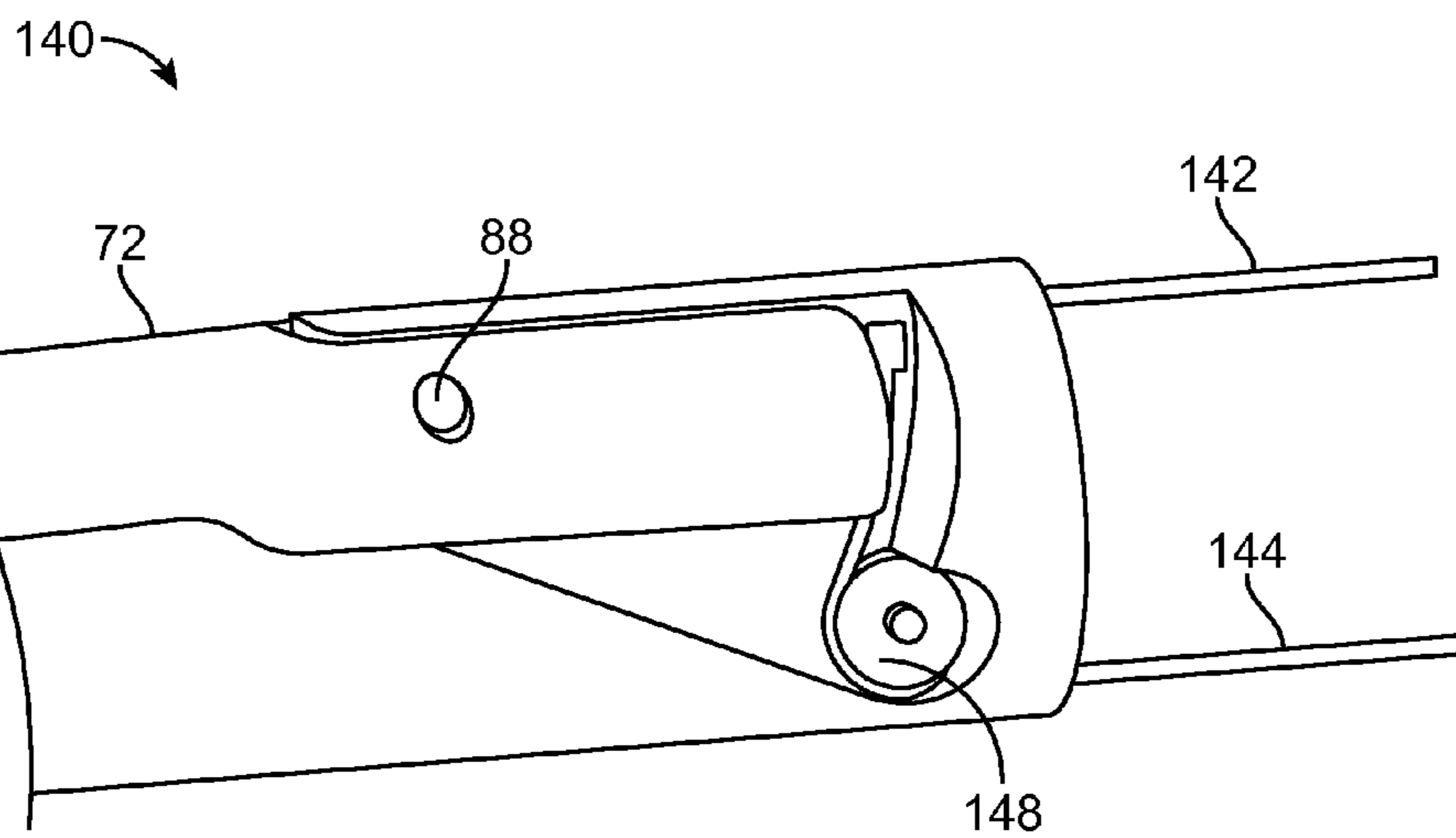
FIG. 9B
