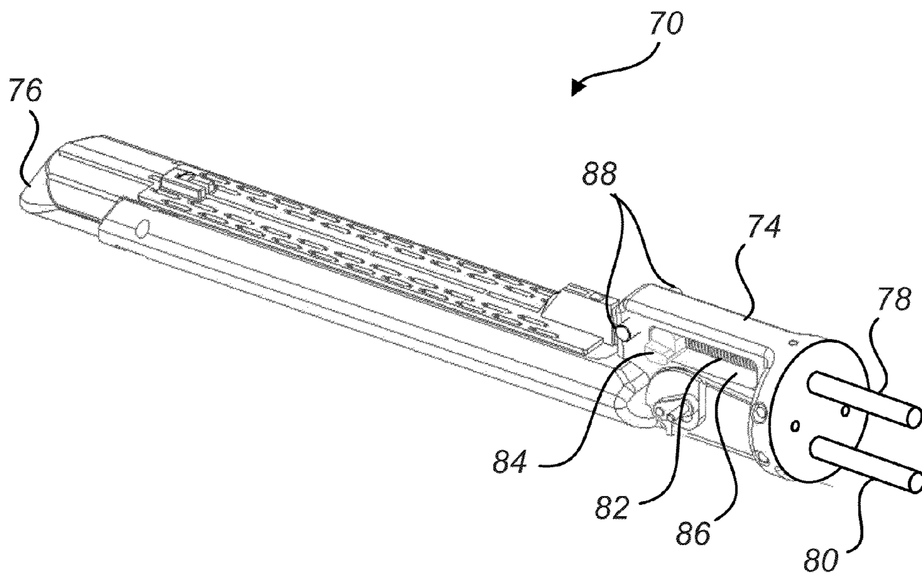
FIG. 6B
