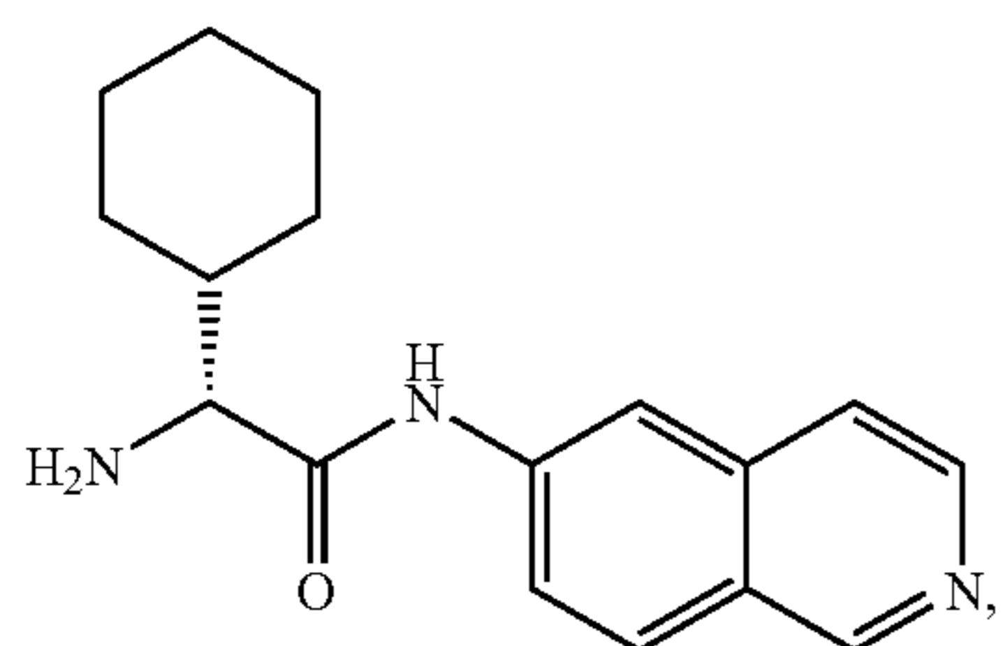
(R)-2-amino-2-cyclohexyl-N-(isoquinolin-6-yl)acetamide
