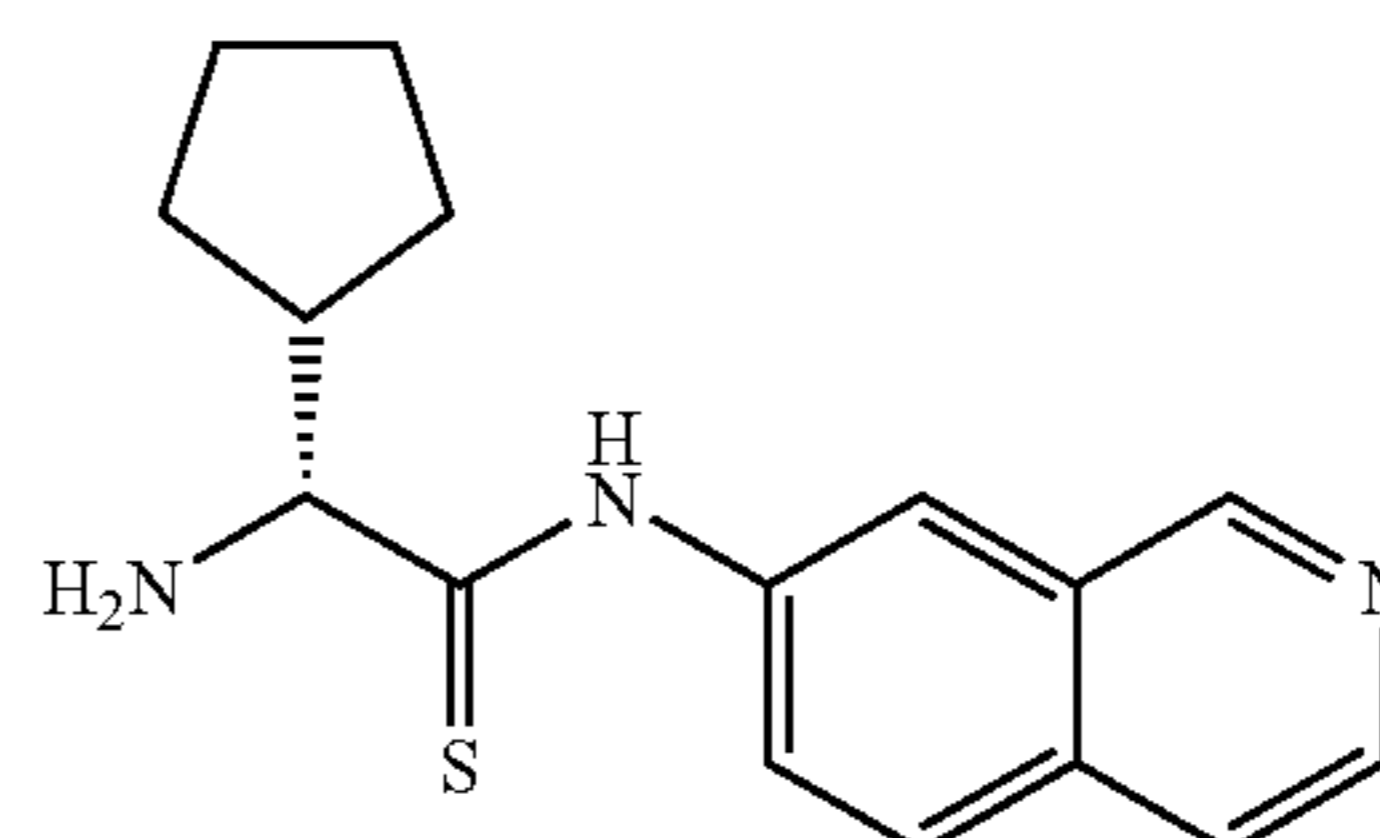
(R)-2-amino-2-cyclopentyl-N-(isoquinolin-7-yl)acetamide
