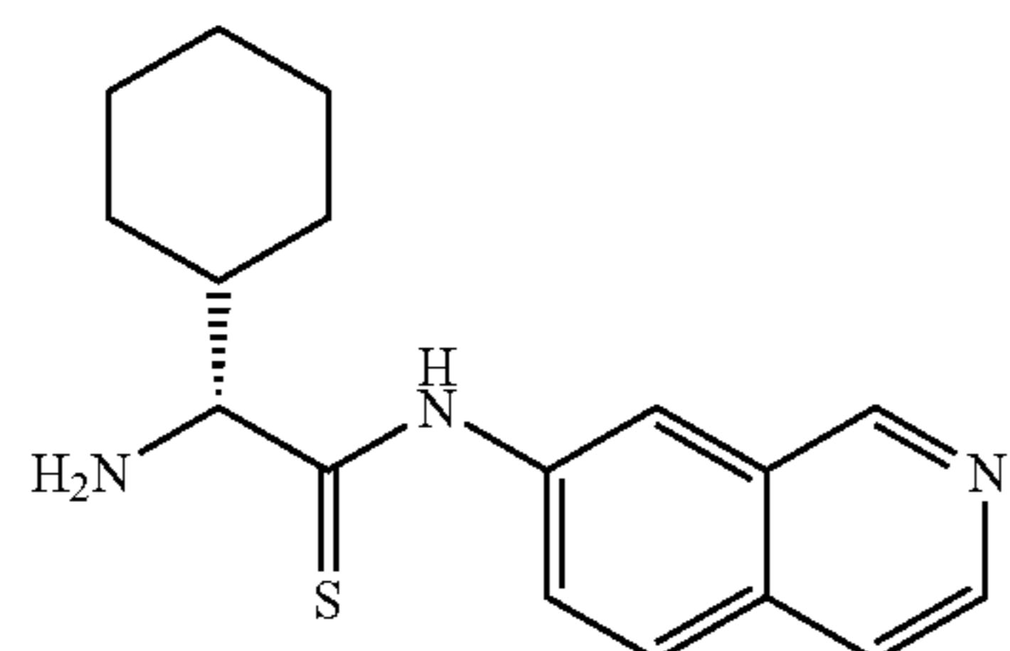
(R)-2-amino-2-cyclohexyl-N-(isoquinolin-7-yl)acetamide
