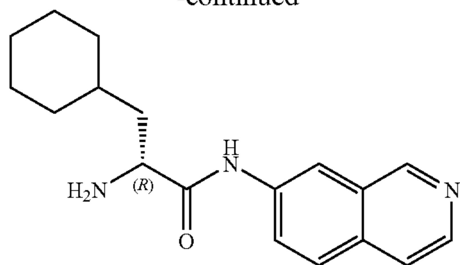
(R)-2-amino-3-cyclohexyl-N-(isoquinolin-7-yl)propanamide
