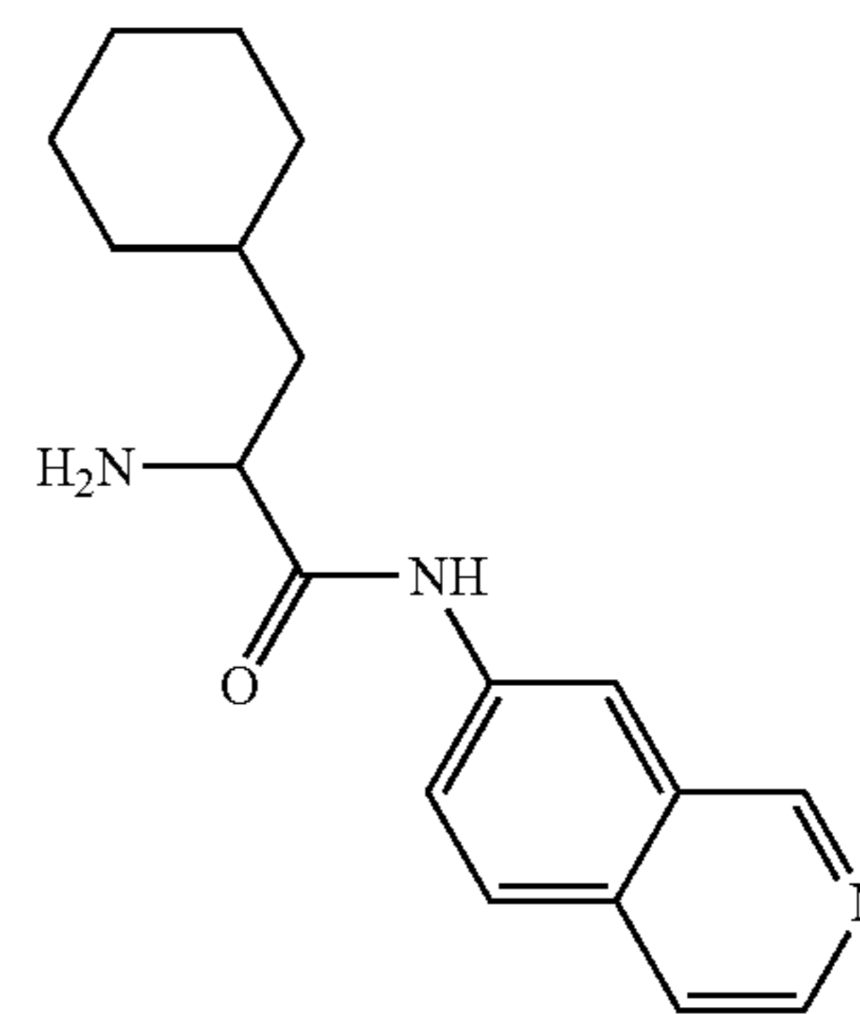
2-amino-3-cyclohexyl-N-(isoquinolin-7-yl)propanamide
