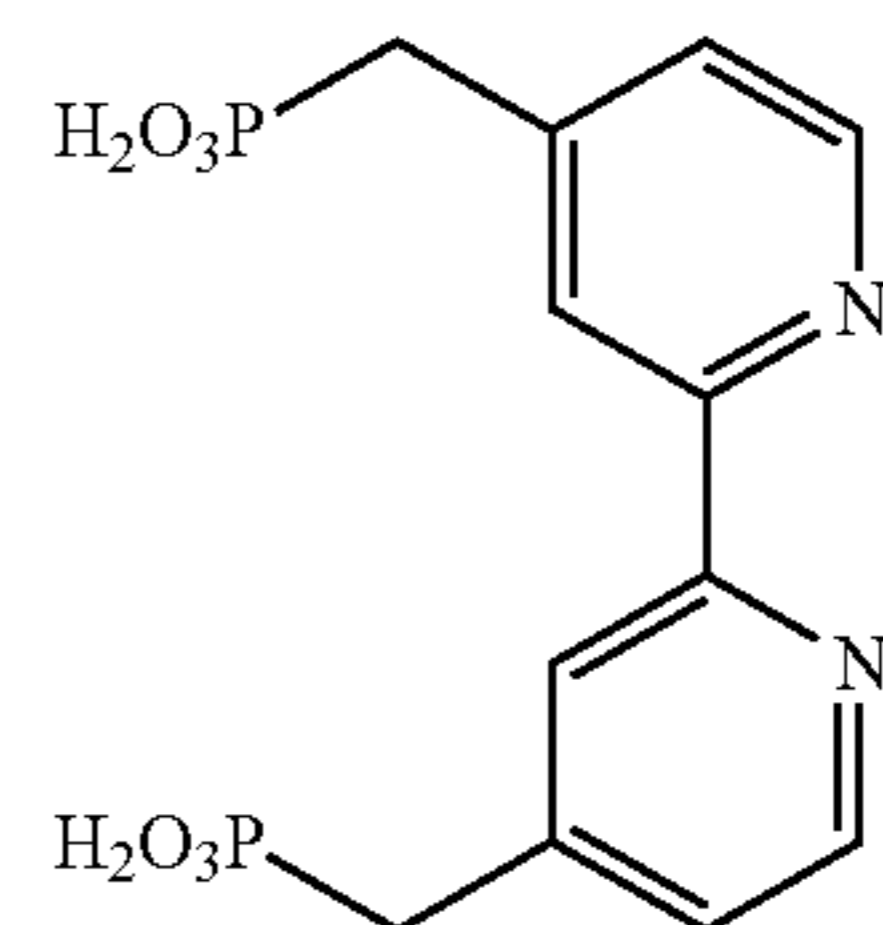
P 2 -bpy
