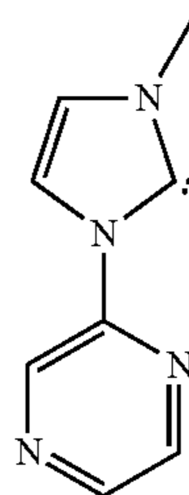
Melm-pz
